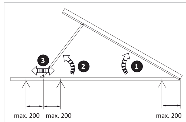
Afb. 29: Opbouw van de collectorsteunen voor platte daken
