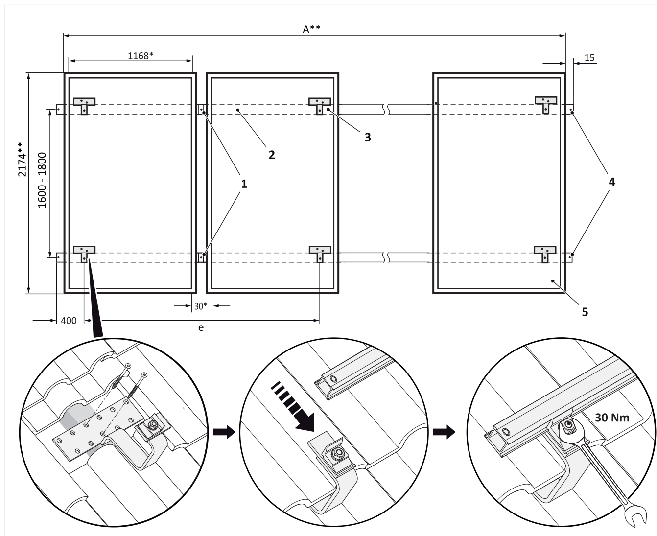
Afb. 18: Montage van de dakbeugels en de montagerails naast elkaar.
