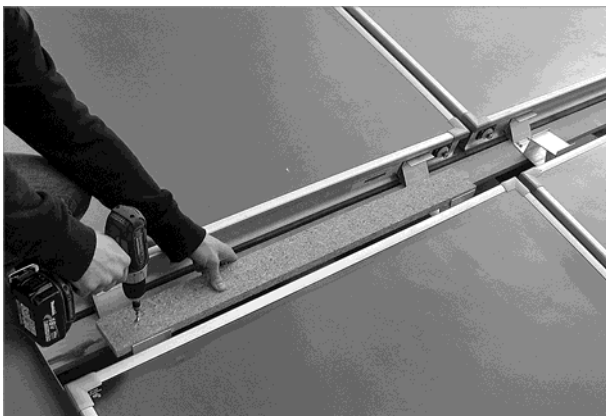
Afb. 67: De tussenplaatsteunen op de collector-afstandsstukken schroeven
