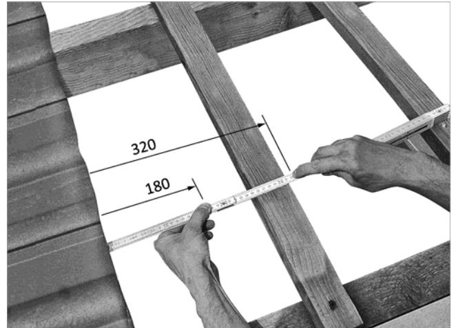
Afb. 44: De positie van de onderste daklat controleren
