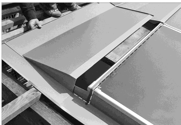
Afb. 79: De bovenplaat op de zijplaat plaatsen en tegen de collector schuiven.
