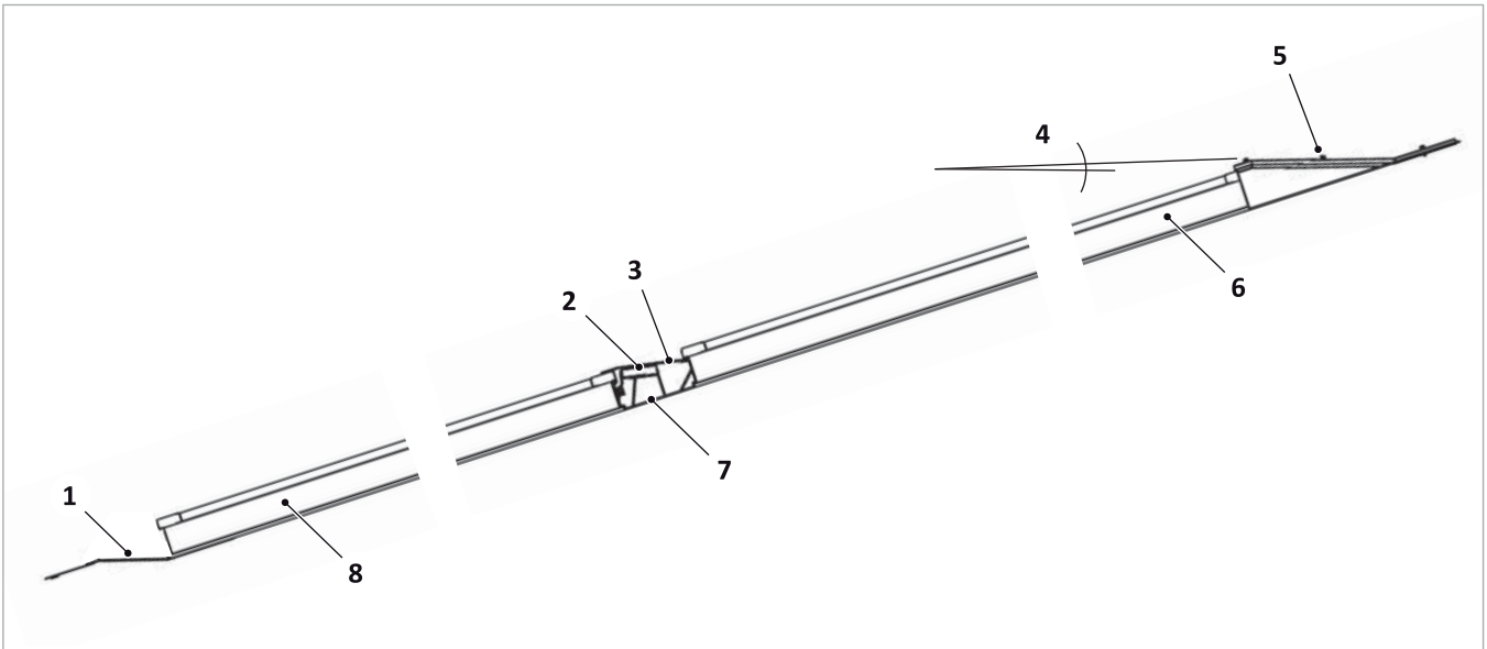
Afb. 41: Doorsnede van een collectorveld met twee rijen
