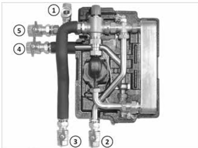
Abb. 4: Warmwasserstation eingehängt
