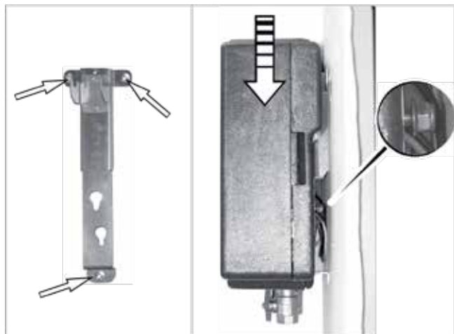
Abb. 3: Halteschiene montieren, Station einhängen und fixieren
