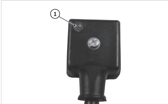
Abb. 11: Magnetventil-Stecker
