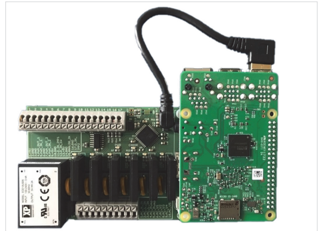
Abb. 9: Relaisplatine V 4.2 mit Steuerungs-PC
