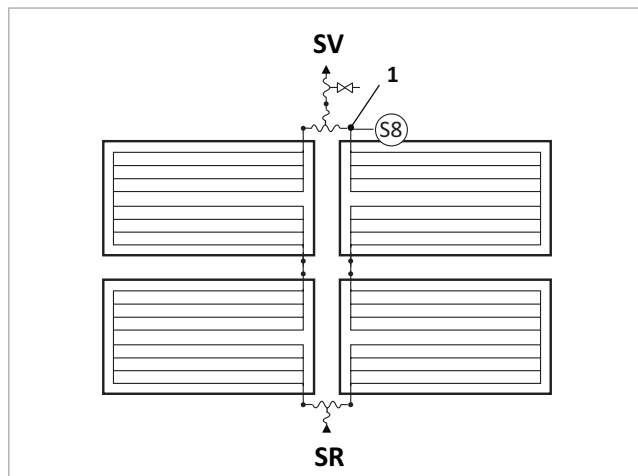
Abb. 2: Parallelschaltung / Parallel connection / Collegamento in parallelo / conexión en paralelo / Conexão paralela / Connexion parallèle / Parallel-aansluiting
