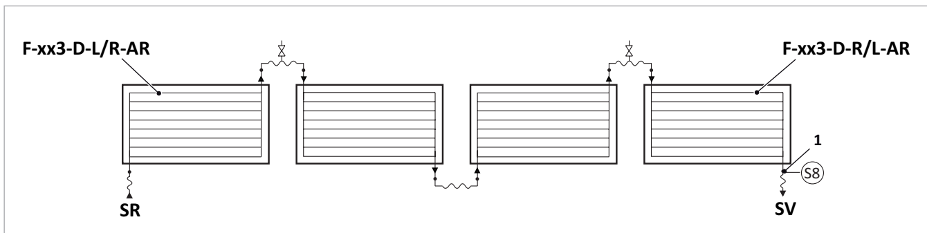
Abb. 3: Reihenschaltung / Series connection / Collegamento in serie / Conexión en serie / Conexão em série / Connexion série / Series-aansluiting
