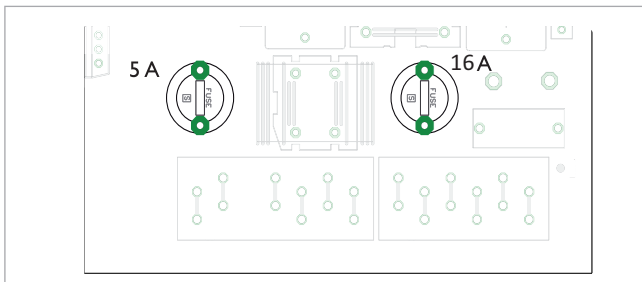
Abb. 41: Sicherungen der Leistungselektronik
