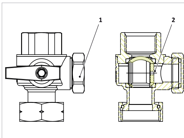
Abb. 40: Seitliche Kappe abnehmen
