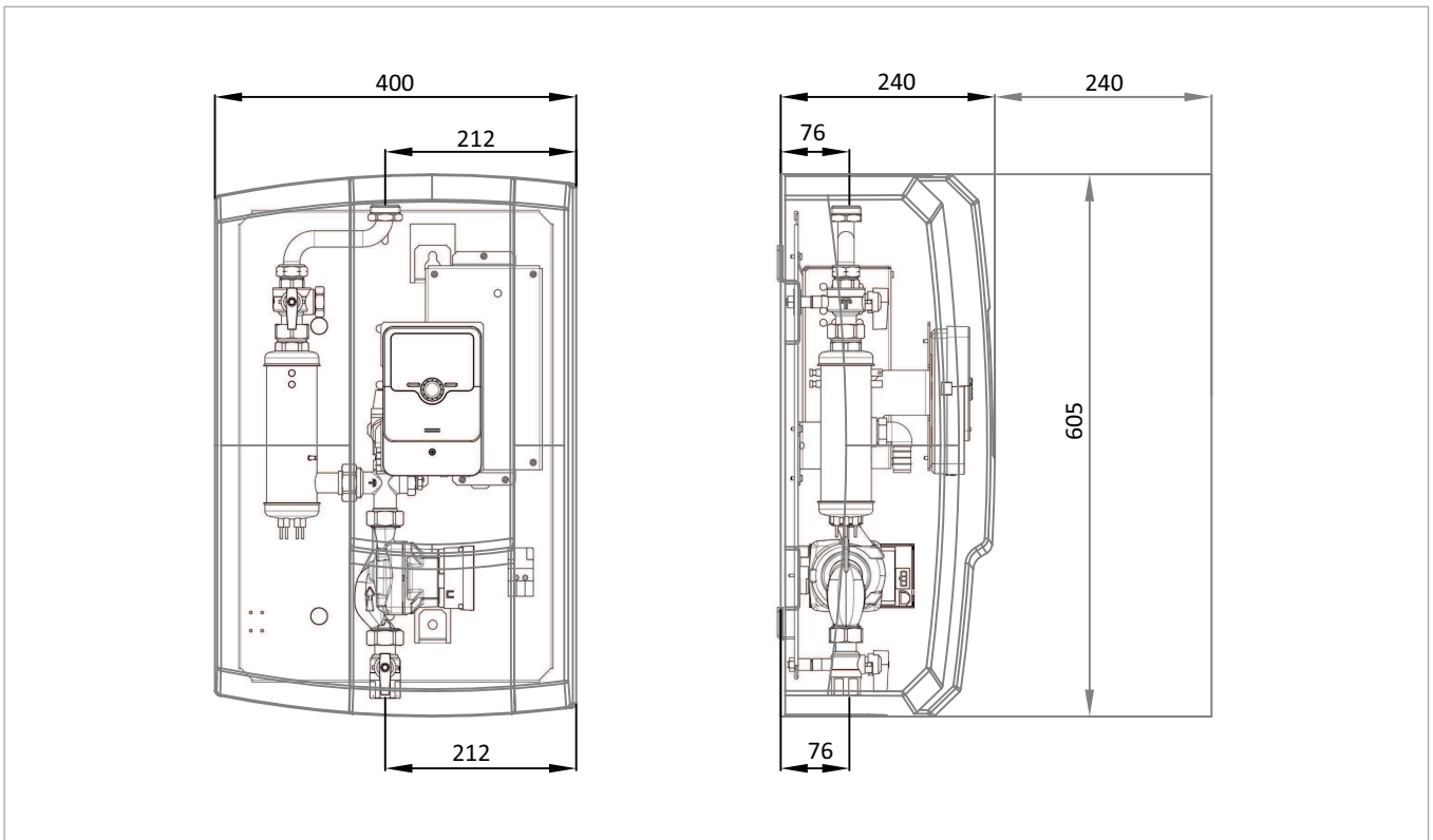
Abb. 43: Abmessungen und Mindest-Platzbedarf für Montage und Wartungsarbeiten
