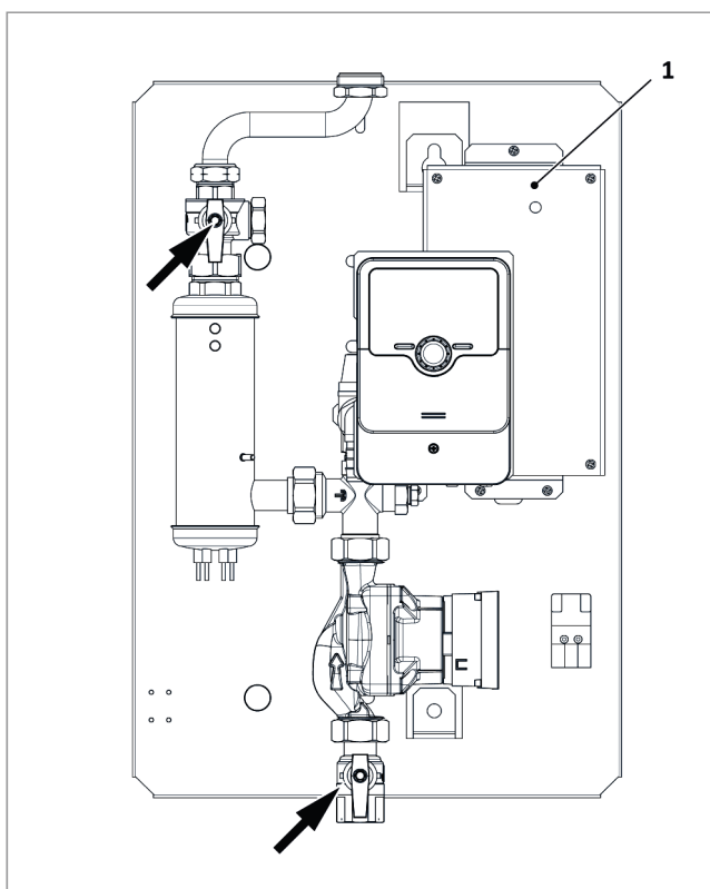
Abb. 39: Kugelhähne absperren
