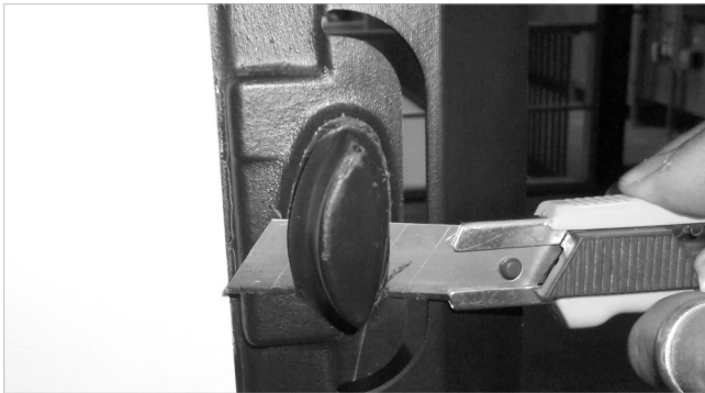
Abb. 2: Knopf abschneiden
