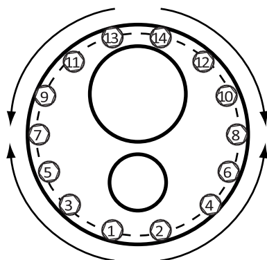
Fig. 4: Secuencia de apriete de los tornillos
