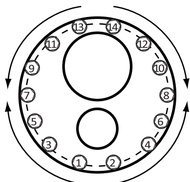
Fig. 5 : ordre de serrage des vis
