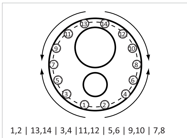
Abb. 1: Anzugsreihenfolge der Schrauben
