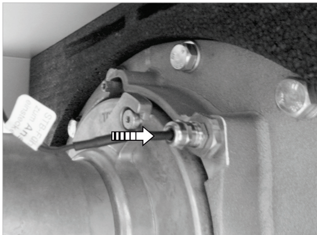
Abb. 71: mSTB einstecken
