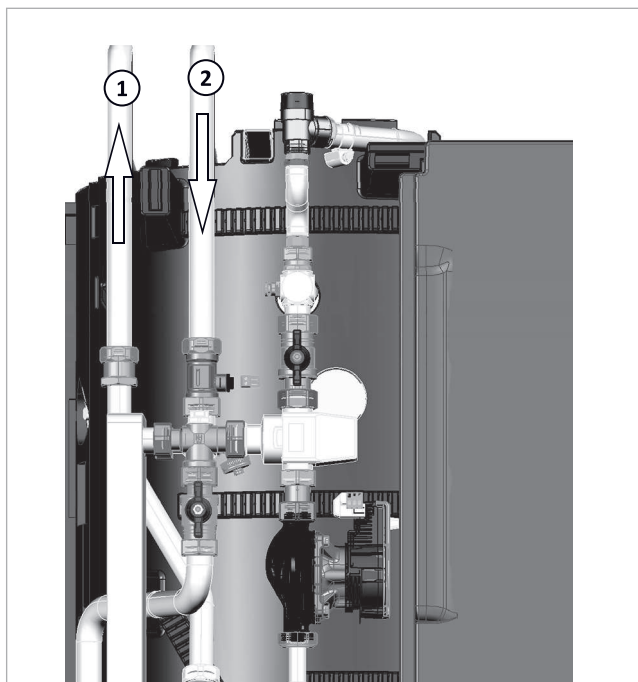
Abb. 28: TWW-/TWK-Anschluss von oben
