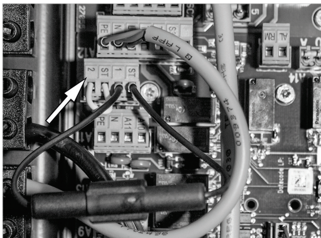
Abb. 57: Buchsenleiste aufstecken
