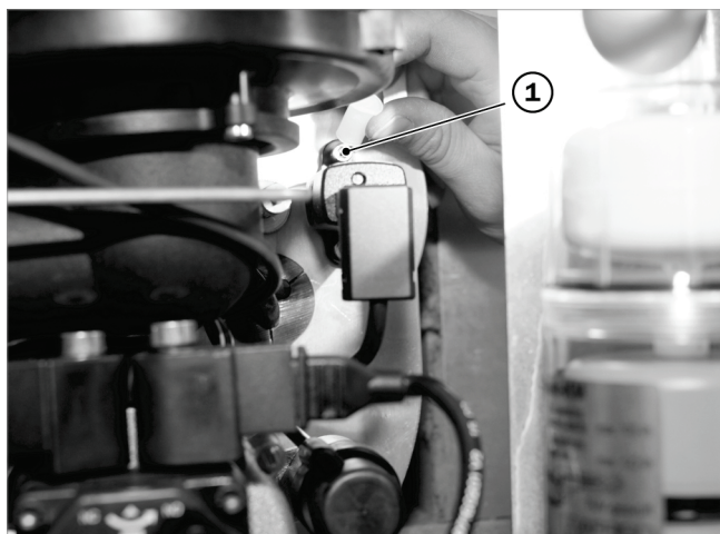
Abb. 119: Gebläsedruck messen
