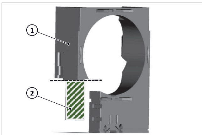
Abb. 10: Flanschisolierung beschneiden
