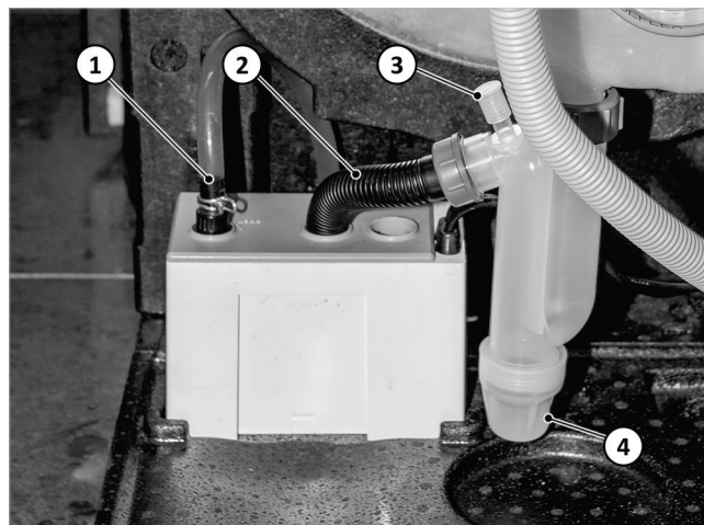
Abb. 91: Kondensatpumpe, angeschlossen
