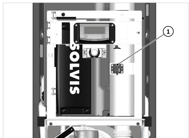
Abb. 78: Ölfilter-Halterung befestigen
