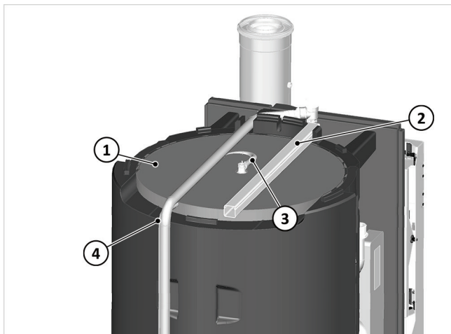
Abb. 18: Deckelrunde und Leitungskanäle auflegen
