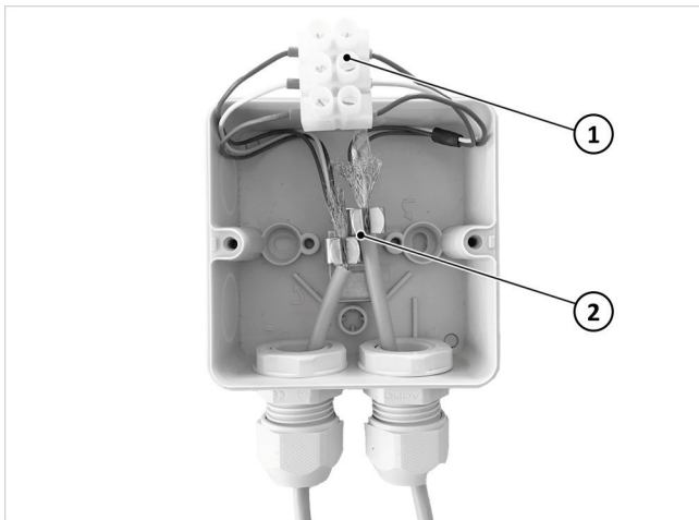
Abb. 110: Modbus-Verbindungsdose befestigen
