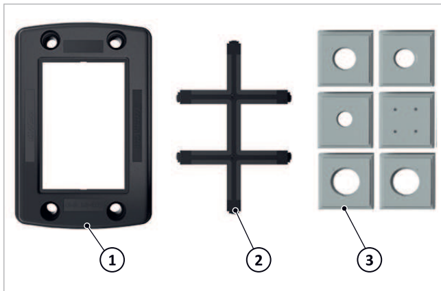
Abb. 75: Leitungsdurchführungssystem mit Ölleitung
