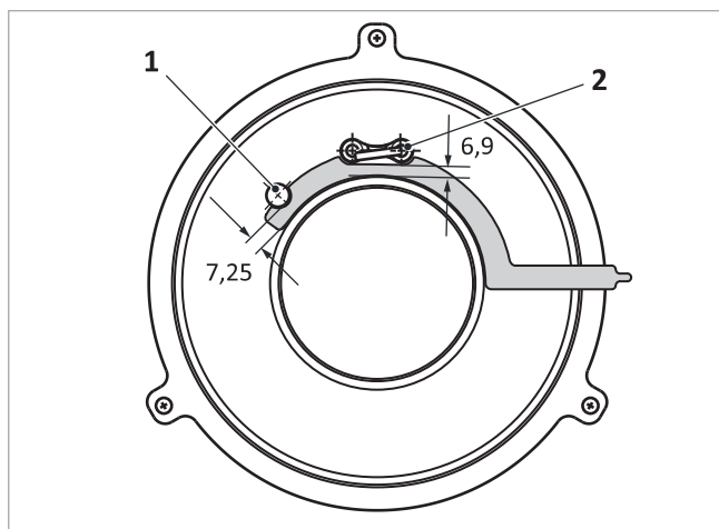
Abb. 142: Abstände Ionisations- und Zündelektrode zum Brennnervlies
