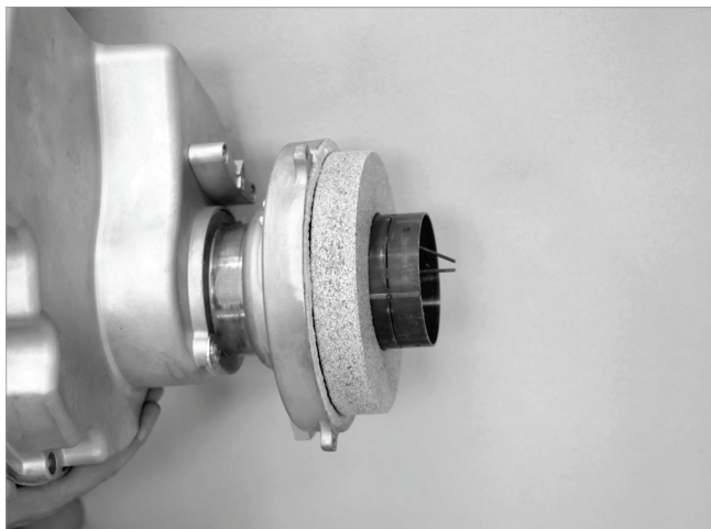
Abb. 68: Kesseltürstein aufsetzen
