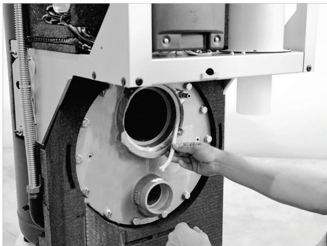
Abb. 46: Brennerdichtschnur einlegen
