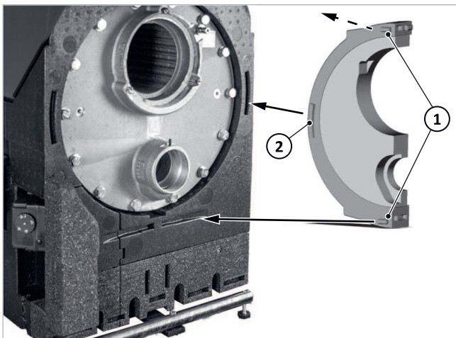
Abb. 99: Vordere Flanschisolierung (rechts, Rückansicht) mit Rastfedern
