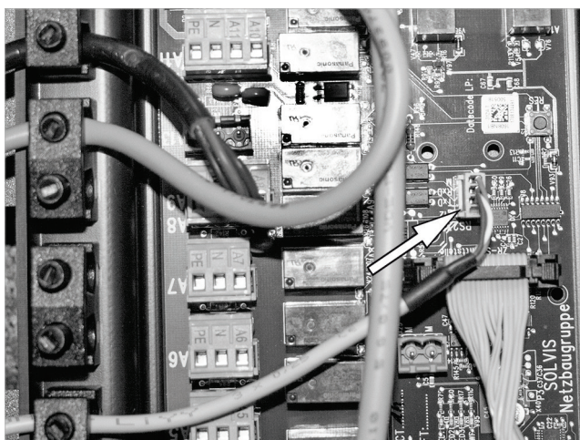
Abb. 56: Bus-Stecker anschließen
