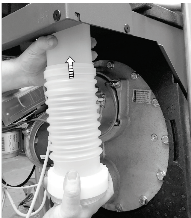
Abb.88: Abgasanschlusstück auf Abgasrohr stecken.
