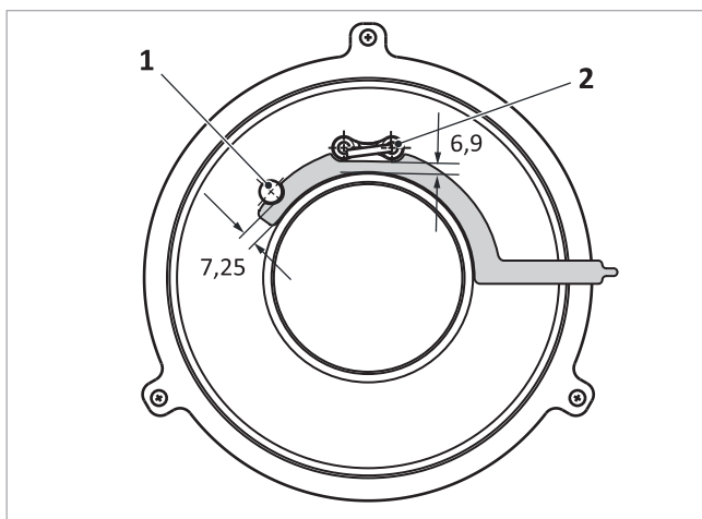
Abb. 47: Abstände Ionisations- und Zündelektrode zum Brennerflansch
