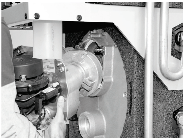
Abb. 70: Brenner einbauen
