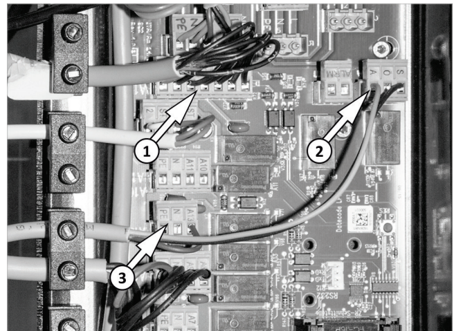
Abb. 77: Anschluss der Brennerstecker Öl-Brenner
