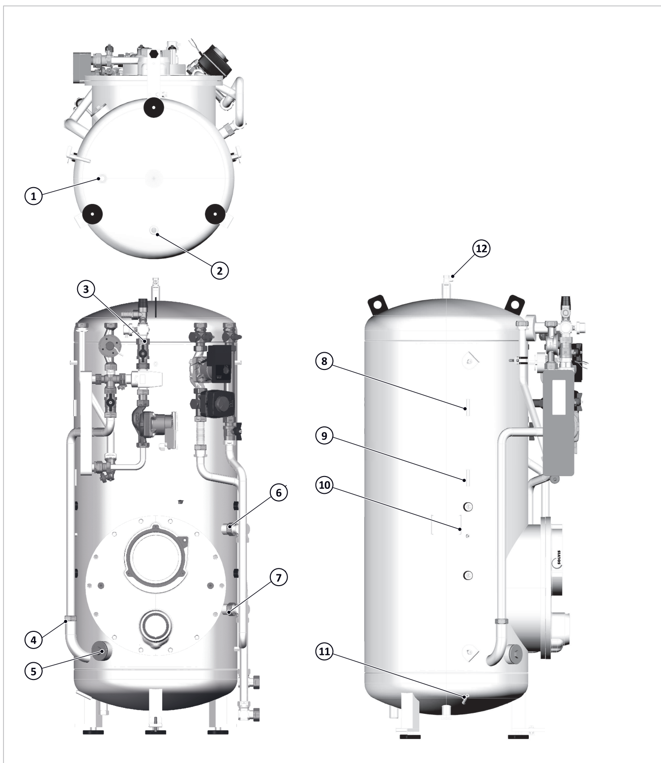
Abb. 162: Frontansicht Schichtenspeicher
