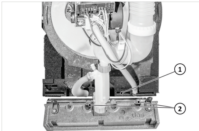
Abb. 94: Leitungen durch Bodenteil führen
