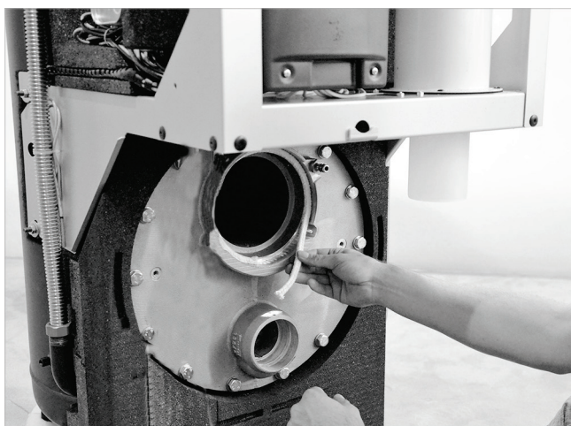
Abb. 64: Brennerdichtschnur einlegen
