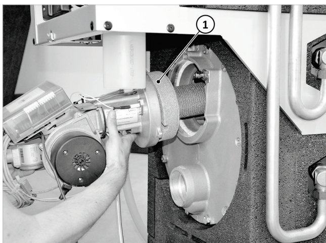
Abb. 49: Brenner einbauen
