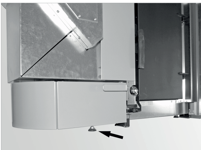
Abb. 103: Stellschraube einrichten
