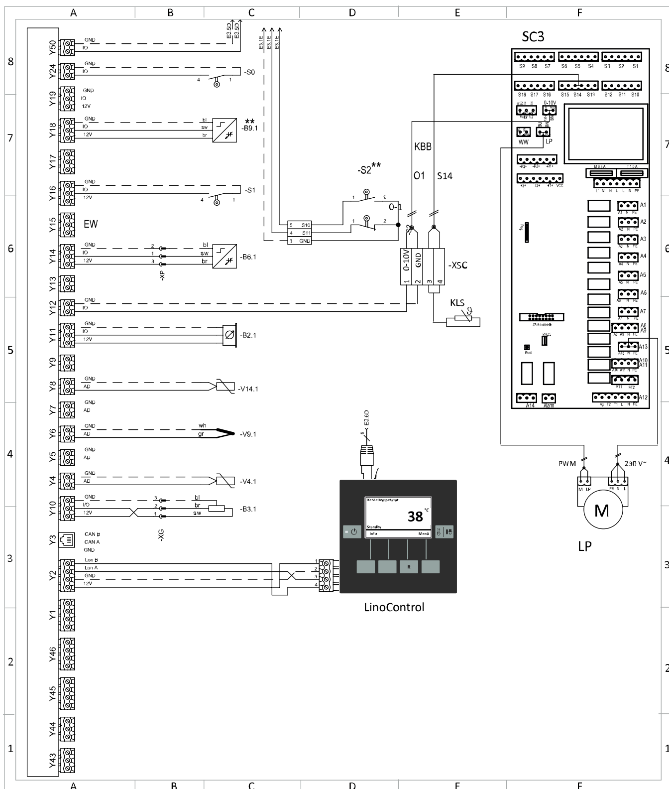
Abb. 187: Grundschaltbild SolvisLino 4 (Plan E2)
