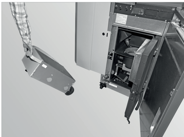
Abb. 168: Aschebehälter entfernen
