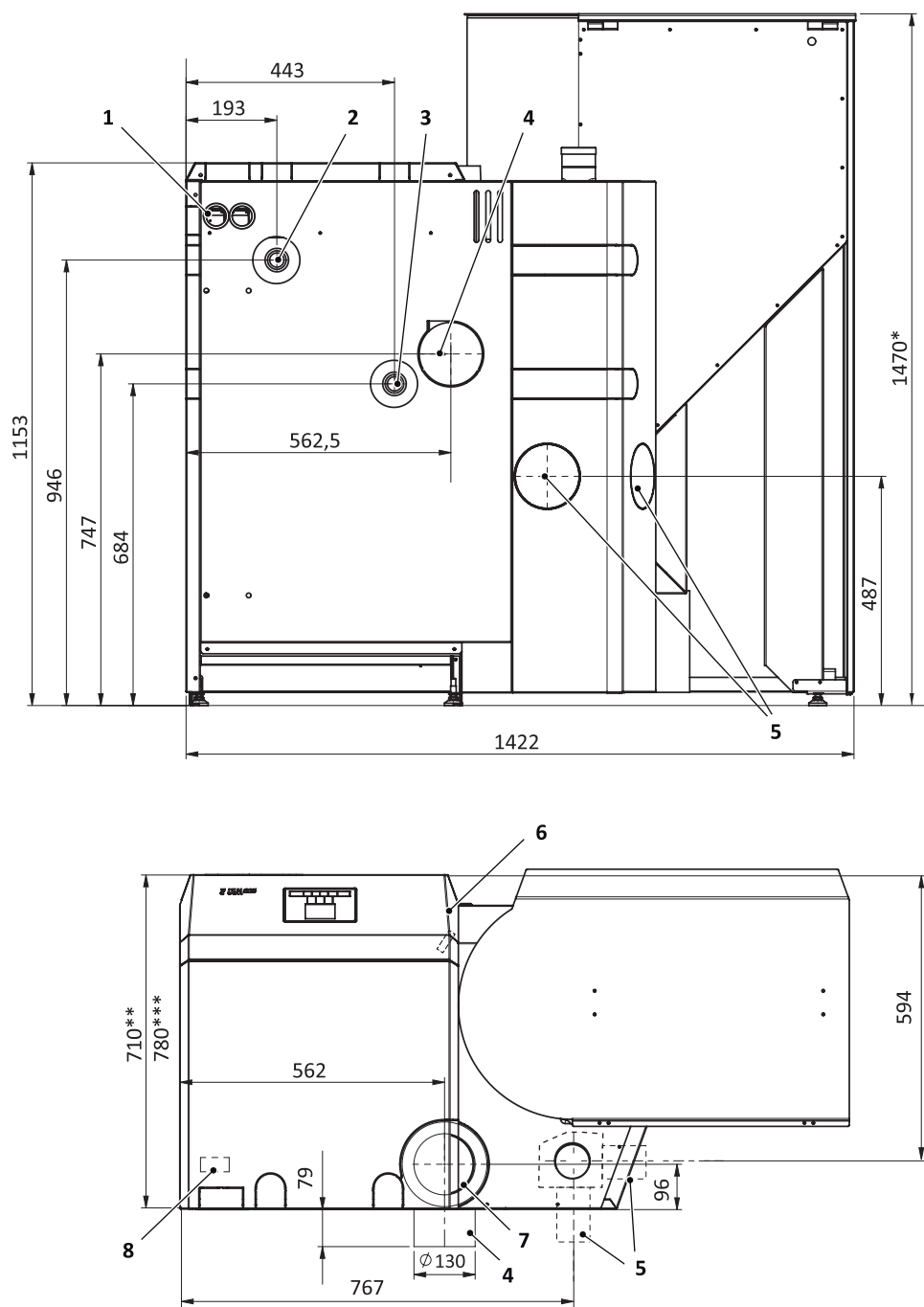
Abb. 181: Ansichten SolvisLino 4 mit Vorratsbehälter (LI-4-xx-VO)
