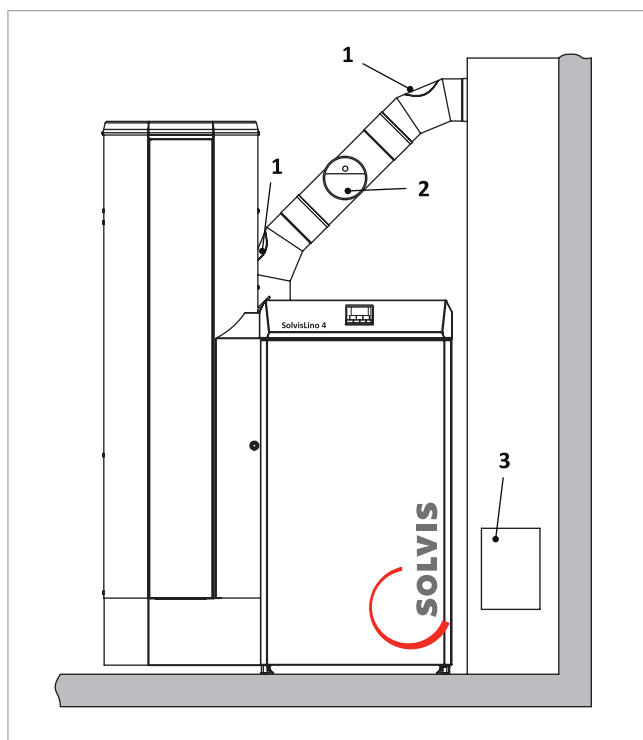
Abb. 163: Reinigungsöffnungen (Ansicht ohne Isolierung)
