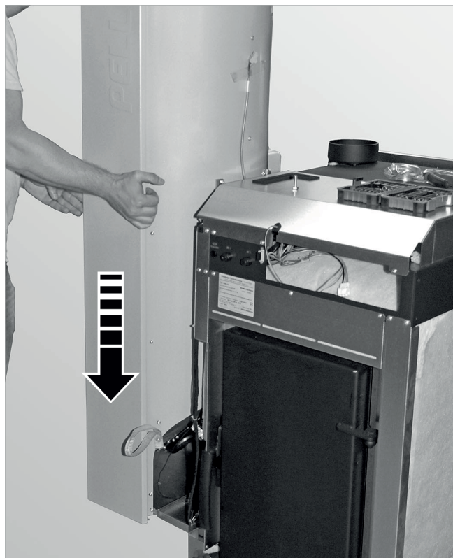
Abb. 33: Blende abnehmen
