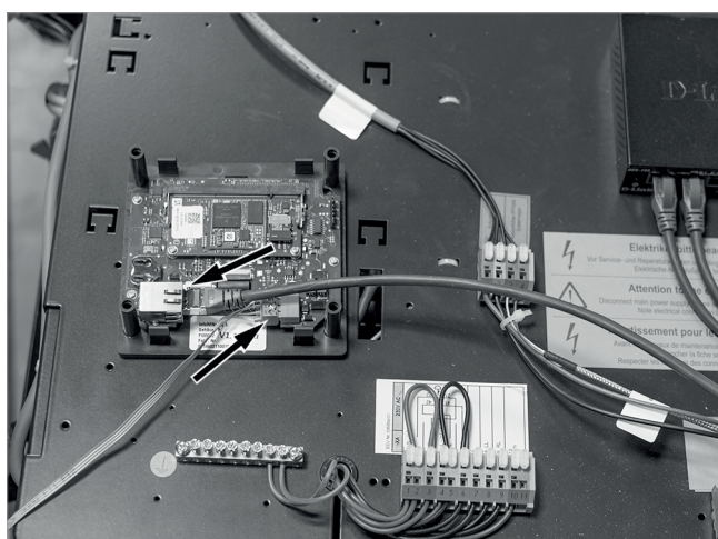
Abb. 91: Kabel zusammenstecken
