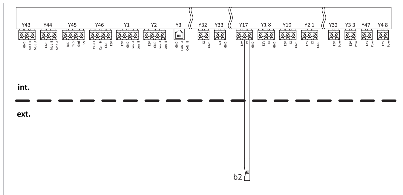
Abb. 195: Anschlussplan Rauchgasthermostat
