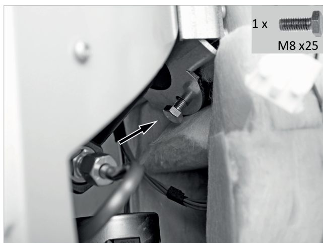
Abb. 31: Vorratsbehälter festschrauben
