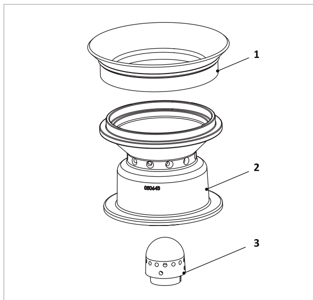
Abb. 153: Zusammenbau Brennertopf
