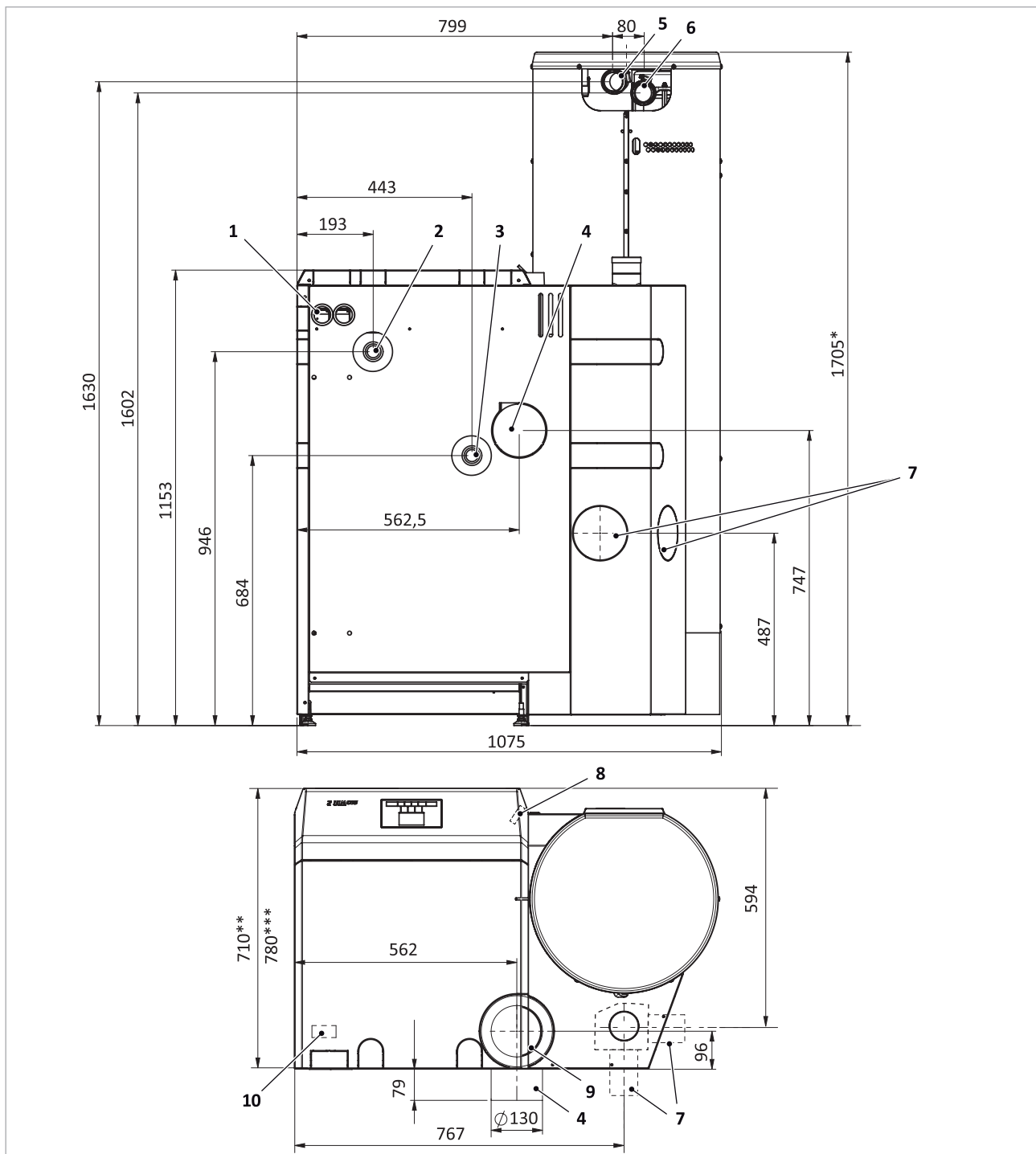
Abb. 180: Ansichten SolvisLino 4 mit Saugturbine (LI-4-xx-GS)
