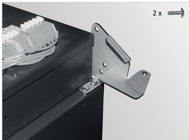
Abb. 85: Türscharnier oben locker anschrauben
