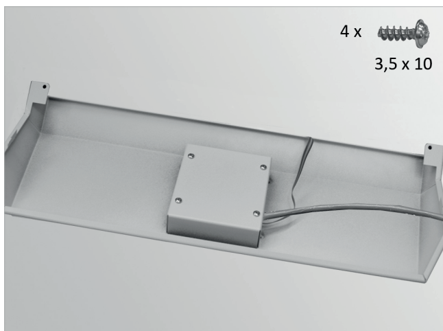
Abb. 92: LinoControl festschrauben
