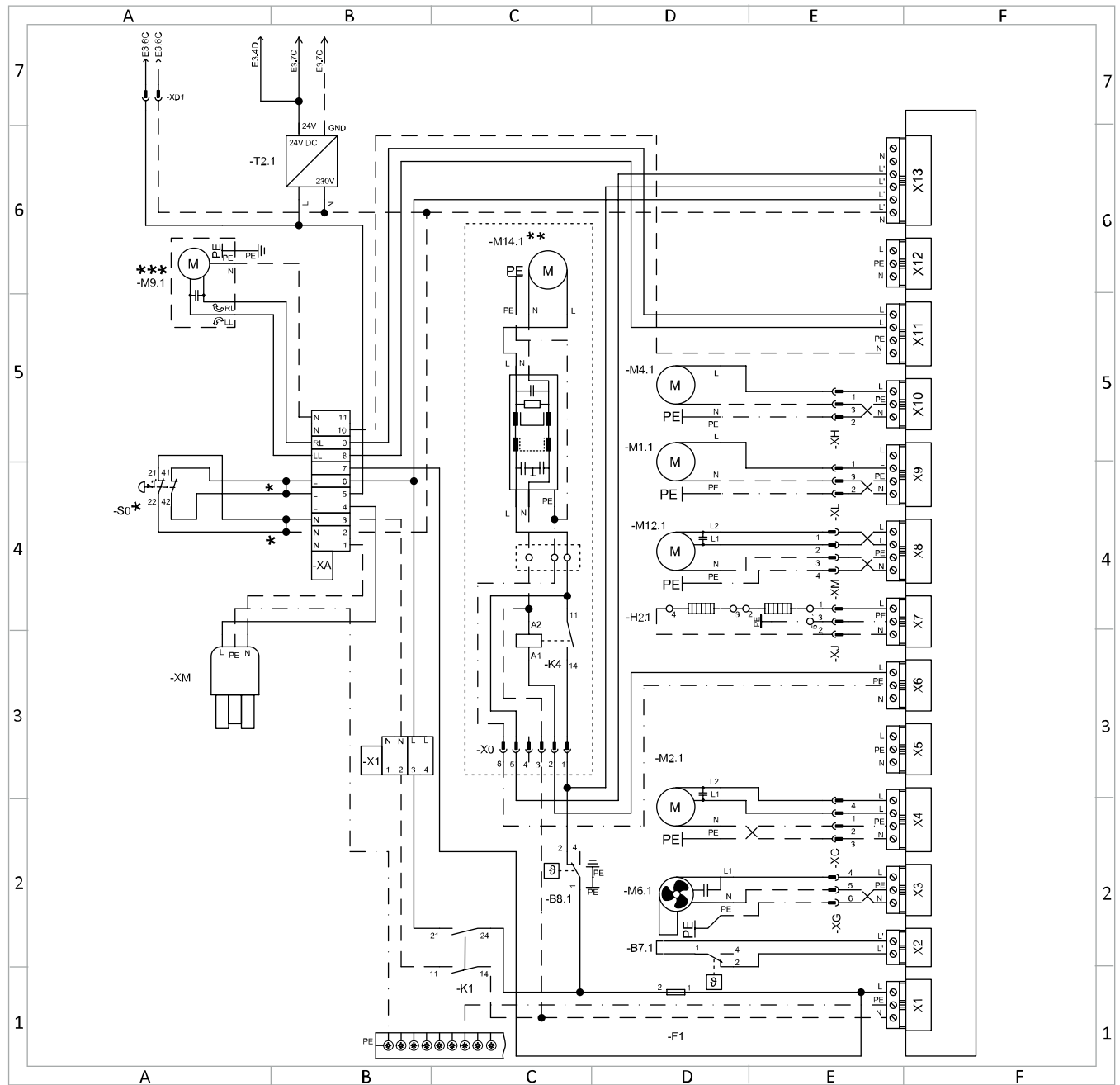
Abb. 186: Grundschaubild SolvisLino 4 (Plan E1)
