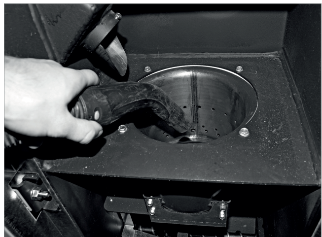
Abb. 148: Brennertopf aussaugen
