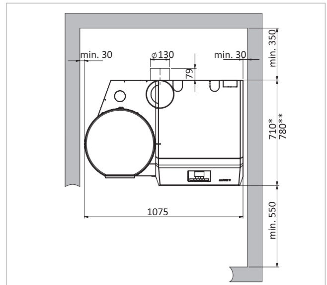
Abb. 183: Mindestabstand Rauchgasrohr hinten (Maße in mm)
