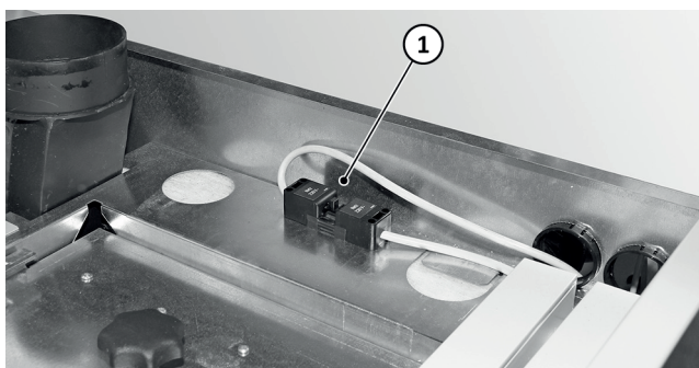
Abb. 167: Geräte-Netzstecker abziehen
