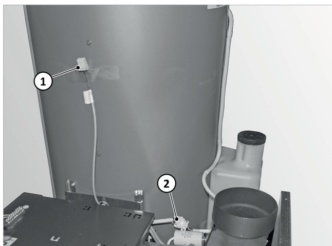
Abb. 40: Netzstecker anstecken
