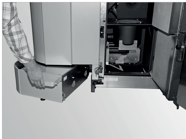
Abb. 135: Behälter leicht nach links drücken
