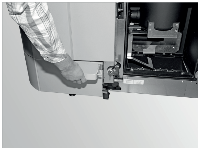
Abb. 133: Griff herausziehen
