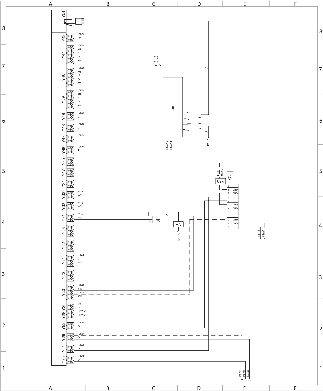
Abb. 188: Grundschriftbild SolvisLino 4 (Plan E3)
