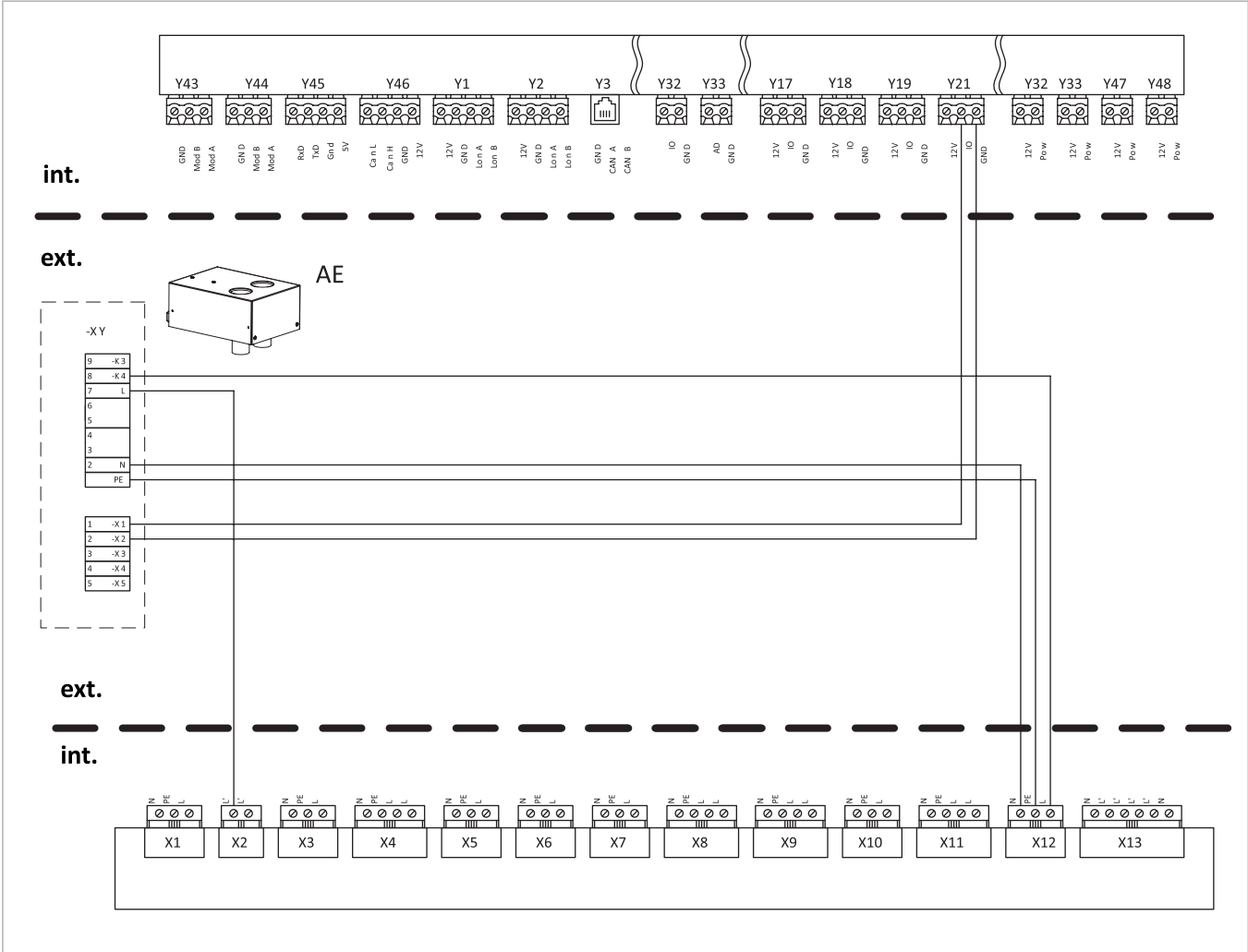
Abb. 192: Anschlussplan Absperreinheit
