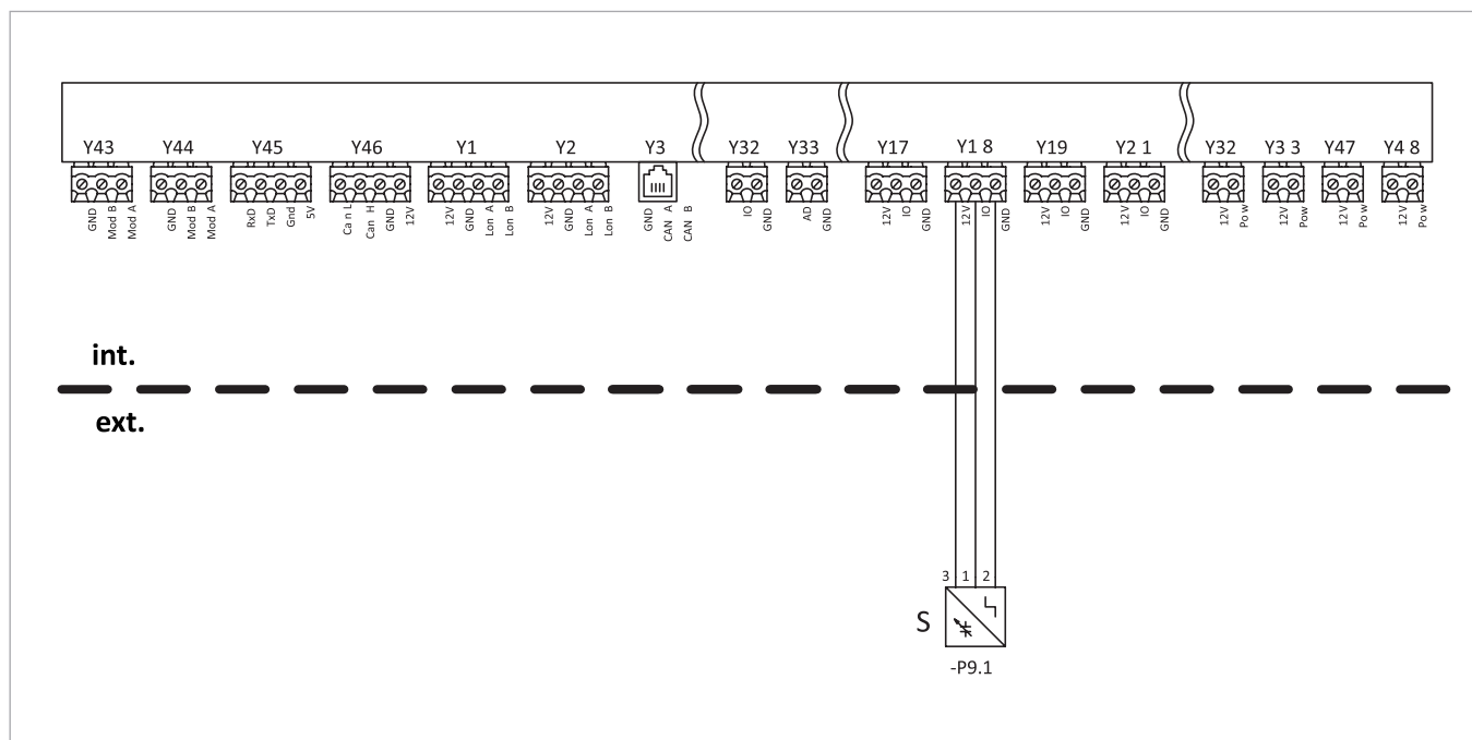
Abb. 193: Anschlussplan Absperreinheit
