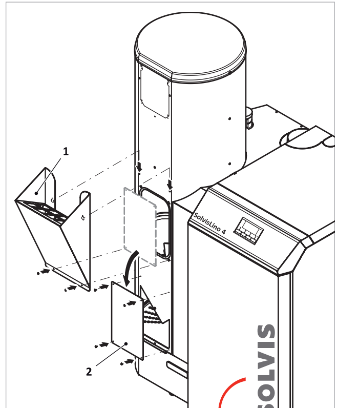
Abb. 174: Pelletschütte und Revisionsdeckel montieren
