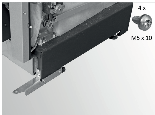
Abb. 84: Türscharnier unten anschrauben
