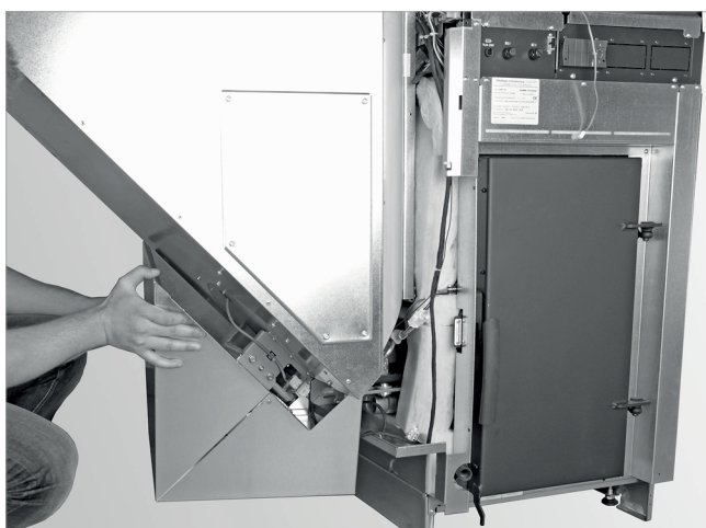
Abb. 66: Abdeckung einhängen
