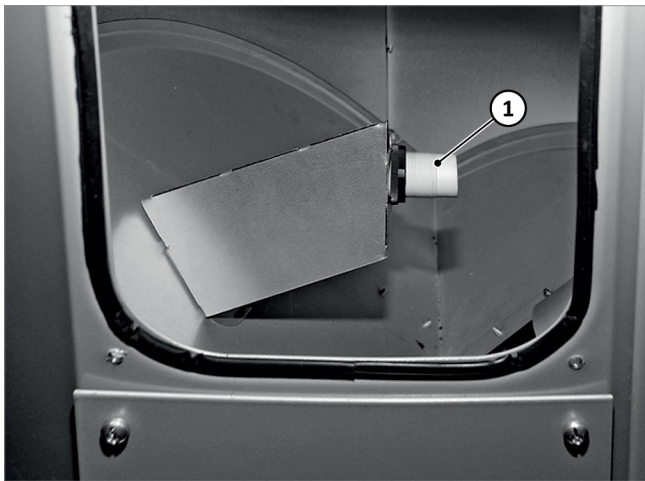
Abb. 173: Näherungsschalter reinigen
