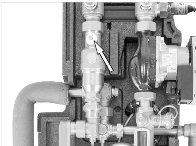
Abb. 25: Luftfang entlüften
