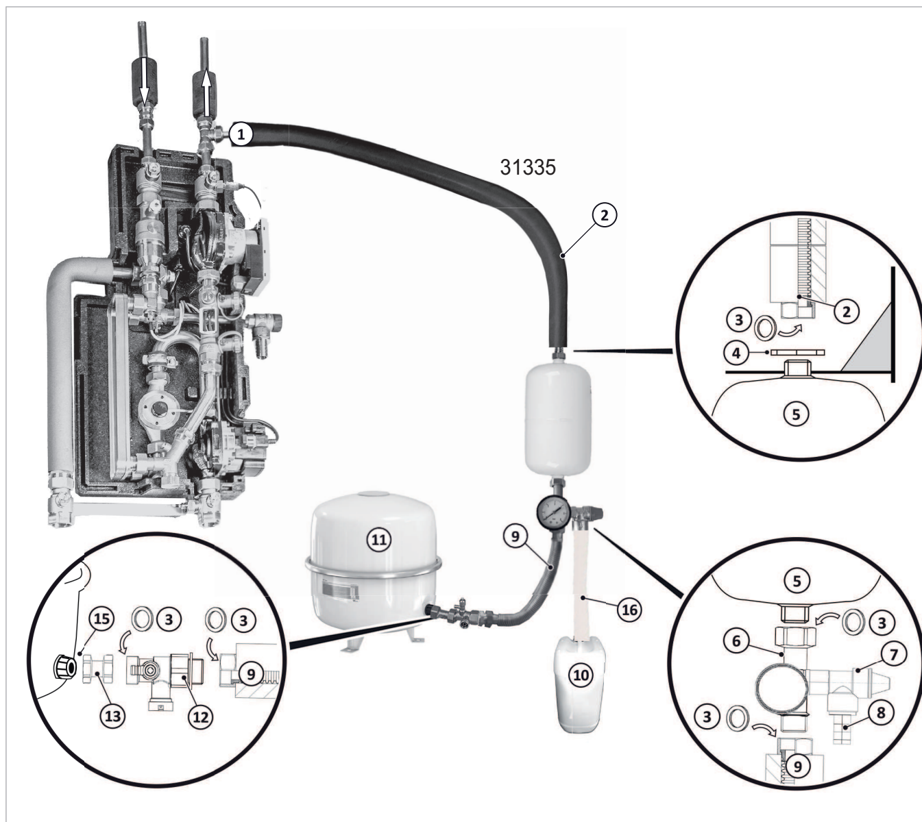
Abb. 5: Anbindung Solar-MAG
