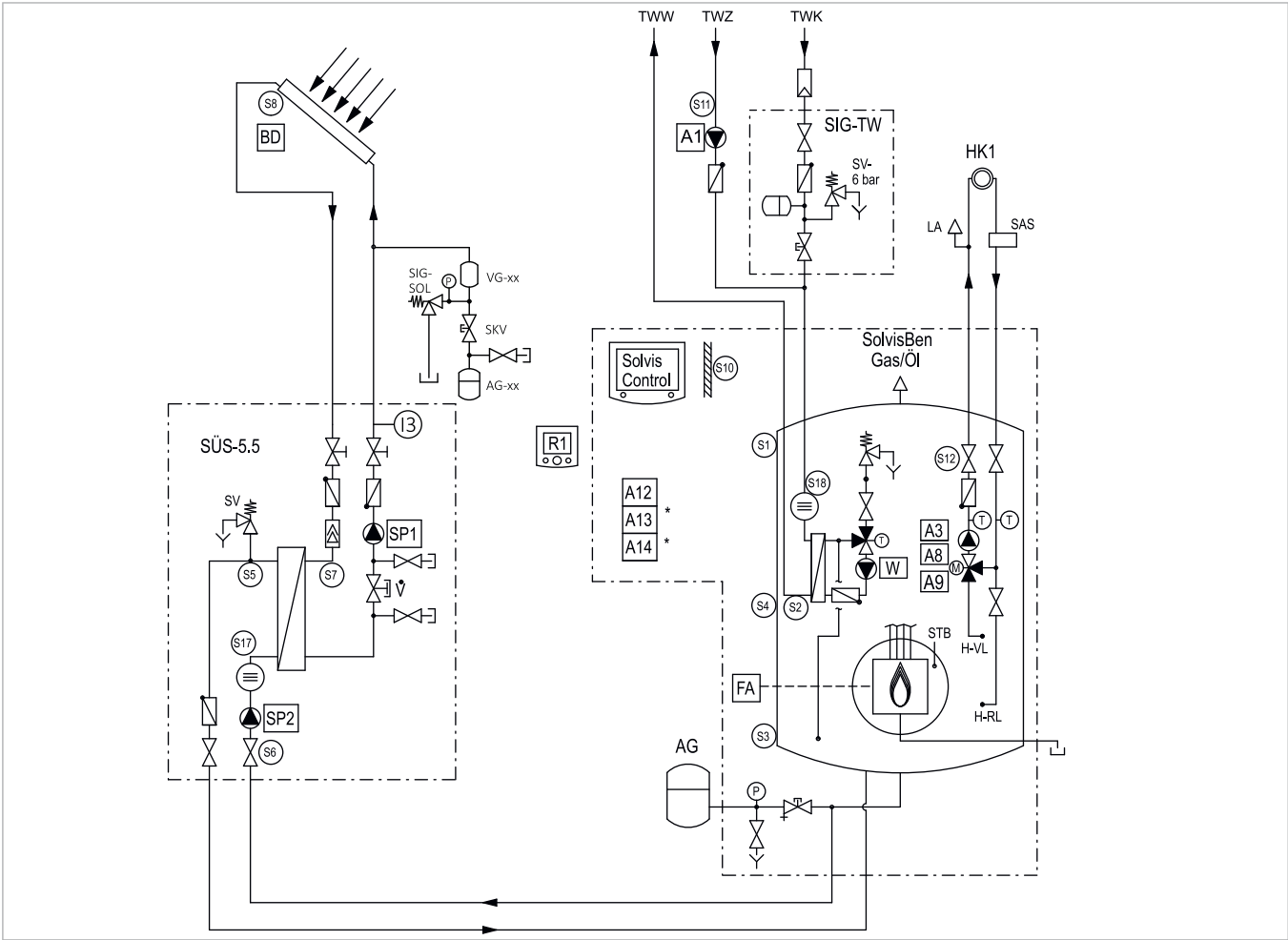
Abb. 29: SolvisBen Gas / SolvisBen Öl mit integrierter Heizkreisstation und Solaranlage
