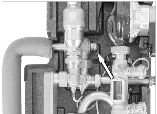
Abb. 17: Handentlüfter Sekundärseite
