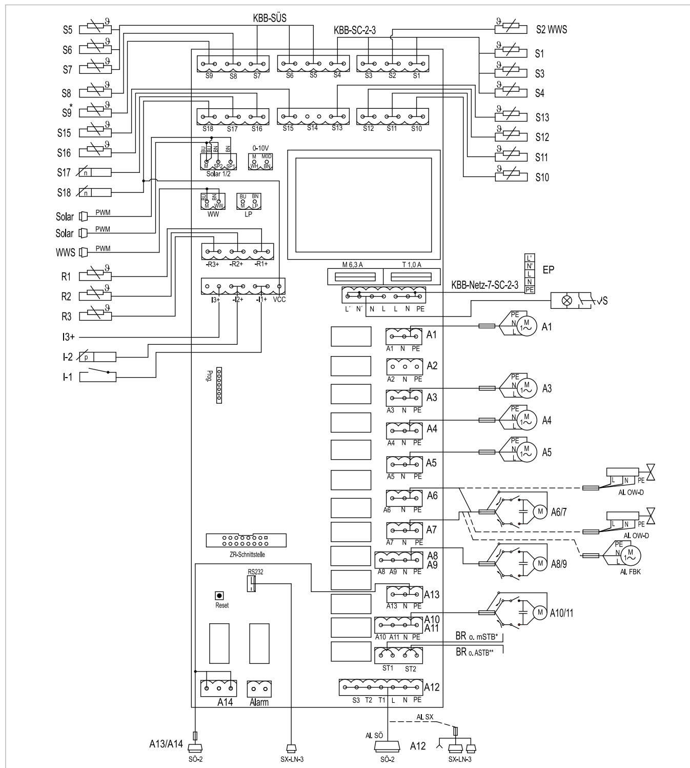
Abb. 30: Netzbaugruppe SolvisControl 3 für SolvisBen Gas und Öl
