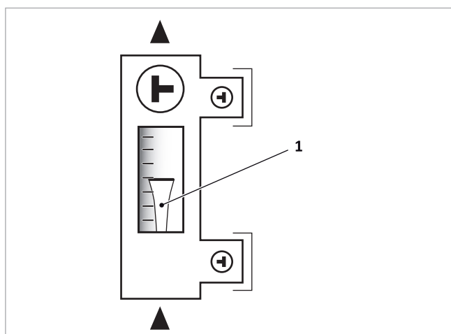
Abb. 22: Volumenstrom an oberer Kante des Schwebekörpers (1) ablesen
