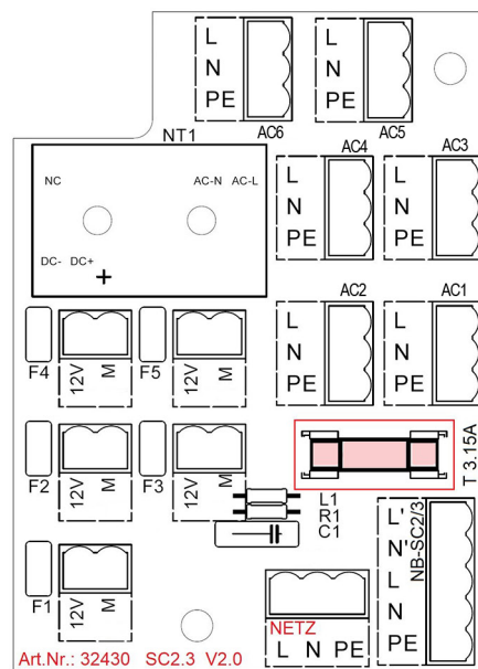
Abb. 31: Erweiterungsplatine für die Netzplatine der SolvisControl 3
