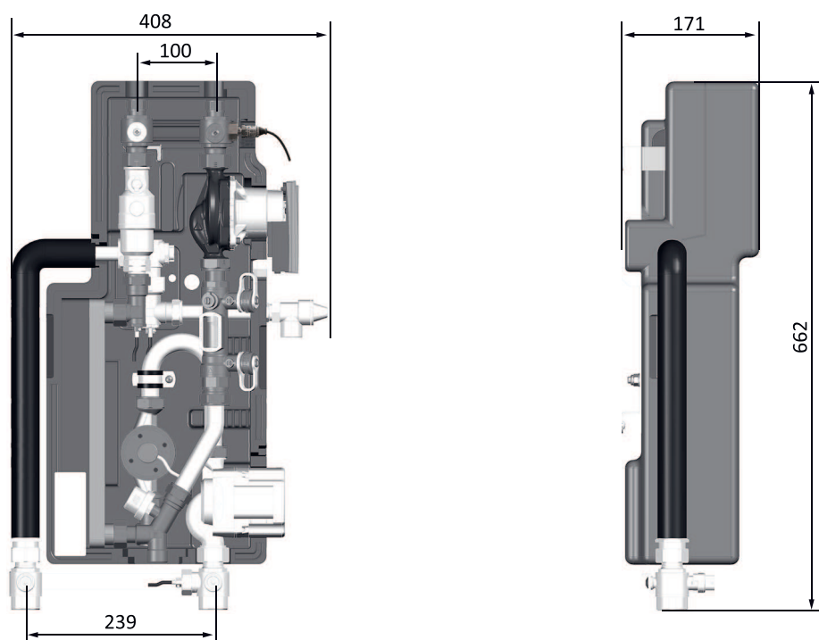
Abb. 26: Abmessungen der Solarwärmeübergabestation
