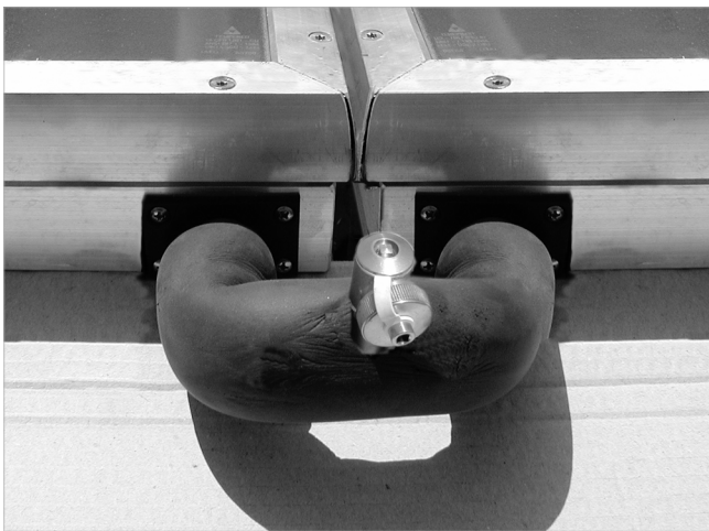
Abb. 24: Beispiel am SolvisFera Diagonal mit SFE-Hahn
