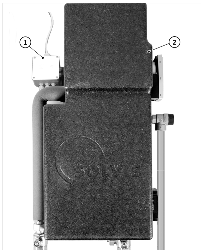
Abb. 11: Anschlussdose montiert
