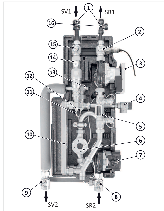
Abb. 1: Solarwärmeübergabestation
