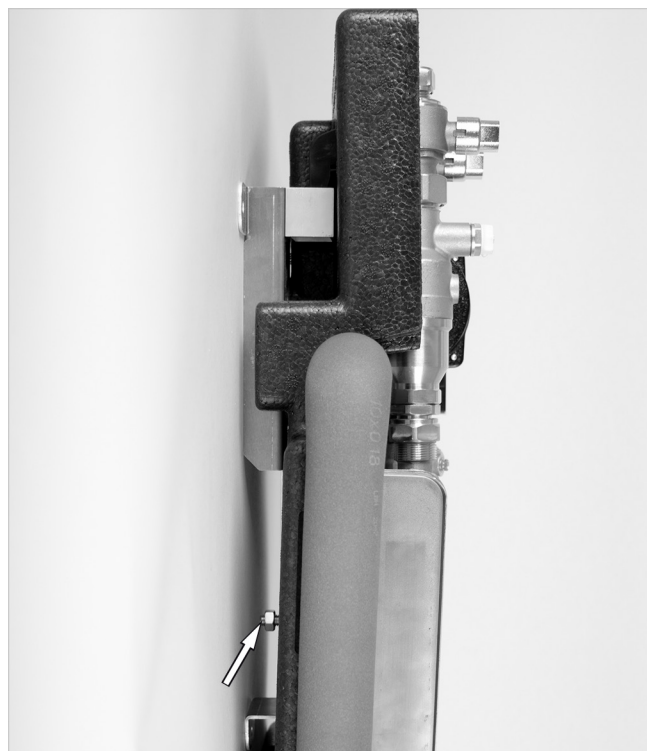
Abb. 4: Mutter festziehen
