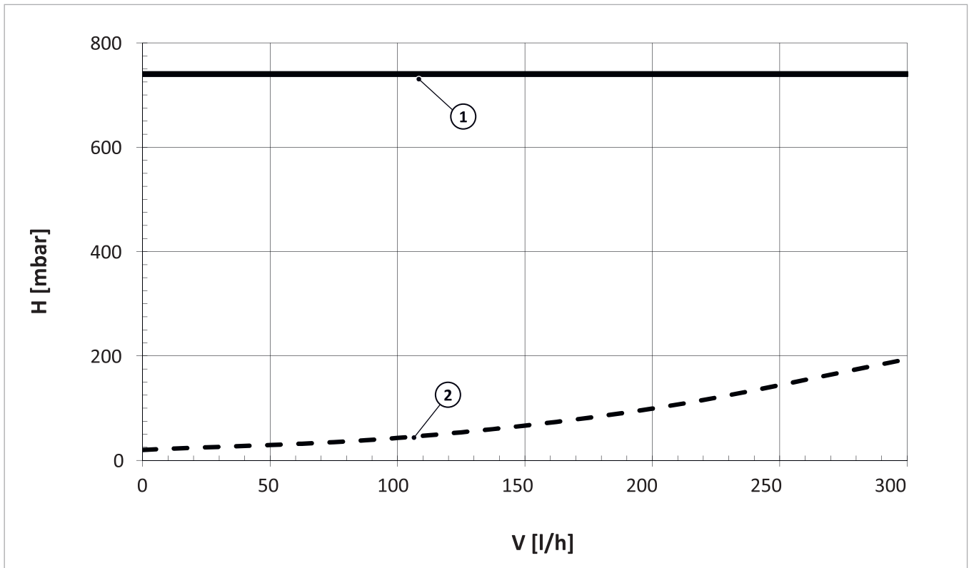
Abb. 27: Druckverlustkurve des Primärkreises SÜS-5,5
