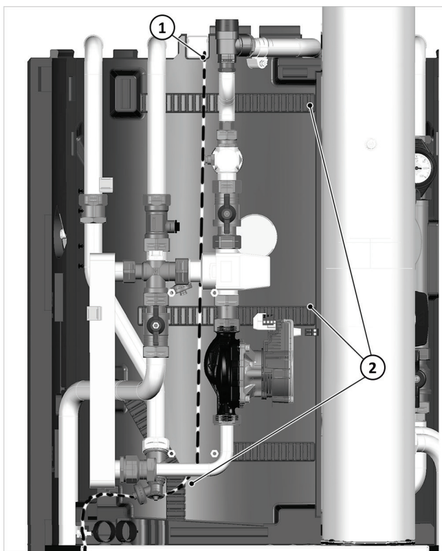
Afb. 103: Kabelgeleiding door de WWS-isolatie
