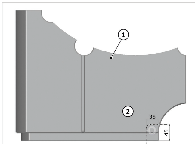
Afb. 127: Eventueel doorvoer gasleiding opensnijden
