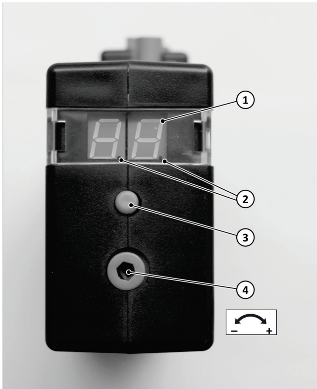
Afb. 152: Interface branderautomaat CM 168
