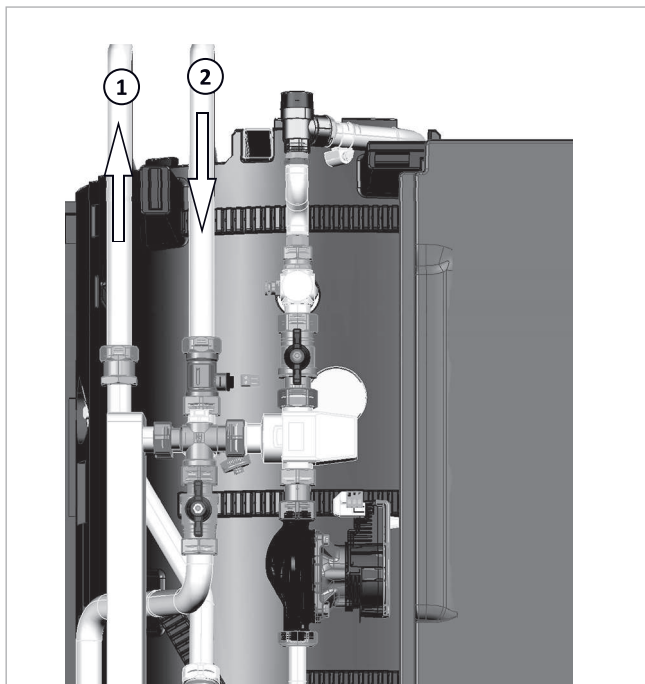
Afb. 28: TWW-/TWK-aansluiting van bovenaf
