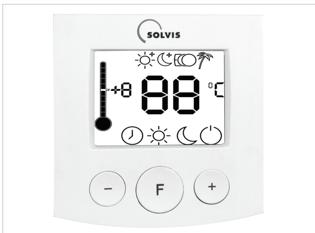
Afb. 107: Ruimtebedieningselement BE-SC-2
