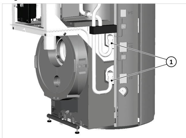
Afb. 31: De aansluitingen van de HKS controleren/vastdraaien
