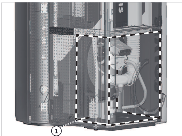
Afb. 1: Aanzuigkamer SolvisBen
