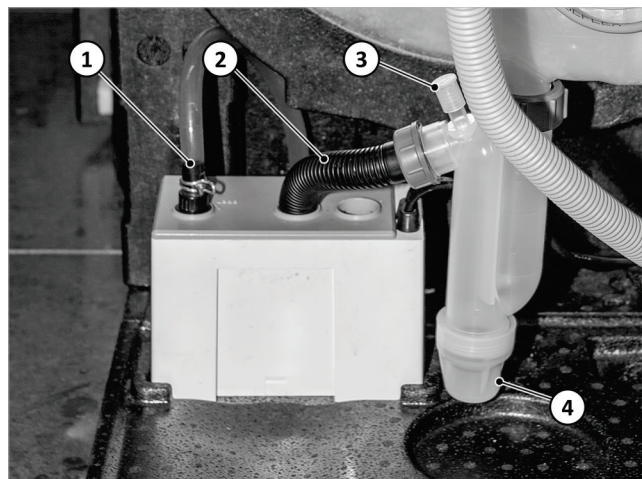
Afb. 91: Condenspomp, aangesloten
