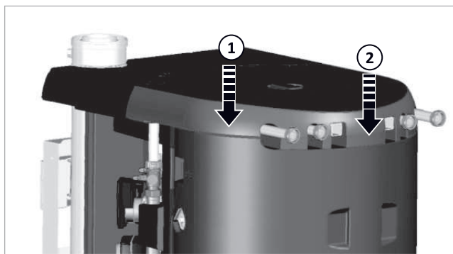
Afb. 129: Koppelingsprofiel rechts en achter
