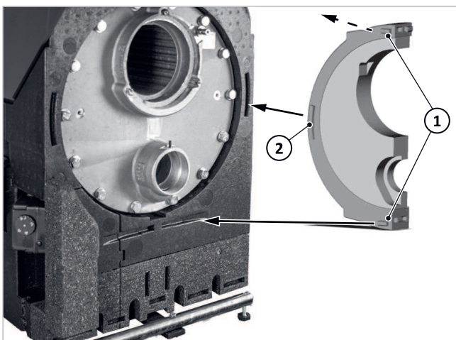
Afb. 99: Voorste flensisolatie (rechts, achteraanzicht) met vergrendelingsveren
