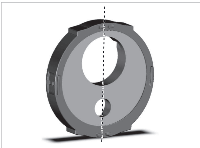
Afb. 98: Flensisolatie aan de voorkant (vooraanzicht) met scheidingsvlak
