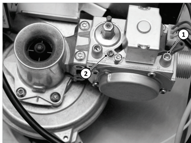
Afb. 115: Brander instellen
