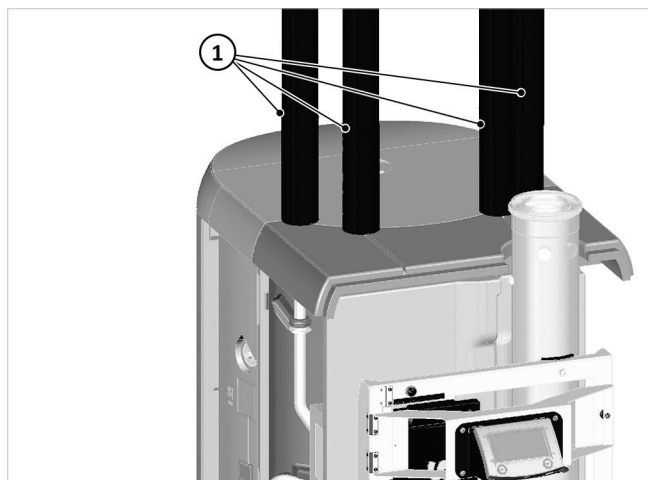
Afb. 128: Bovenste isolatiedelen met de aansluitingen van bovenaf
