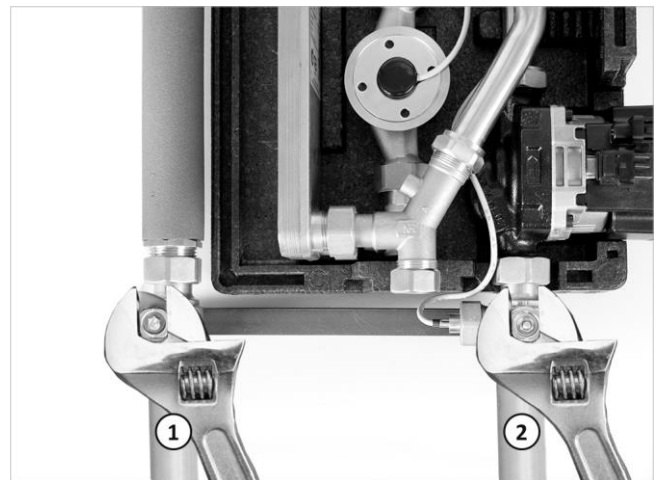
Afb. 16: Beide kogelkranen volledig geopend
