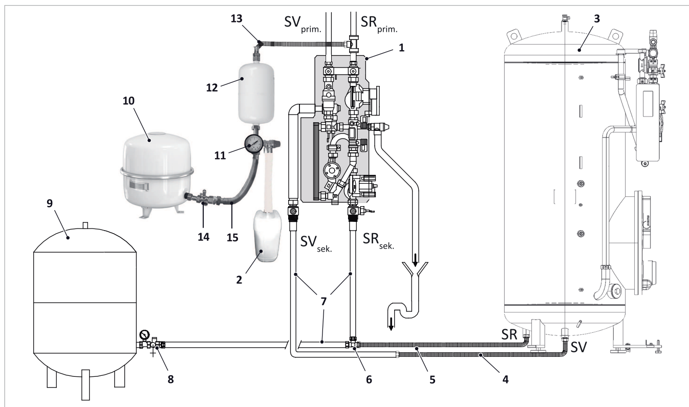
Afb. 2: Montage SUES-5.5, SOL-MAG en H-MAG op SolvisBen
