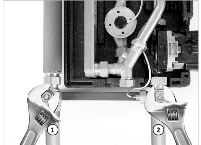
Afb. 15: kogelkranen half geopend / geheel geopend
