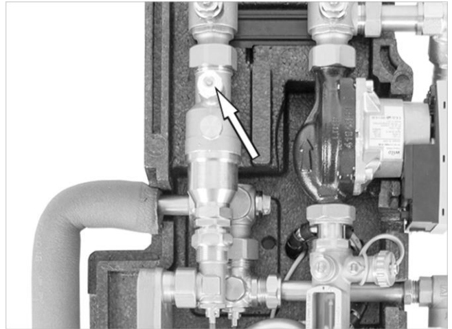
Afb. 24: Luchtvanger ontluchten
