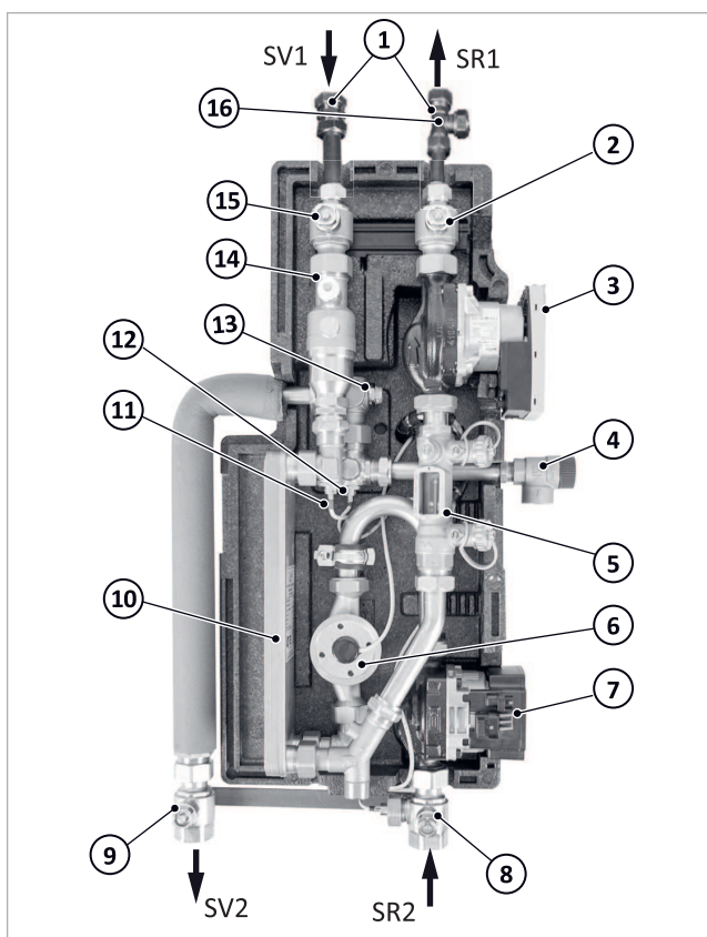
Afb. 1: Zonnewarmte-overdrachtsgroep
