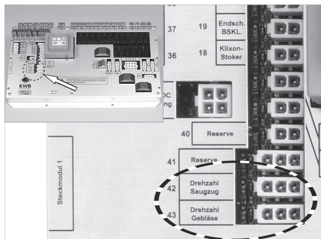
Abb. 8: Stecker 42 un 43 ohne Funktion
