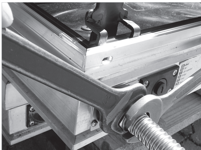
Fig. 9: Fije el tubo ondulado en el exterior.
