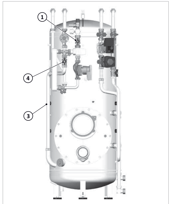
Abb. 3: Frontansicht SolvisBen
