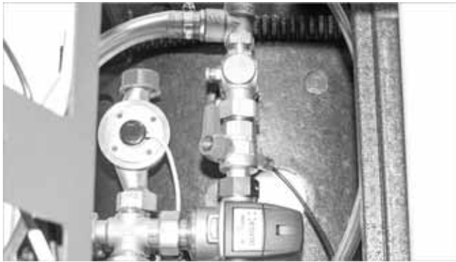
Abb. 4: Kugelhahn mit Tauchsensord, leicht schräg eingebaut
