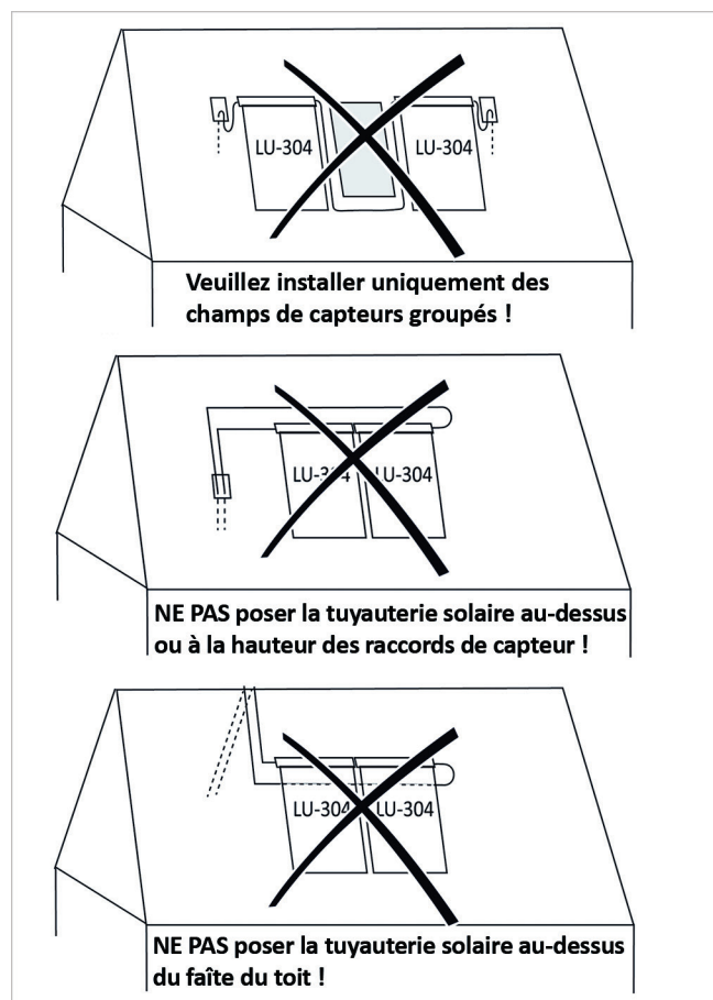
Fig. 6 : installation incorrecte de la tuyauterie solaire
