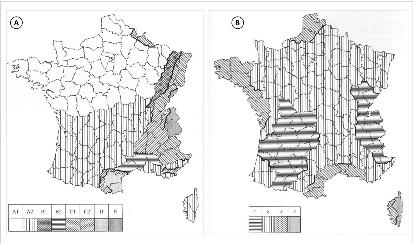
Fig. 50: répartition des zones de charge de neige et vent en France
