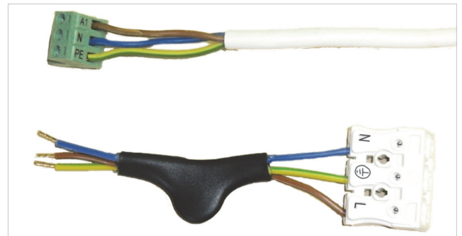
Abb. 1: Anschlusskabel und Zwischenstecker
