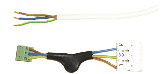
Abb. 2: 3-poligen Stecker anschließen
