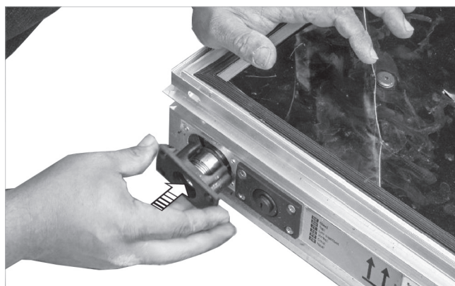
Abb. 11: Anschlussfittinghalter montieren
