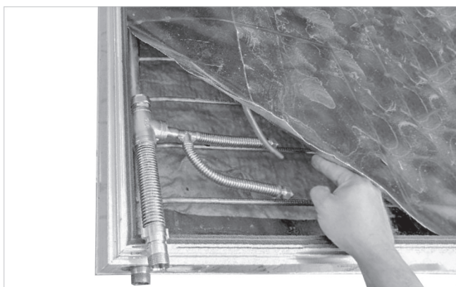
Abb. 3: Reparaturrohr auflegen
