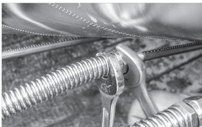
Abb. 9: Klemmringverschraubung festziehen
