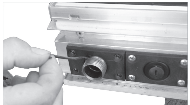
Abb. 1: Schrauben und O-Ring entfernen
