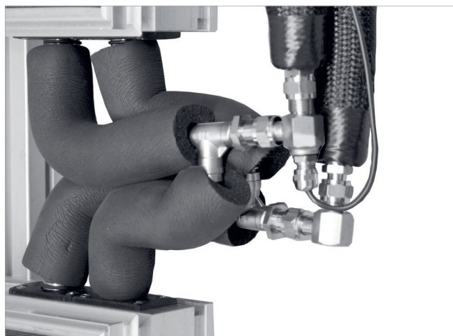
Fig. 53: collegamento a vite parallelo installato in modo incrociato
