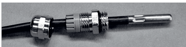
Fig. 70: inserimento del collegamento a vite PG sul sensore a immersione
