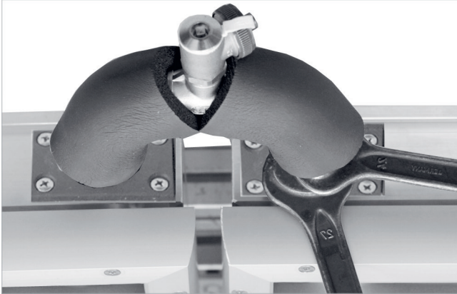
Fig. 67: collegamento dei collettori l'uno accanto all'altro
