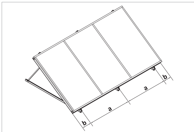
Fig. 20: dimensioni delle distanze supporti per tetto piano
