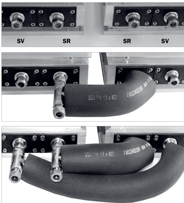
Fig. 48: Montaggio del raccordo filettato parallelo
