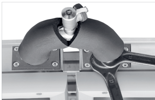
Fig. 64: collegamento dei collettori l'uno accanto all'altro
