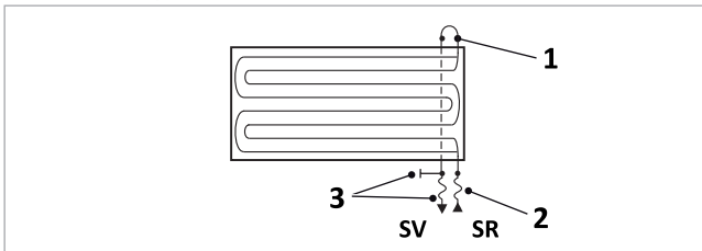
Fig. 42: SolvisFera Integral, cavi di collegamento in basso
