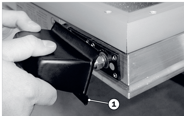
Fig. 51: posizionamento della calotta di protezione
