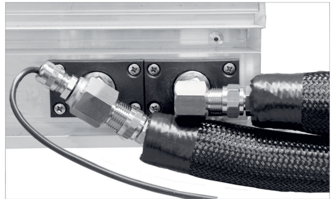
Fig. 44: Raccordo flessibile con isolamento
