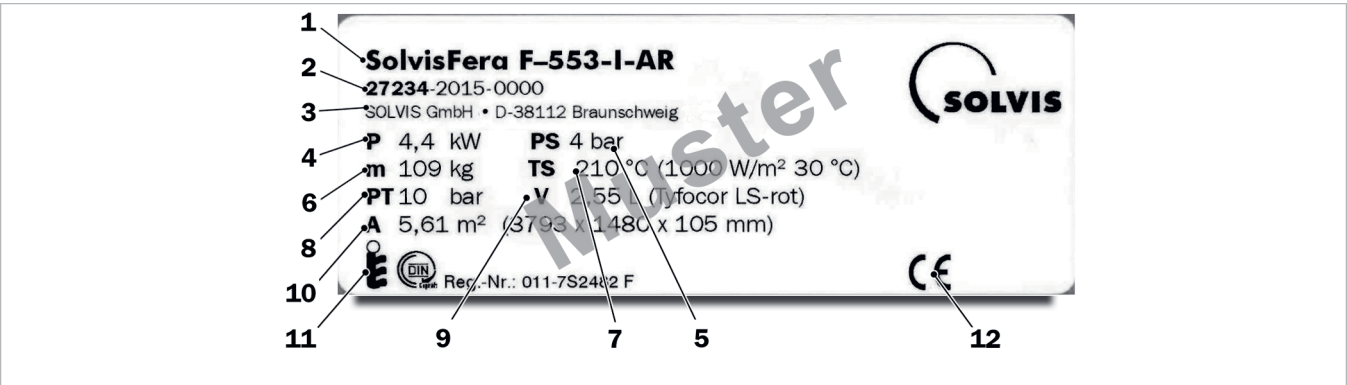
Fig. 78: Esempio di targhetta SolvisFera
