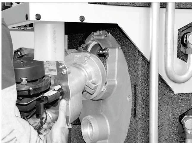
Fig. 70: Montaggio del bruciatore
