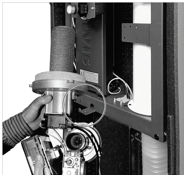
Fig. 141: Aggancio del bruciatore alla console (posizione di manutenzione)
