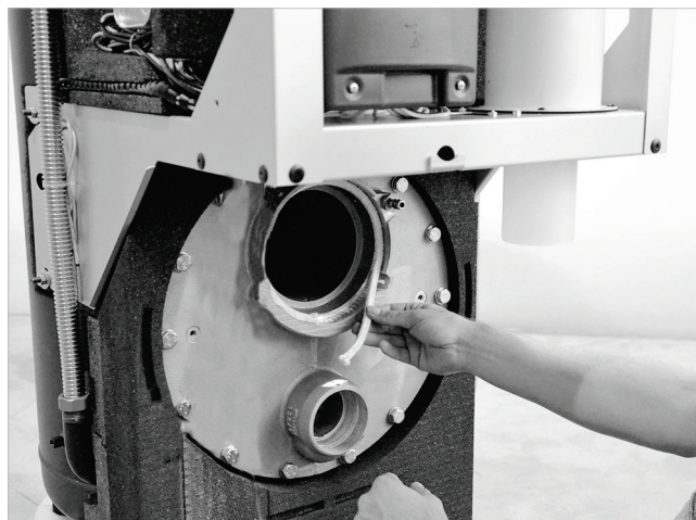
Fig. 46: Inserire il cordoncino di tenuta del bruciatore
