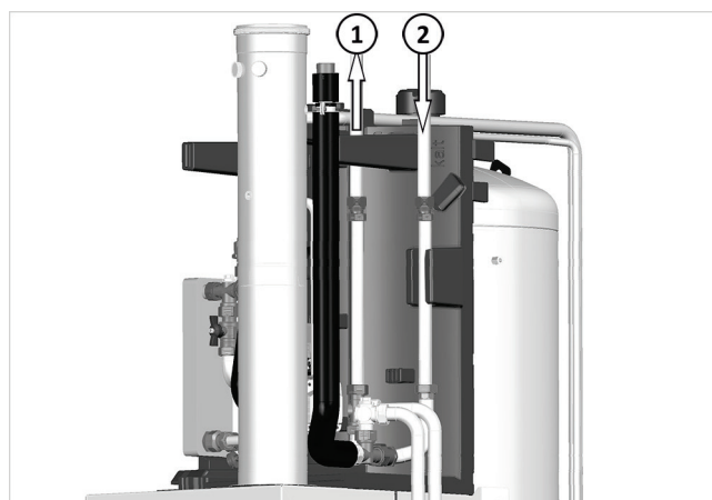
Fig. 39: attacco H-VL /H-RL dall'alto
