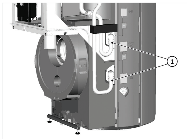
Fig. 31: Controllare/serrare gli attacchi della SCR
