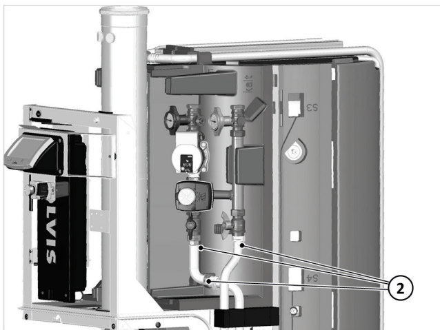
Fig. 32: Controllare/serrare gli attacchi angolo di mandata/ritorno
