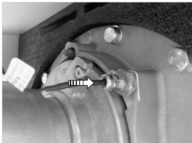
Fig. 71: inserimento del mSTB
