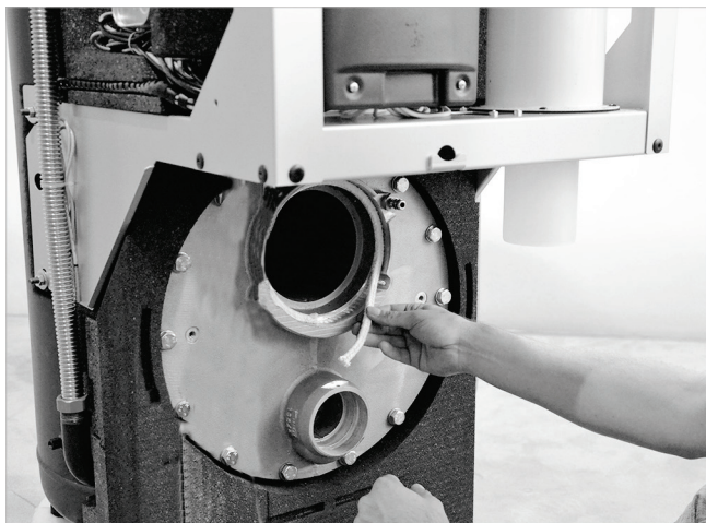
Fig. 64: Inserire il cordoncino di tenuta del bruciatore
