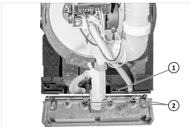
Fig. 94: Far passare le tubazioni attraverso la base
