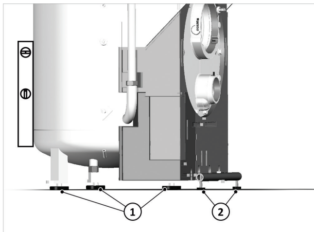
Fig. 5: installazione dell'accumulatore
