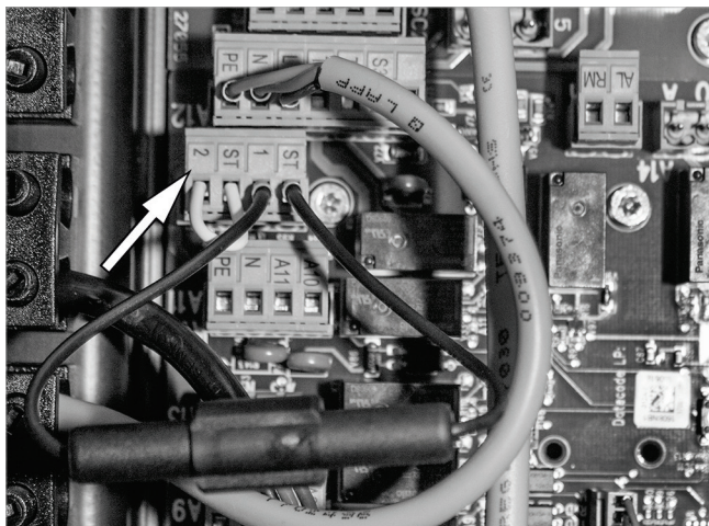
Fig. 57: Inserire la presa di collegamento
