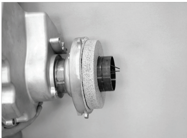
Fig. 68: applicazione del portello caldaia con isolante refrattario
