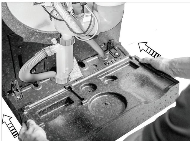
Fig. 97: Innestare la parte anteriore della base
