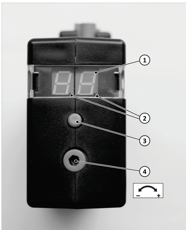
Fig. 117: Impostazione del numero di giri del soffiante dall'interfaccia
