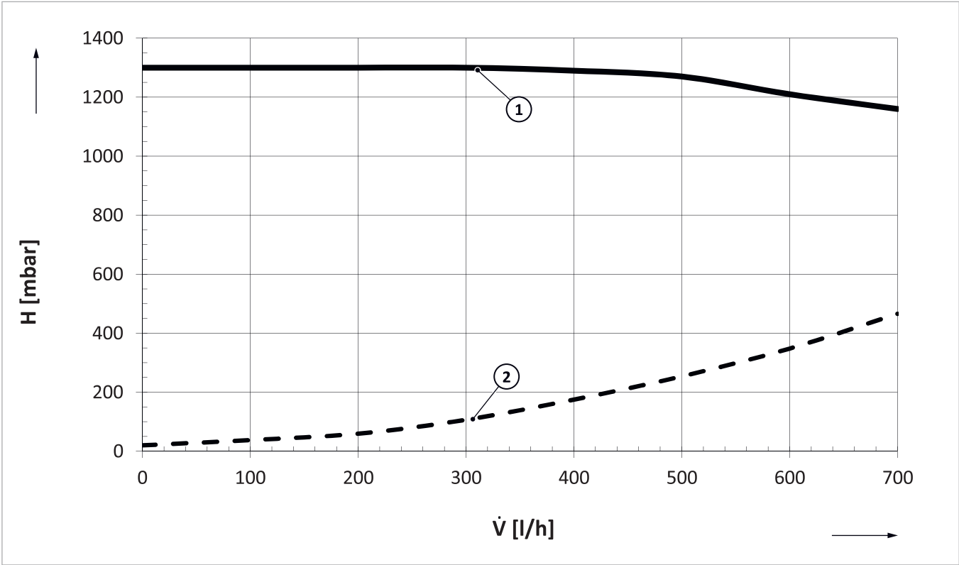
Fig. 28: Curva della perdita di pressione del circuito primario
