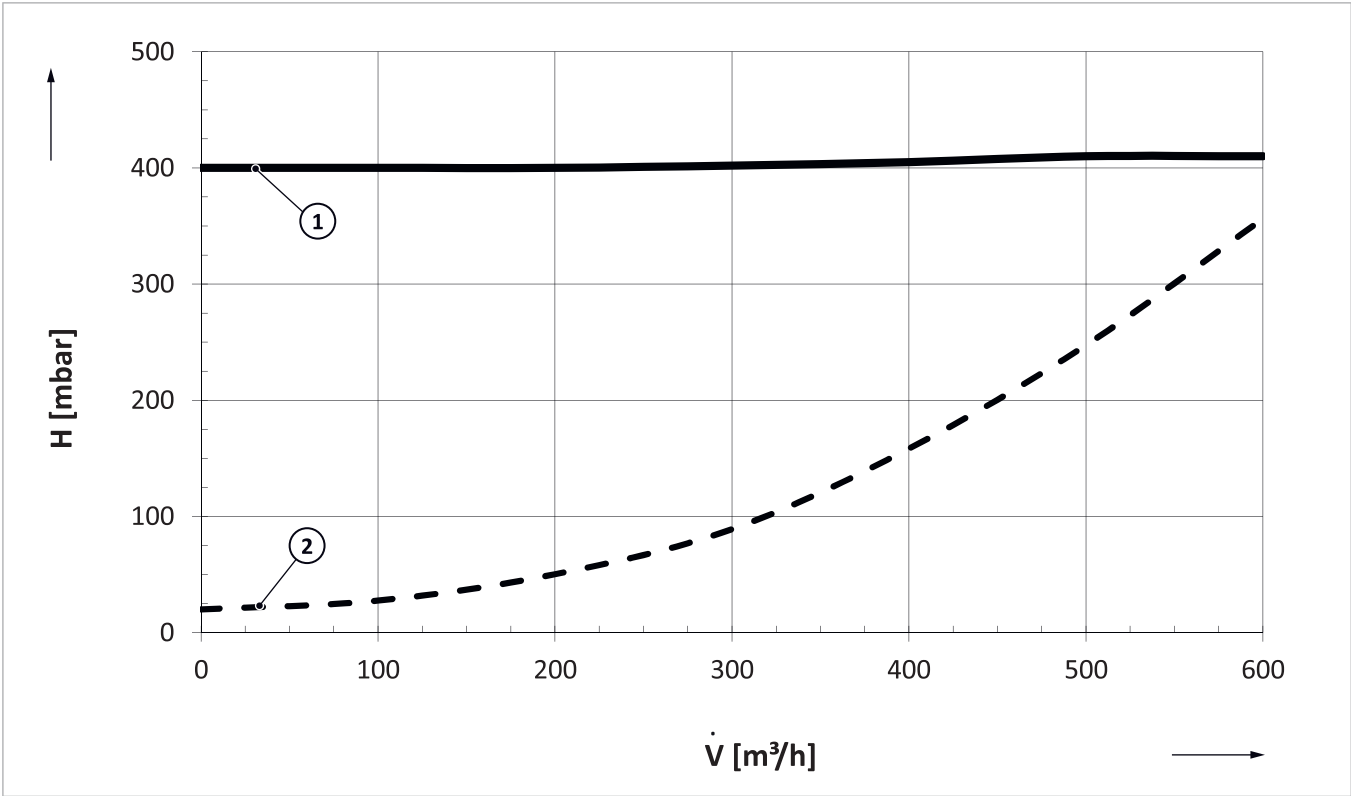
Fig. 29: Curva della perdita di pressione del circuito secondario
