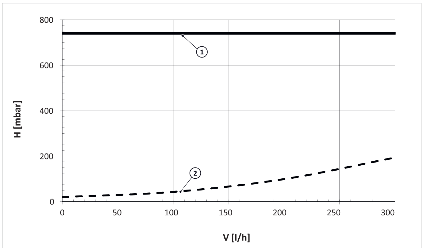
Fig. 26: Curva perdita di pressione del circuito primario SÜS-5,5
