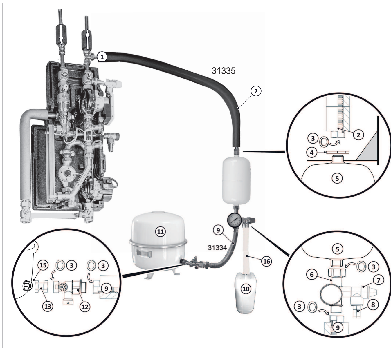
Fig. 5: Collegamento Solar-MAG
