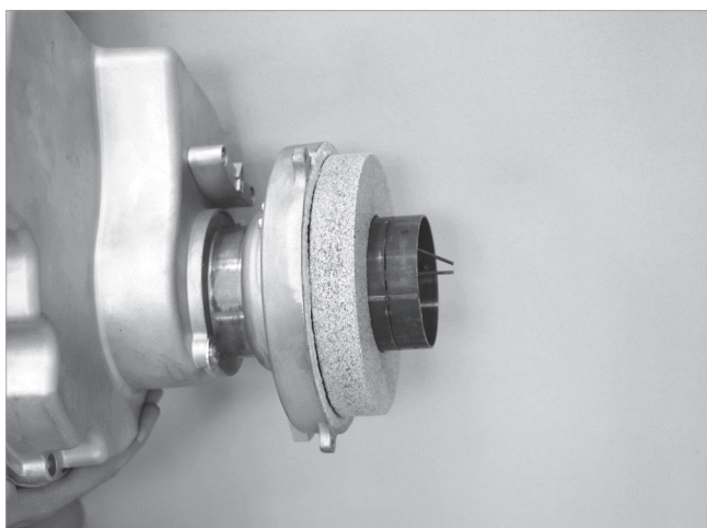
Afb. 5: Keteldeurisolatie plaatsen
