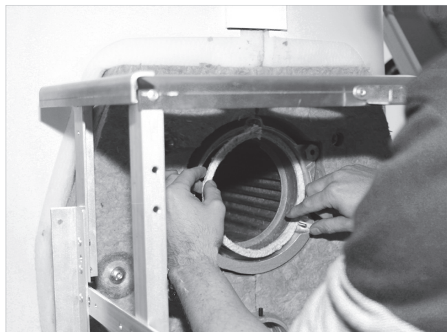
Afb. 1: Branderafdichtband plaatsen
