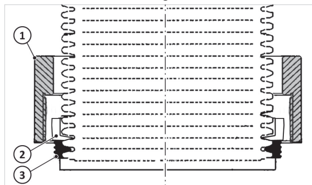
Afb. 10: Schroefkoppeling opgestoken
