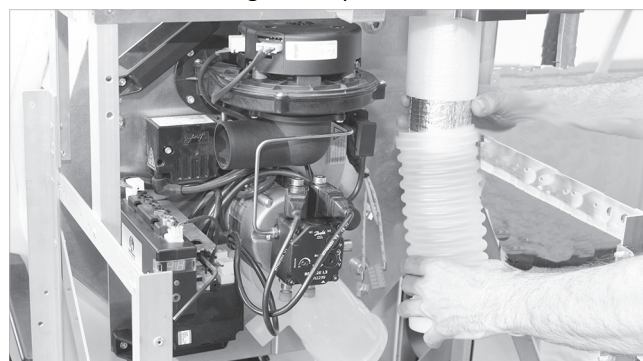
Afb.12: Rookgasaansluitstuk opsteken
