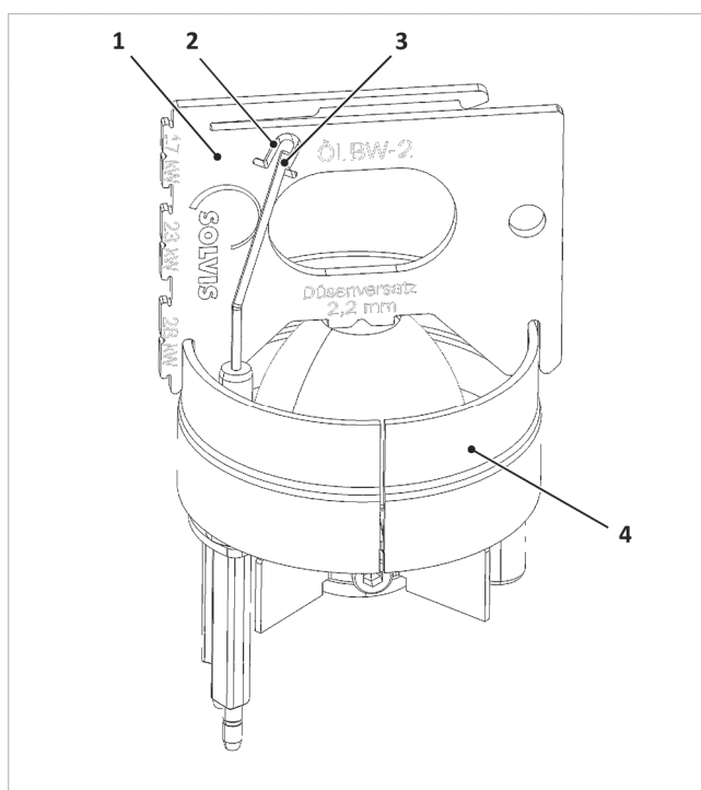
Afb. 36: Ontstekingselektroden controleren
