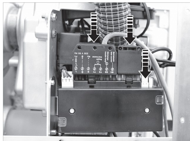
Afb. 23: Stekker opsteken
