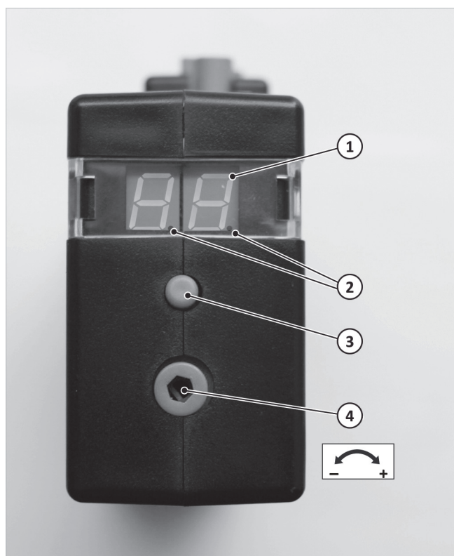
Afb. 39: Interface branderautomaat CM 168
