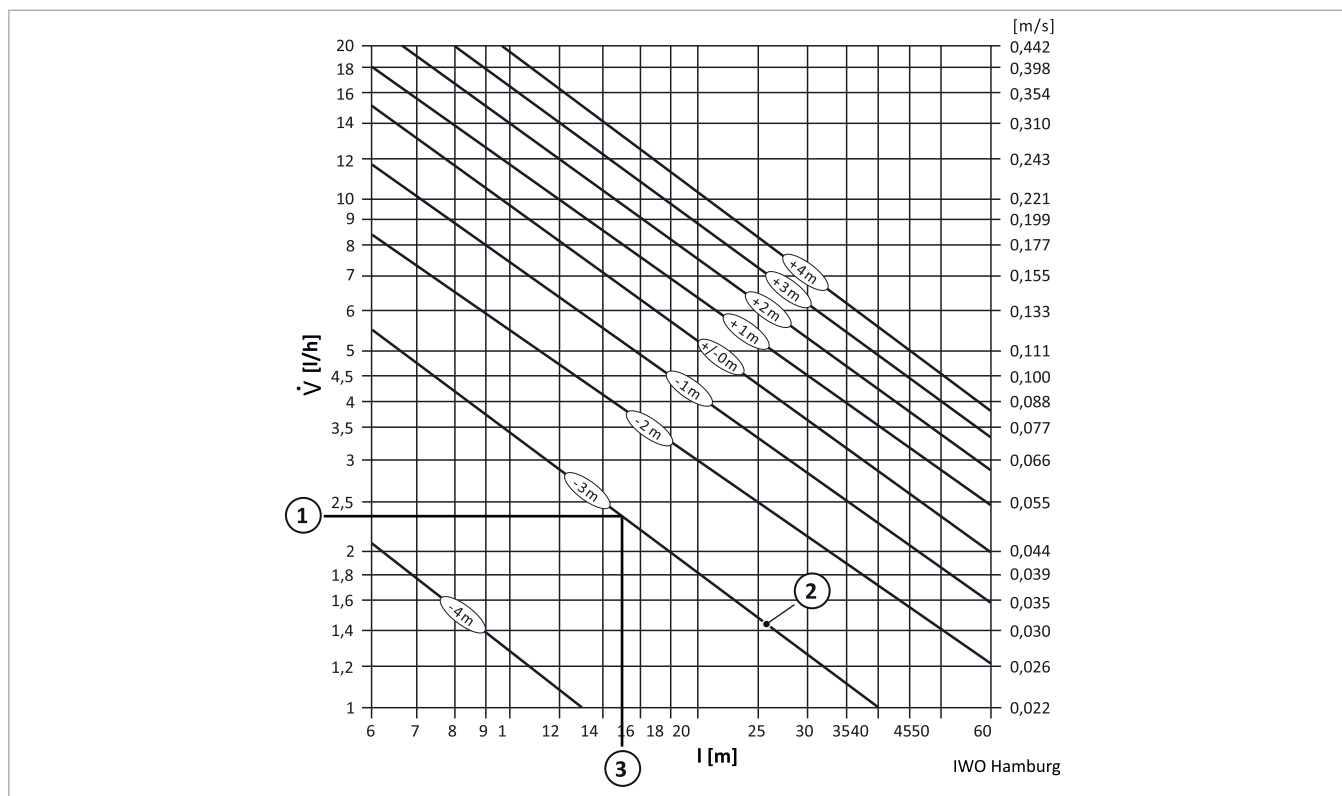
Afb. 24: Maximale leidinglengte in een één-leidingsysteem afhankelijk van de opvoerhoogte
