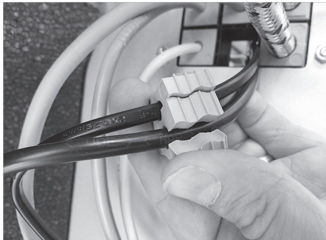
Fig. 13: Colocación del paso de cables alrededor del cable
