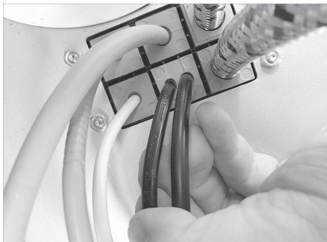
Fig. 14: Inserción del paso de cables en la abertura
