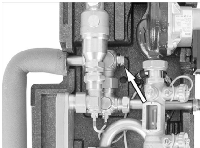
Fig. 17: Purgador de aire manual del lado secundario
