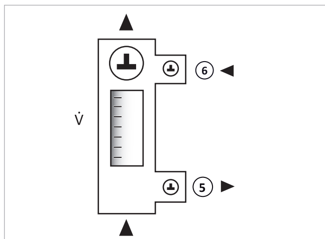
Fig. 20: Caudalímetro \dot{V} en posición de lavado 2
