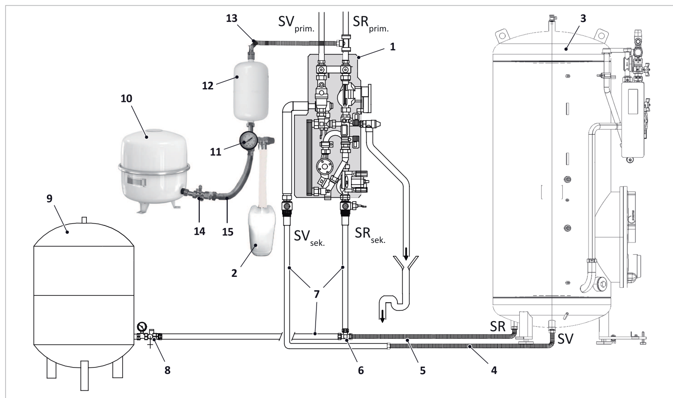
Fig. 2: Montaje de SUES-5.5, SOL-MAG y H-MAG en SolvisBen
