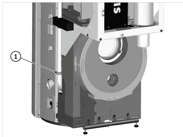
Fig. 25: controllare/serrare il raccordo a vite del ritorno
