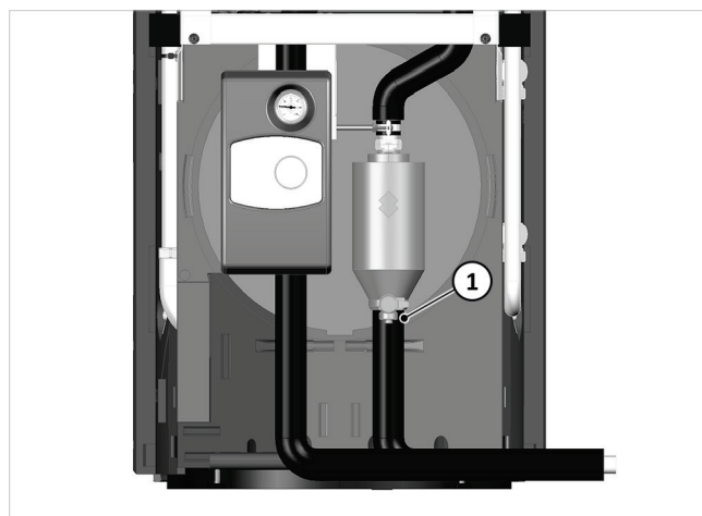
Fig. 82: pulizia del separatore di fanghi tramite rubinetto di scarico
