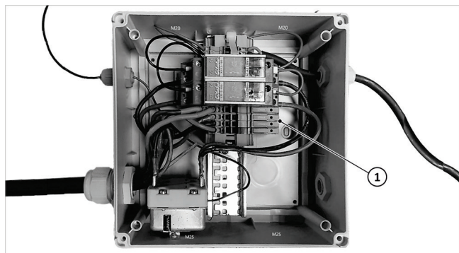
Fig. 54: Scatola di connessione
