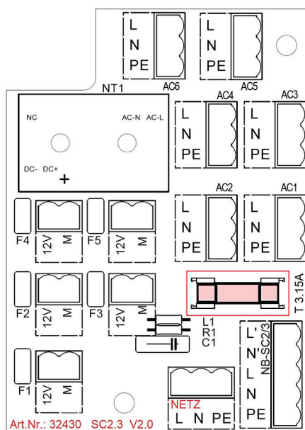
Fig. 100: Scheda di ampliamento per il gruppo di rete di SolvisControl 3
