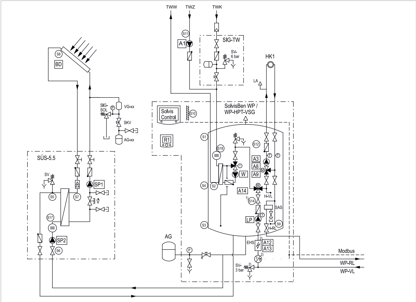
Fig. 88: SolvisBen WP con stazione circuito di riscaldamento integrata, impianto solare e pompa di calore SolvisLea, SolvisLea Eco o SolvisMia - Parte 1
