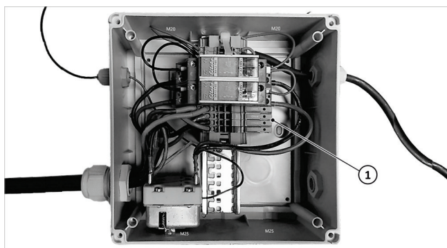
Fig. 54 : boîtier de raccordement
