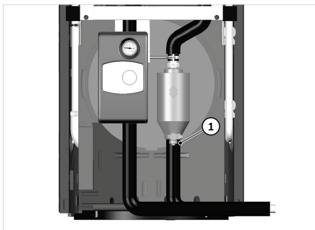
Fig. 80 : nettoyage du séparateur de boues au moyen du robinet de purge
