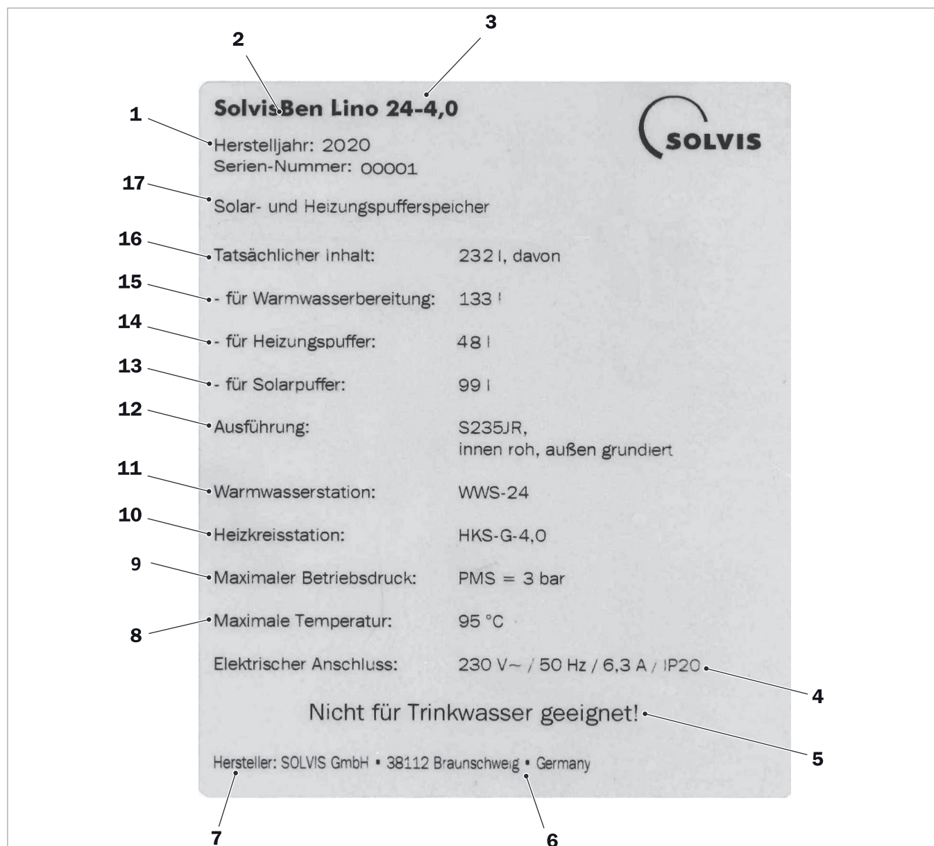
Fig. 103 : modèle de plaque signalétique de SolvisBen Lino
