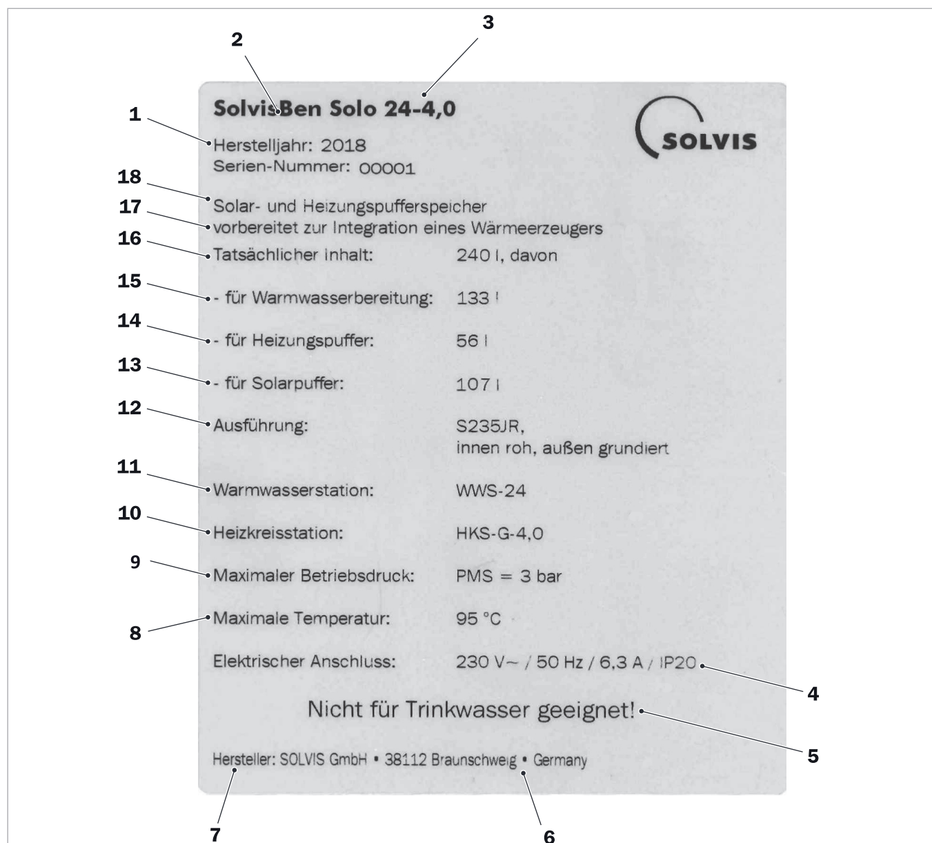
Fig. 104 : modèle de plaque signalétique de SolvisBen Solo
