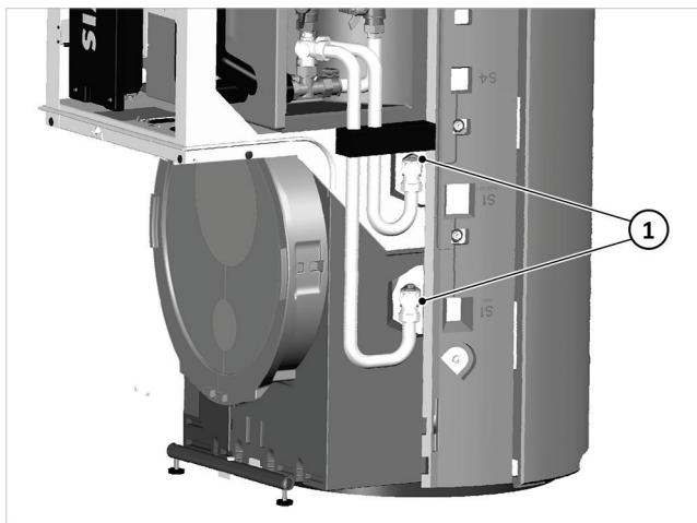
Fig. 30 : contrôler / resserrer les raccords de la station de chauffage
