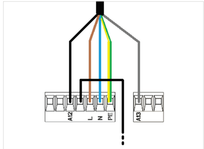
Fig. 53 : raccordement de SolvisLea
