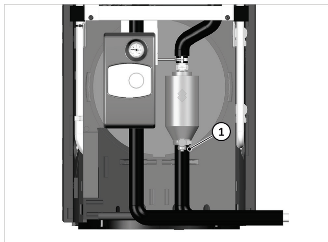
Afb. 82: Spuivoorziening en aftapkraan reinigen
