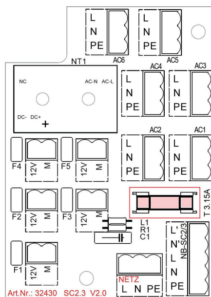
Afb. 100: Uitbreidingsprintplaat voor de netwerkaart van de SolvisControl 3
