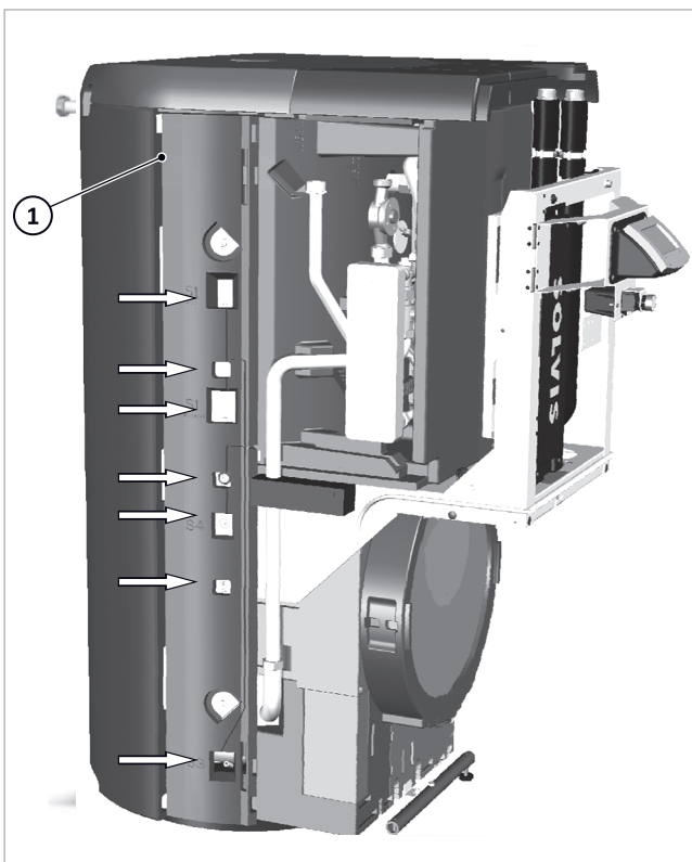
Afb. 74: Vliesstoppen linker kant (SolvisBen Solo)
