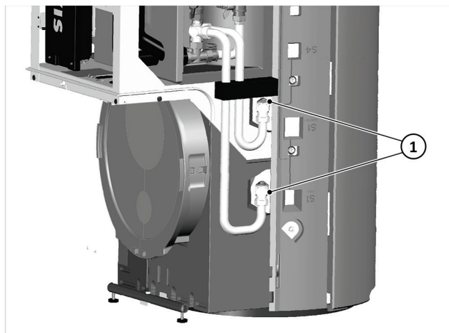
Afb. 30: De aansluitingen van de HKS controleren/vastdraaien
