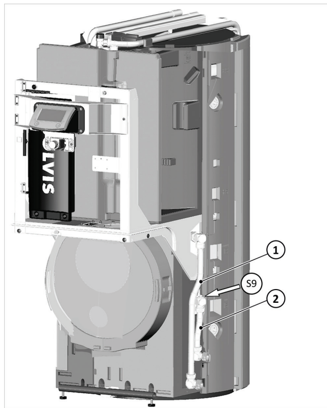
Afb. 35: H-VL (1)/H-RL-aansluiting (2) voor externe HKS
