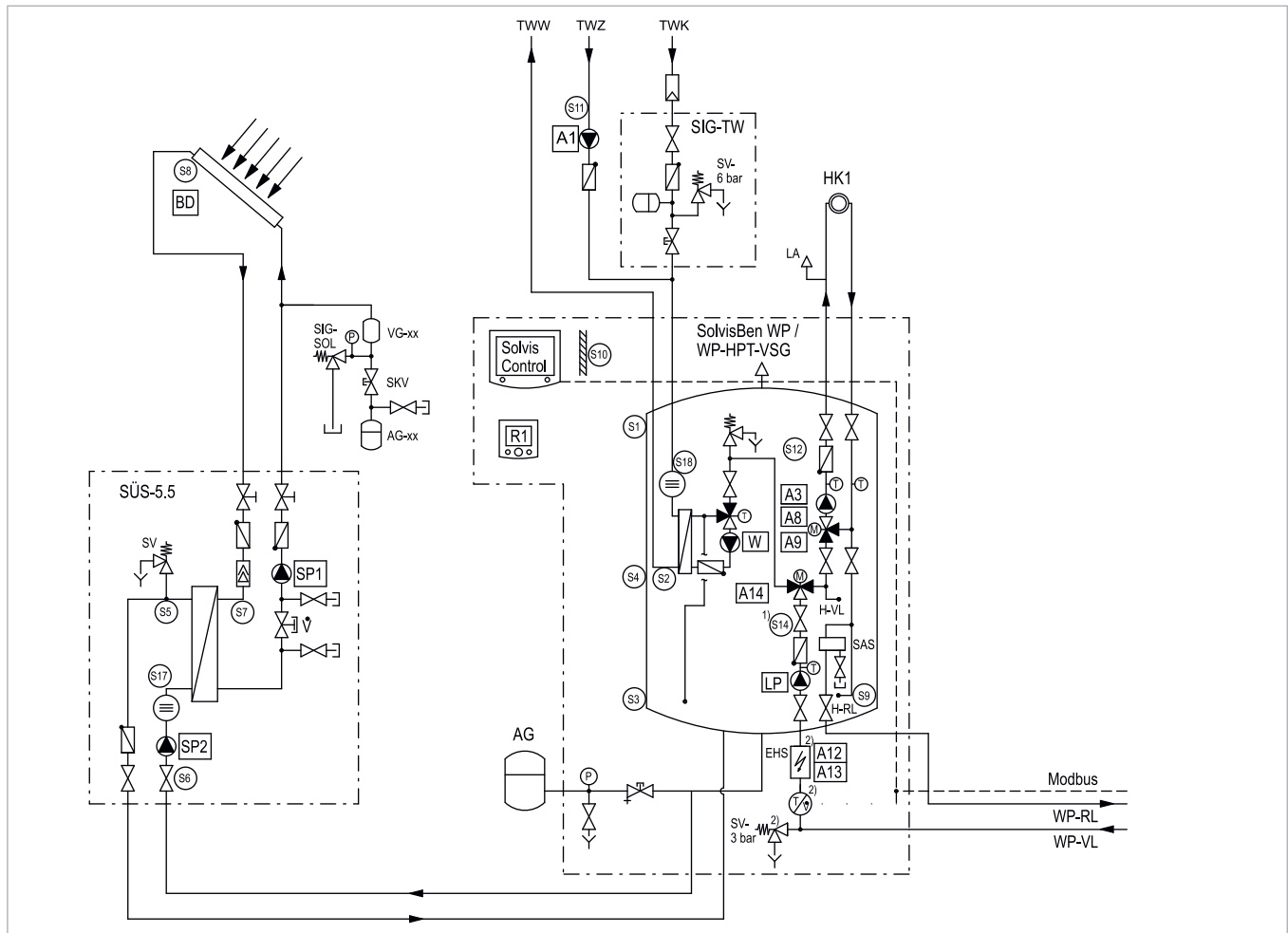
Afb. 88: SolvisBen WP met geïntegreerd verwarmingsgroepsstation, zonne-energiesysteem en warmtepomp SolvisLea, SolvisLea Eco of SolvisMia - deel 1
