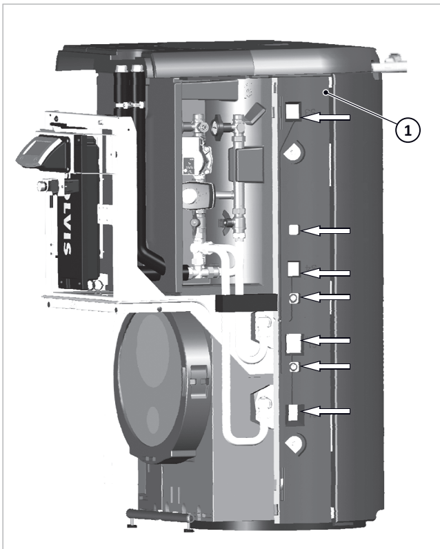
Afb. 73: Vliesstoppen rechter kant (Solvis Solo)
