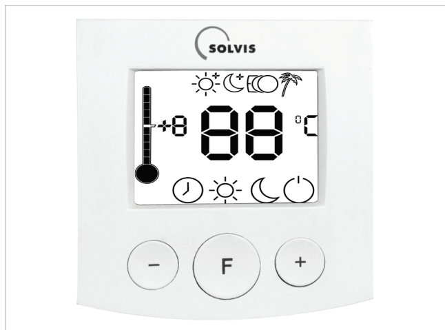
Afb. 49: Ruimtebedieningselement BE-SC-3
