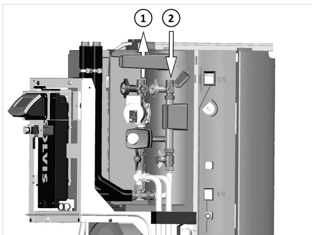
Afb. 32: H-VL/H-RL-aansluiting van bovenaf
