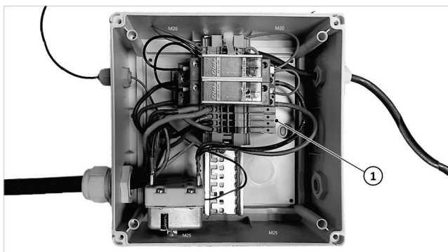
Afb. 54: Aansluitbox
