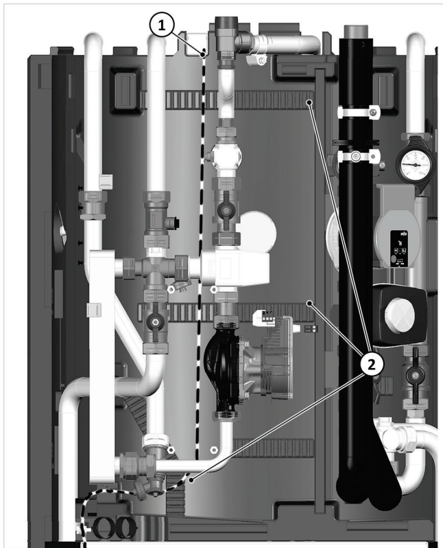
Afb. 45: Kabelgeleiding door de WWS-isolatie
