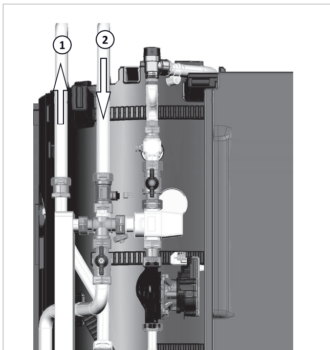
Afb. 27: TWW-/TWK-aansluiting van bovenaf
