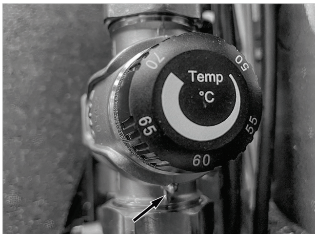
Afb. 60: Instelling TMV
