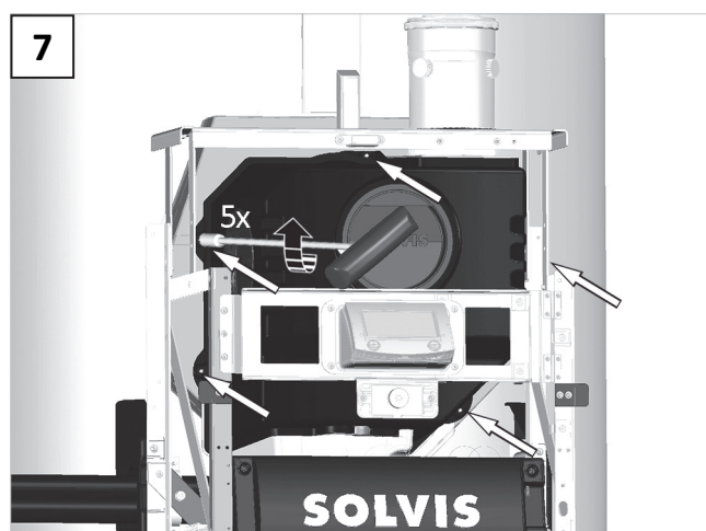
Abdeckung / Cover / Copertura / Cubierta / Cobertura / Couverture / Deksel
