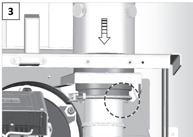
Abgasrohr / Exhaust pipe / Tubo di scarico / Tubo de escape / Tuyau d'échappement / Tubo de escape / Uitlaatpijp
