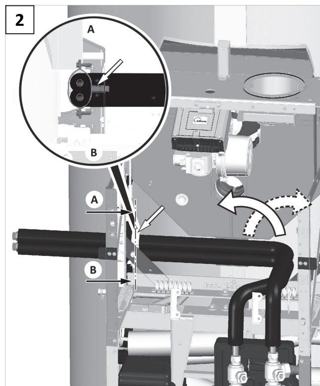
Solarleitungen (opt.) / Solar line (opt.) / Linea solare (optare.) / Línea solar (optar.) / Linha solar (optar.) / Ligne solaire (opter.) / Zonne-lijn (opt.)
