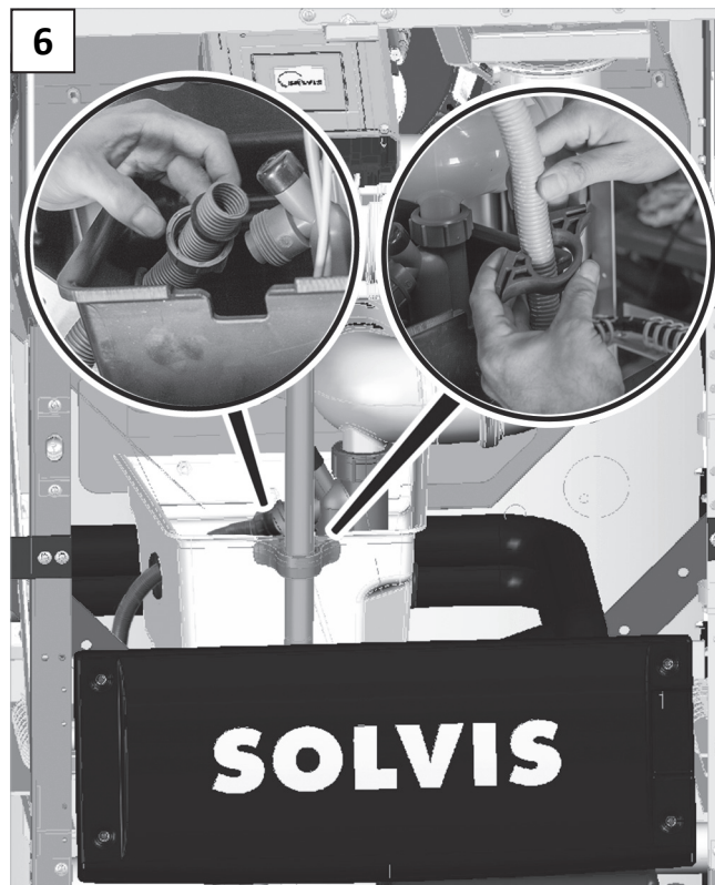
Leitungen / Lines / Linee / Las líneas / As condutas / Les conduites / Leidingen
