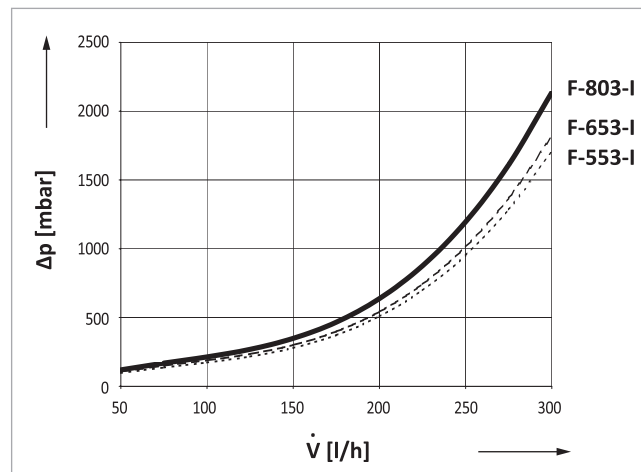
Fig. 74: Curva de pérdida de carga de SolvisFera Integral
