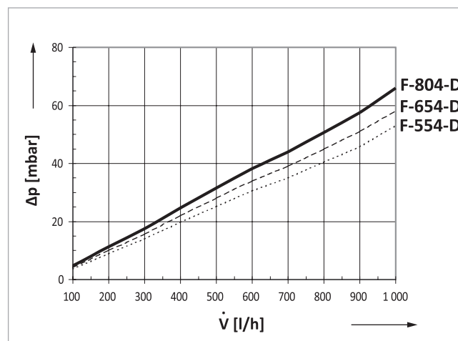
Fig. 75: Curva de pérdida de carga de SolvisFera Diagonal
