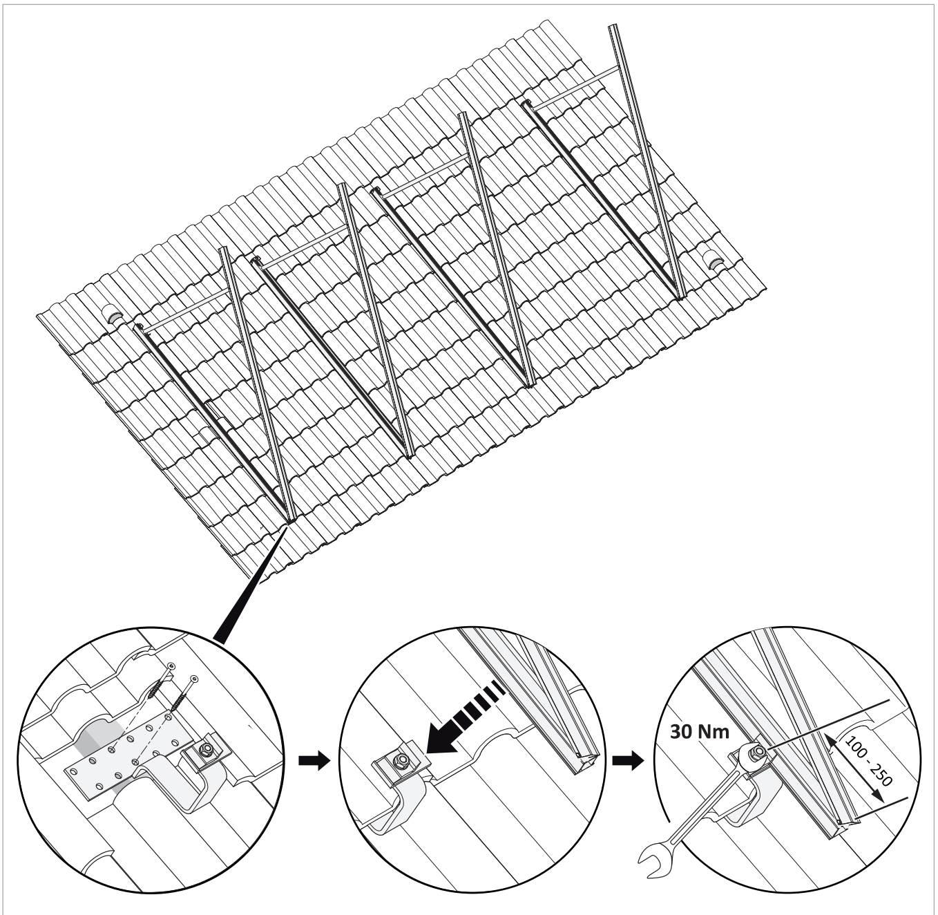
Fig. 29: Montaje del soporte para tejado plano en el soporte sobre tejado ADH-U
