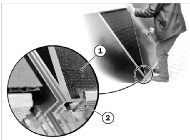
Fig. 33: Colocar las lunas
