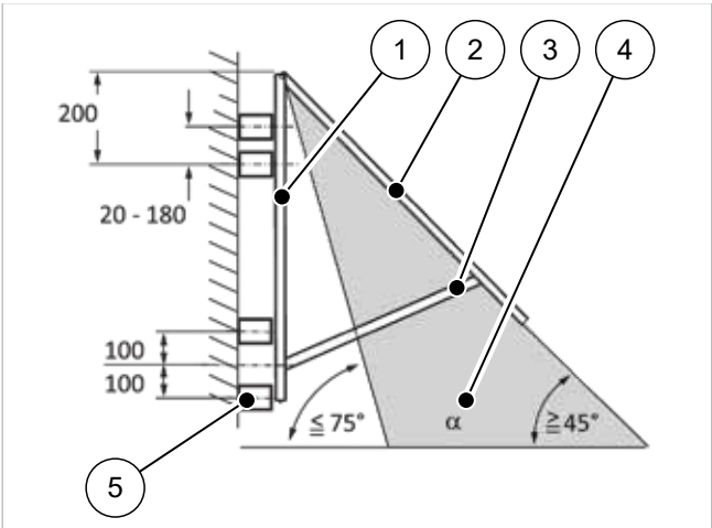
Fig. 24: Ensamblaje de los soportes en la pared
