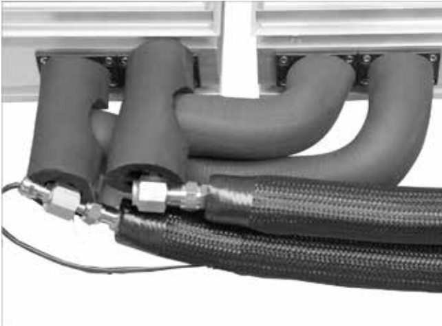
Afb. 49: SolvisFera Integral naast elkaar, aangesloten
