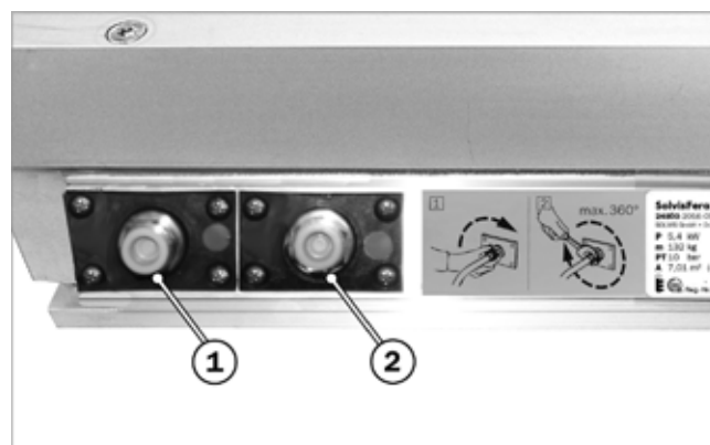
Afb. 40: Aanzicht collector, aansluitingen bovenaan (linkerkant)
