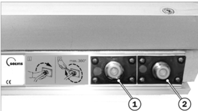
Afb. 43: Aansluiting buitenkant: Zonnesysteemaanvoer
