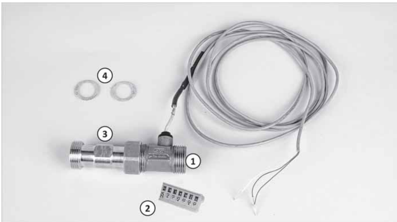
Abb. 1: Volumenstromgeber VSG-TW-SC-2
