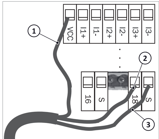
Abb. 4: Anschluss an Netzbaugruppe
