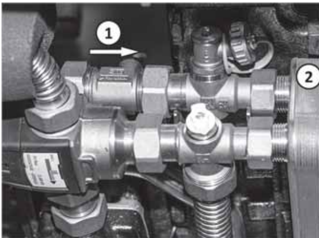
Abb. 3: VSG einbauen, hier WWS-24 in SolvisMax 7
