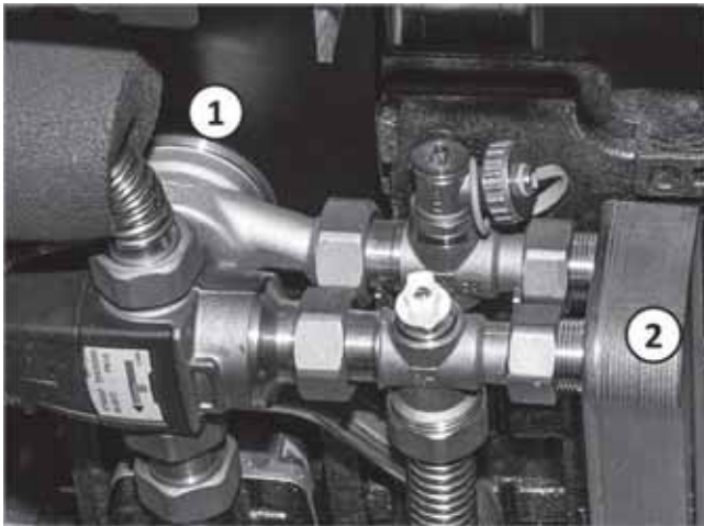
Abb. 2: VSG ausbauen, hier WWS-24 in SolvisMax 7
