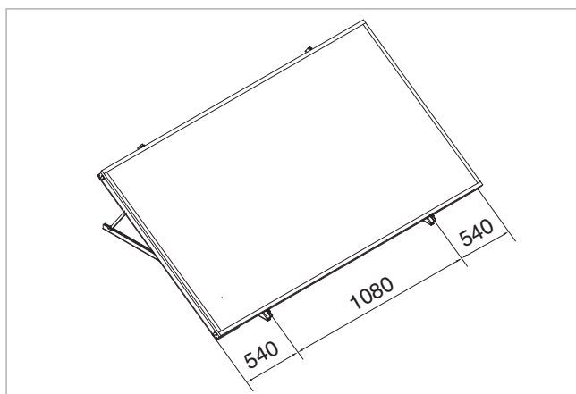
Abb. 62: Tussenafstanden collectorsteunen voor platte daken
