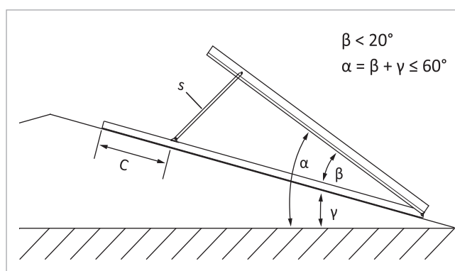
Fig. 37: Ángulo en superficies poco inclinadas
