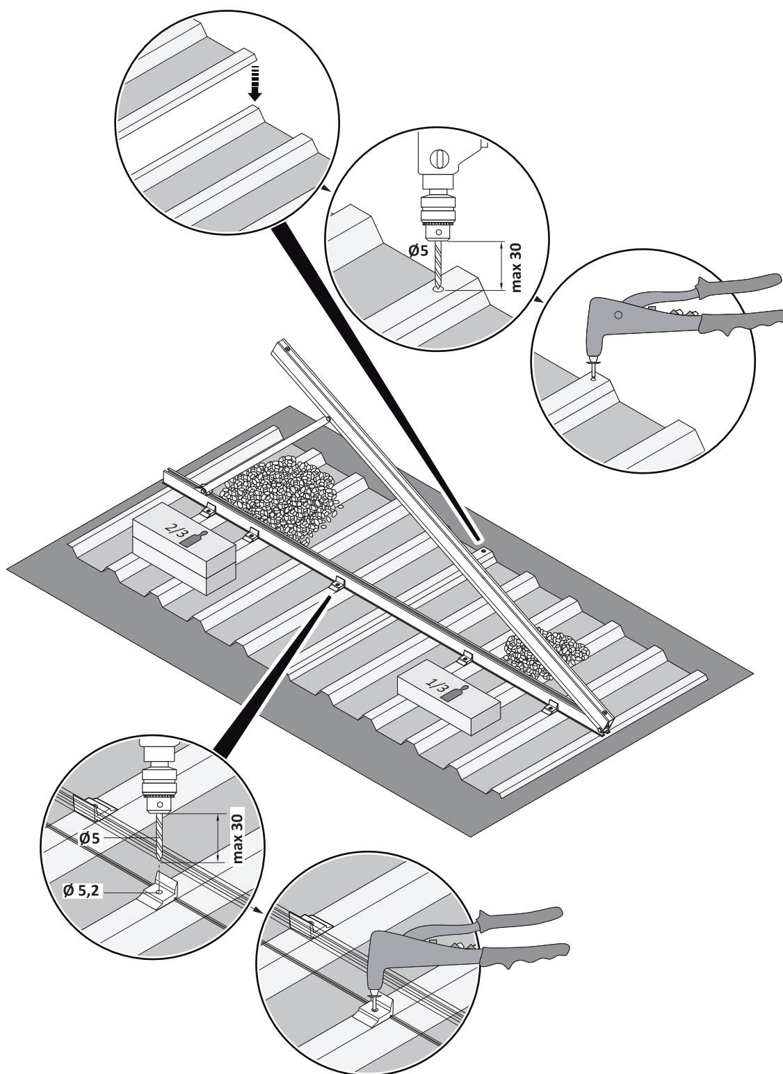
Fig. 42: Montaje del soporte para tejado plano en chapa trapezoidal
