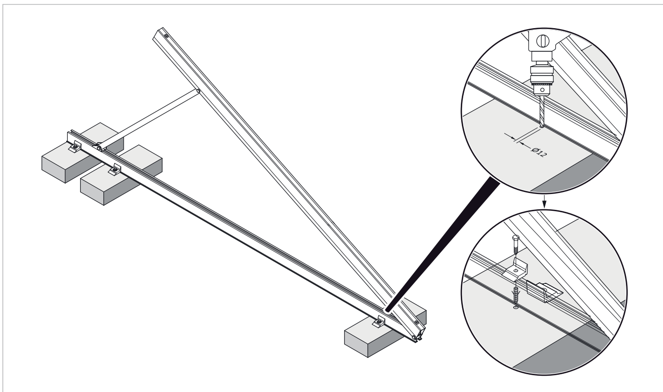
Fig. 55 : montage du montant pour toit plat sur bloc de béton
