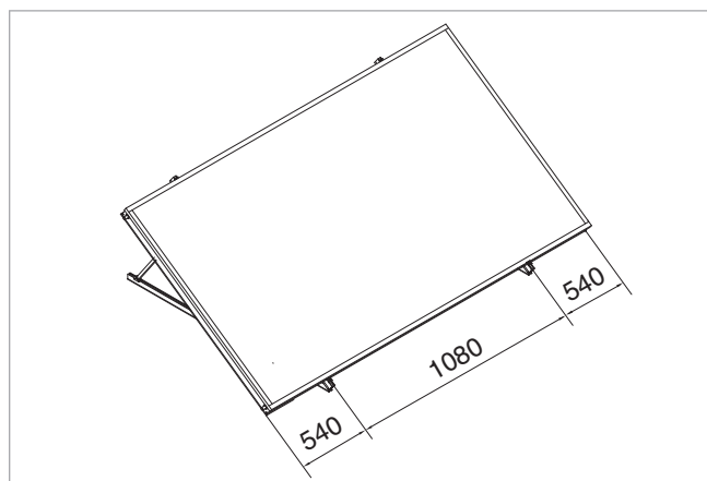
Abb. 20: Dimensoni delle distanze supporti per tetto piano
