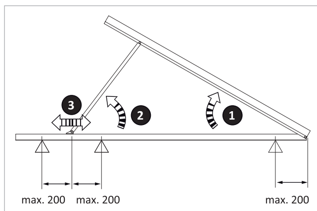
Fig. 36: Estructura del soporte para tejado plano
