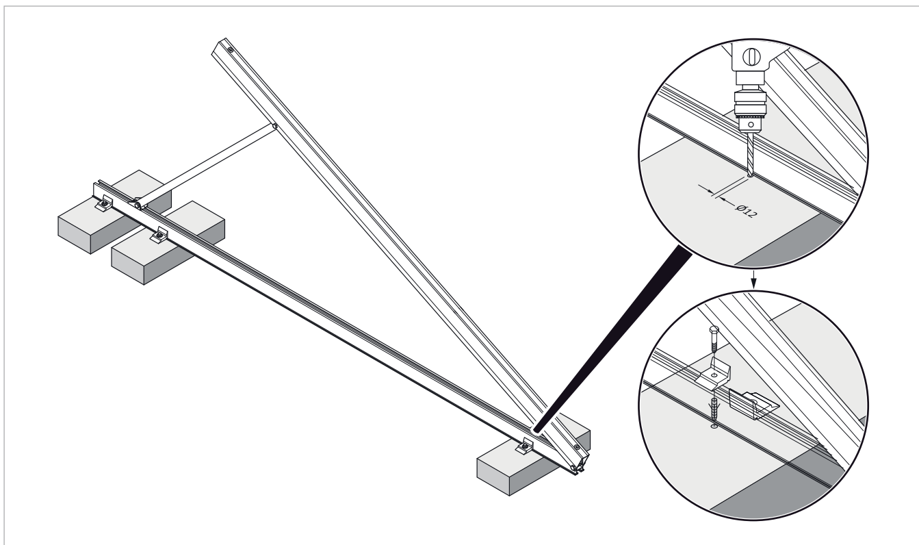
Afb. 69: Montage van de collectorsteunen voor platte daken op betonsteen
