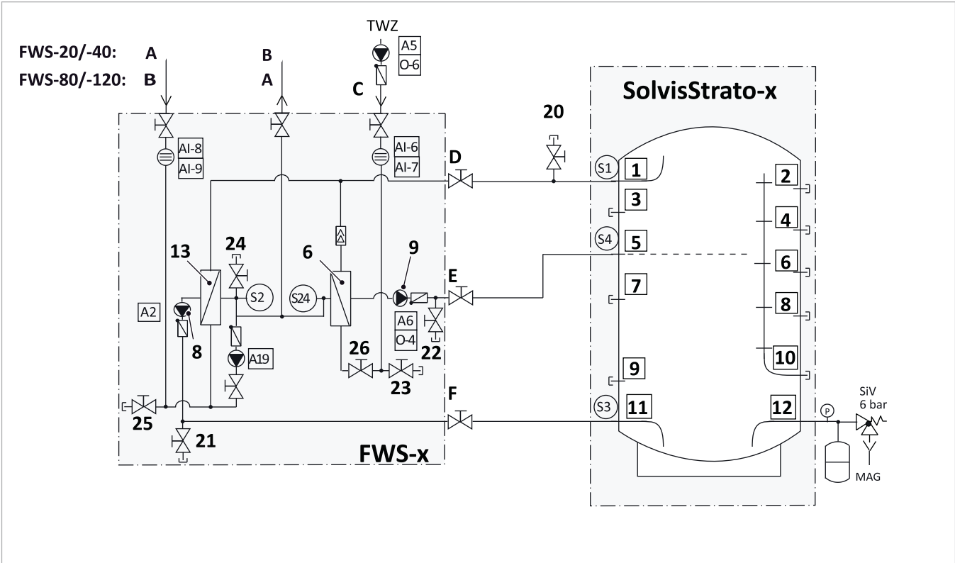
Afb. 6: Hydraulische aansluiting van het tapwaterstation (enkel-voorraadvat-systeem voor de tapwaterverwarming zonder aangesloten zonne-energiesysteem)
