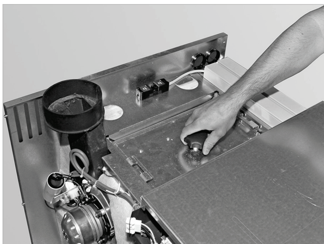
Abb. 18: Verschraubung entfernen
