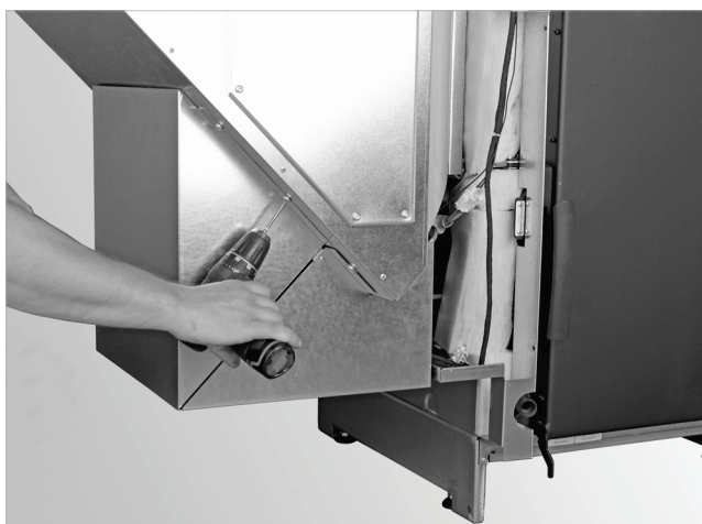
Abb. 67: Schrauben festziehen
