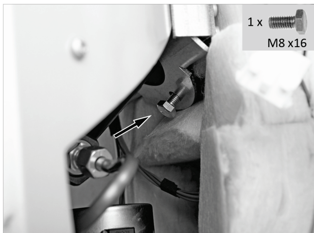
Abb. 59: Vorratsbehälter festschrauben
