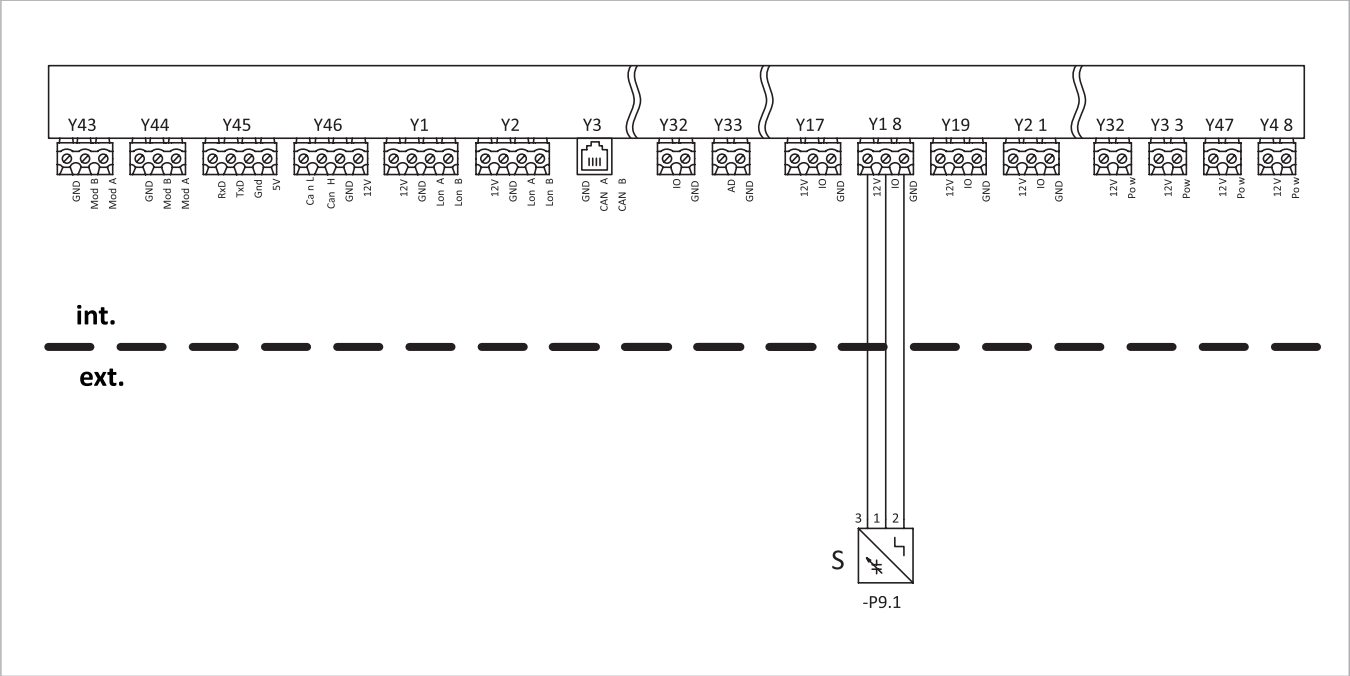
Abb. 192: Anschlussplan Absperreinheit
