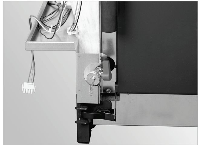
Abb. 27: Füll- und Entleerhahn eindrehen
