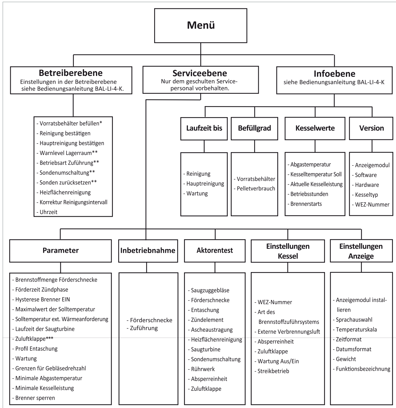
Abb. 119: Struktur in der Betreiber-, Service- und Infoebene
