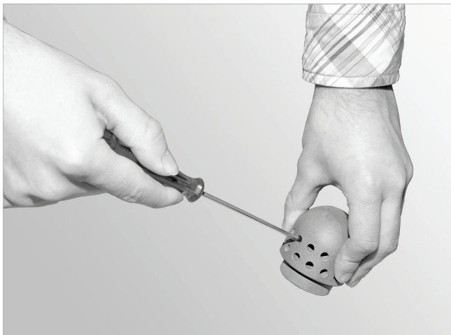
Abb. 150: Primärluftdorn vorsichtig reinigen
