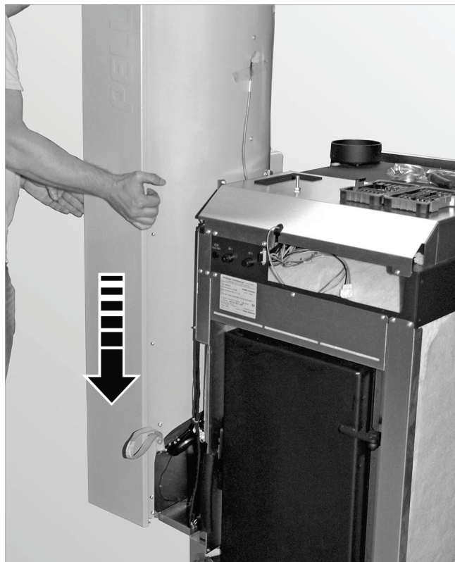
Abb. 169: Blende abnehmen (Bajonettverschluss)
