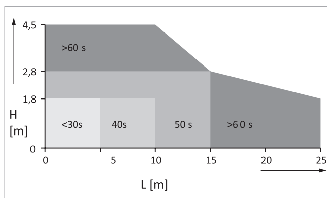
Abb. 120 Saugzeit nach Zuführschlauchlänge und Saughöhe
