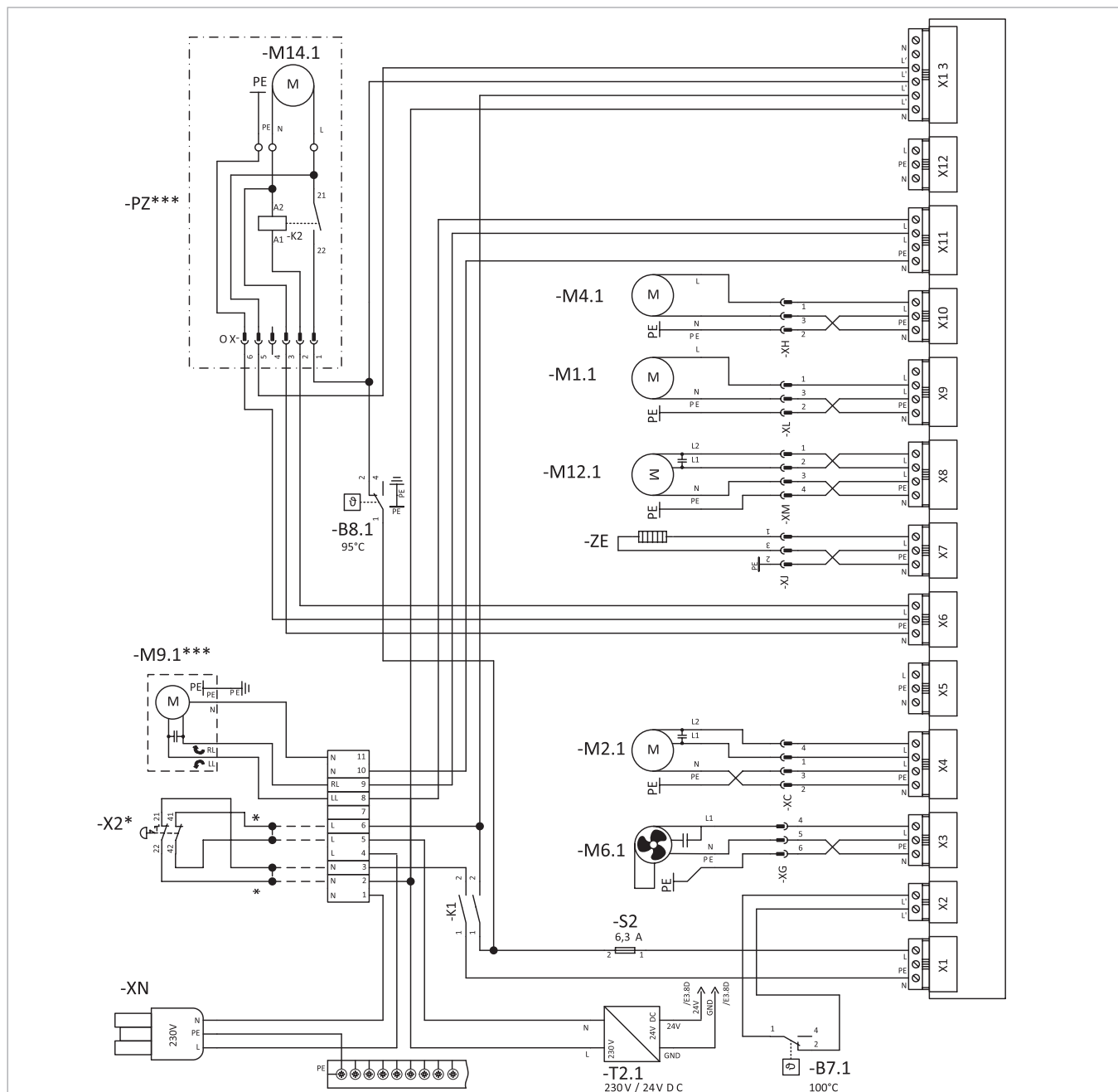
Abb. 185: Grundschahtbild SolvisLino 4 (Plan E1)
