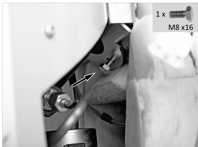
Abb. 33: Vorratsbehälter festschrauben
