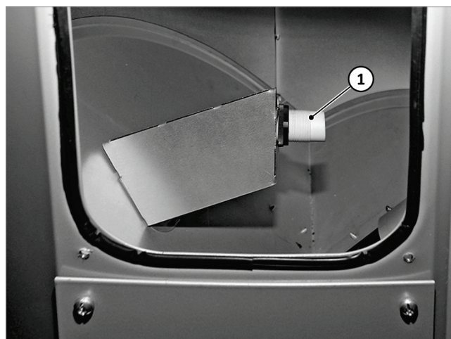
Abb. 172: Näherungsschalter reinigen
