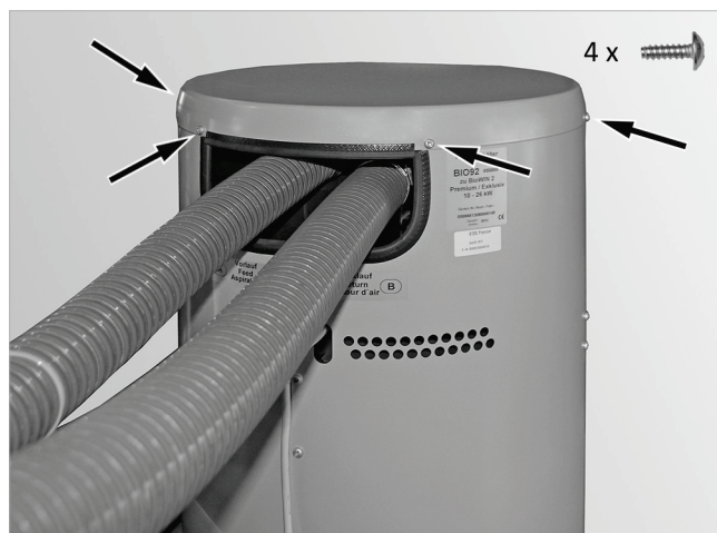
Abb. 105: Montage Förder- und Rückluftschlauch
