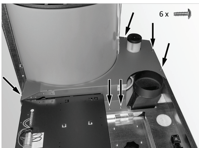
Abb. 77: Verkleidung befestigen
