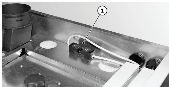
Abb. 166: Geräte-Netzstecker abziehen
