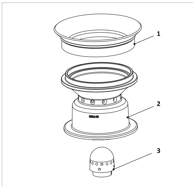
Abb. 153: Zusammenbau Brennertopf
