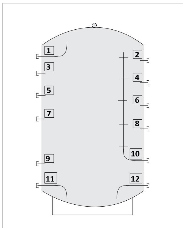
Fig. 25: Conexiones del acumulador intermedio de estratificación SolvisStrato 3
