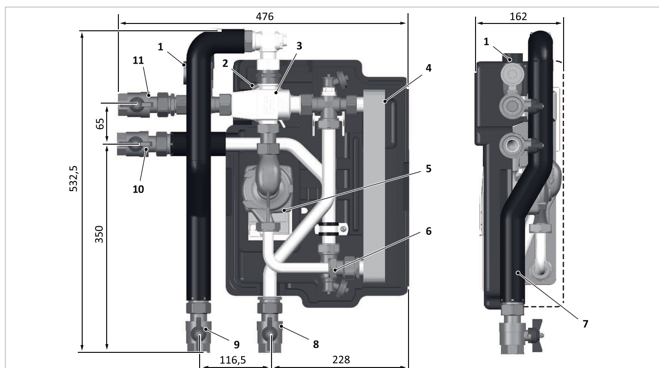
Fig. 31 : vue de la station d'eau chaude WWS-30-WM
