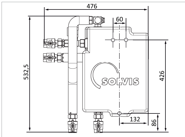
Afb. 42: Boorsjabloon WWS-30-WM (schaal 1: 10)
