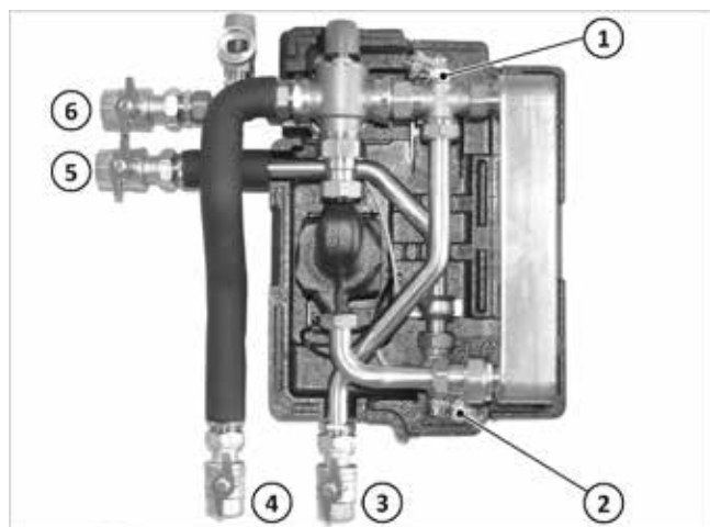
Afb. 48: Spoelen van de warmwater-warmtewisselaar
