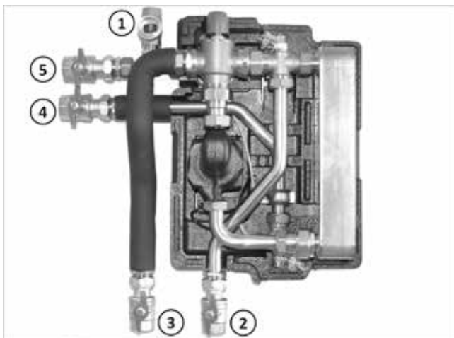
Afb. 44: Warmwatergroep ingehangen
