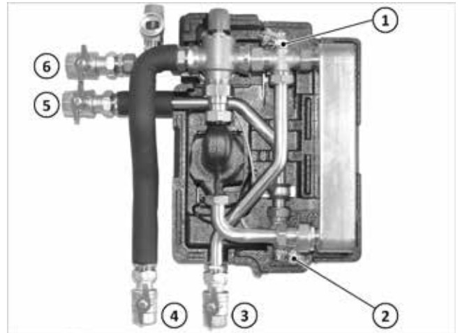
Fig. 38 : rinçage de l'échangeur thermique d'eau chaude
