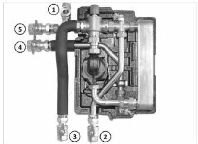
Fig. 34 : station d'eau chaude suspendue
