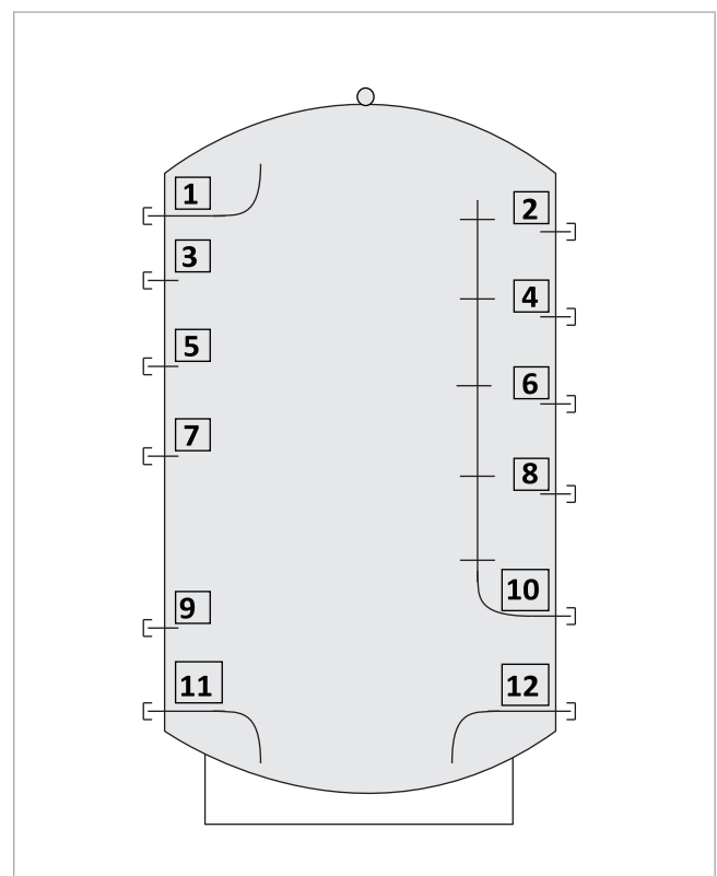
Afb. 45: aansluitingen gelaagd voorraadvat SolvisStrato 3
