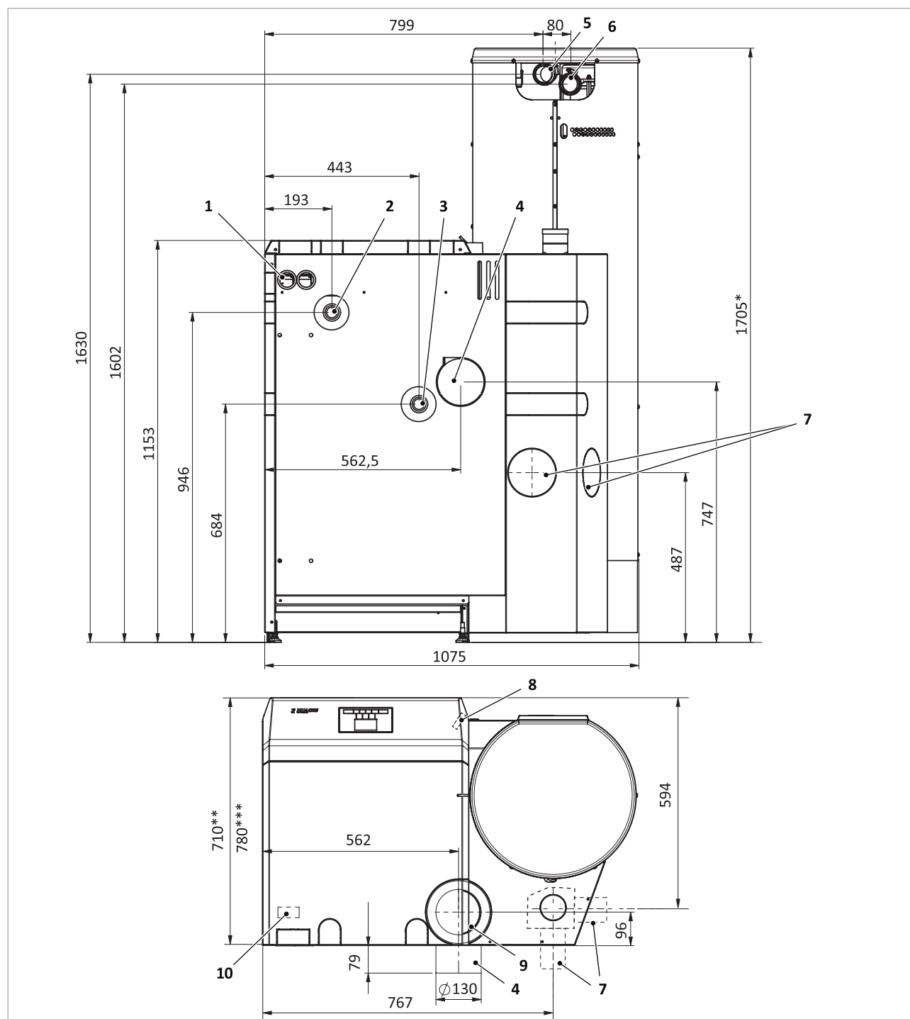
Abb. 20: Ansichten SolvisLino 4/5 mit Saugturbine (LI-4-xx-GS / LI-5-xx-GS)
