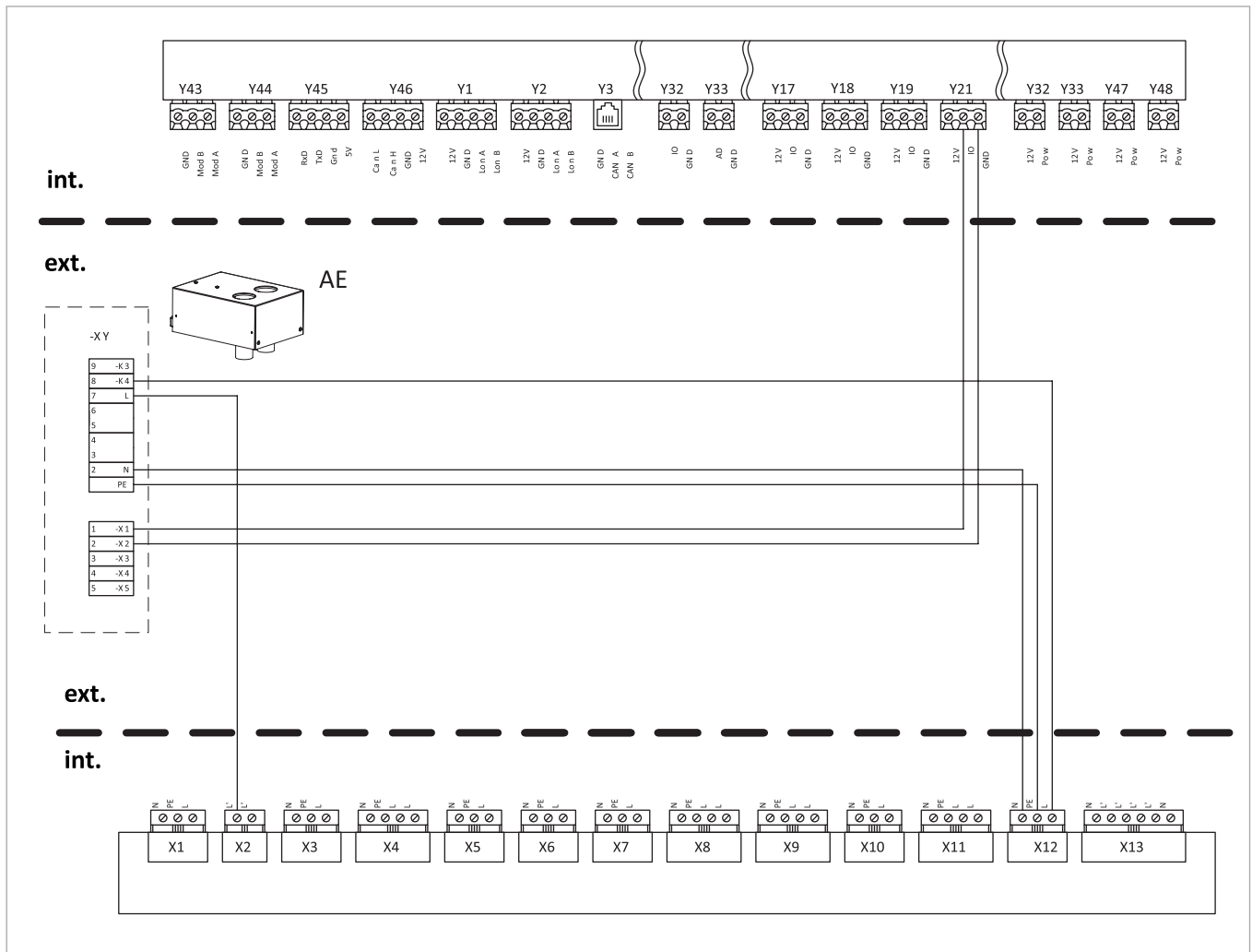
Abb. 18: Anschlussplan Absperreinheit
