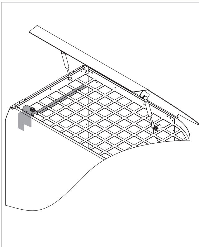
Abb. 15: Schalter montieren
