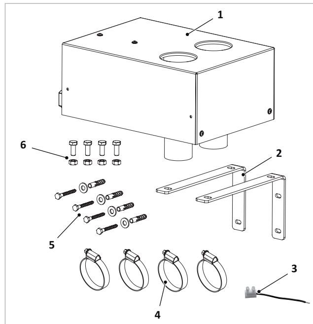
Abb. 4: Absperreinheit für externe Verbrennungsluftzuführung
