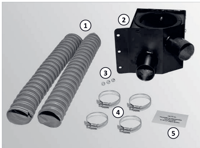
Abb. 3: Adapter für externe Verbrennungsluftzuführung
