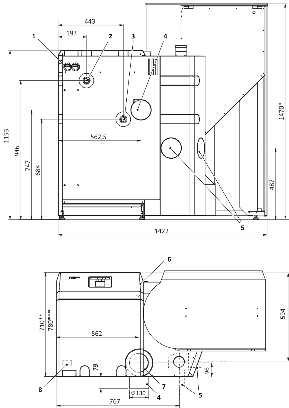
Abb. 21: Ansichten SolvisLino 4/5 mit Vorratsbeälter (LI-4-xx-VO / LI-5-xx-VO)
