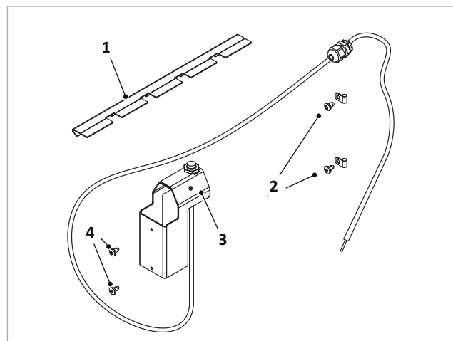
Abb. 6: Schalter Deckel Vorratsbehälter
