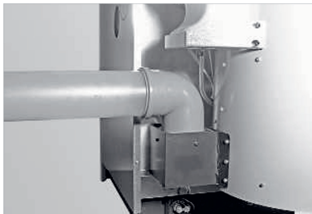
Abb. 10: Zuluftrohr montieren
