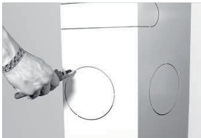
Abb. 11: Vorstanzung ausbrechen
