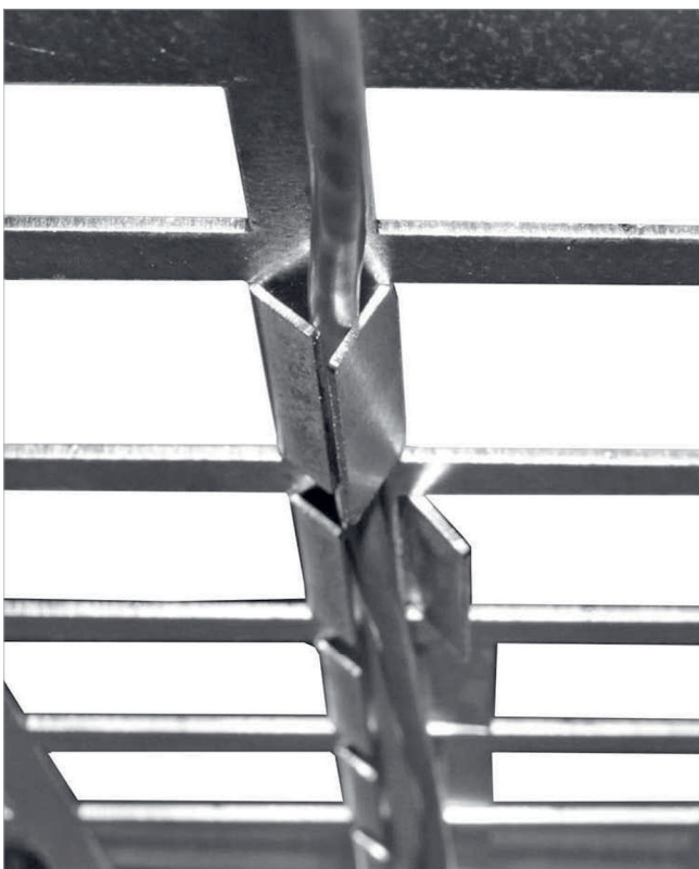
Abb. 16: Kabel unter Gitter verlegen
