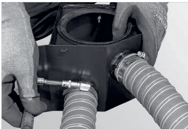
Abb. 7: Schläuche befestigen
