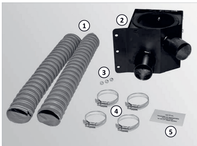
Abb. 5: Adapter für externe Verbrennungsluftzuführung
