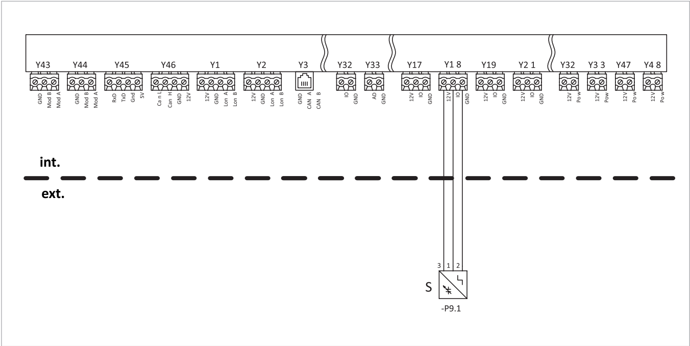
Abb. 19: Anschlussplan Absperreinheit
