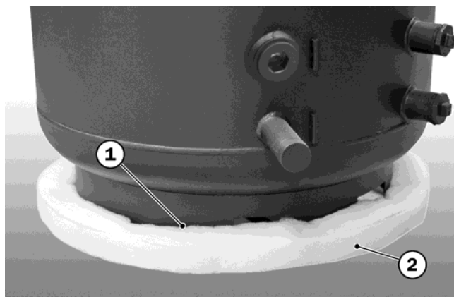
Afb. 6: isolatieschaal om de voet van de boiler plaatsen
