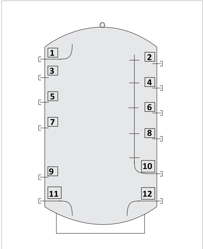
Afb. 13: aansluitingen gelaagd voorraadvat SolvisStrato 3
