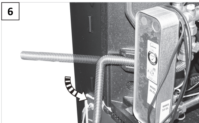
Biegen / Bending / Piegatura / Curvatura / Curvatura / Courber / Buigen
