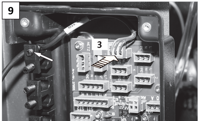
Aufstecken + Kabel sichern / Plug in + secure the cables / Inserire + fissare i cavi / Enchufar + asegurar los cables / Conecte + fixar os cabos / Brancher + fixer les câbles / Ansluiten + zet de kabels vast
