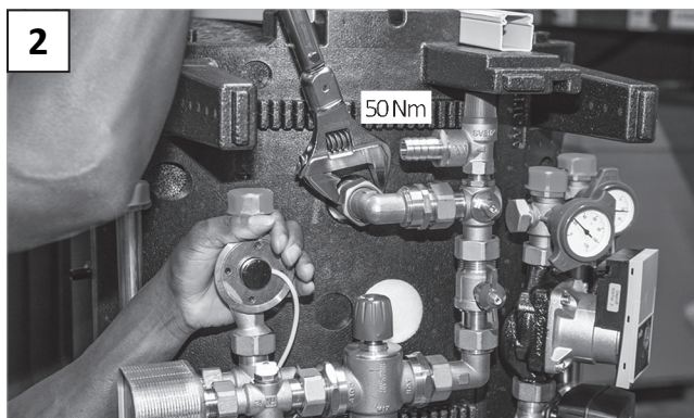
Festziehen / Tighten / Serrare / Apriete / Apertar / Serrer / Aanhalen
