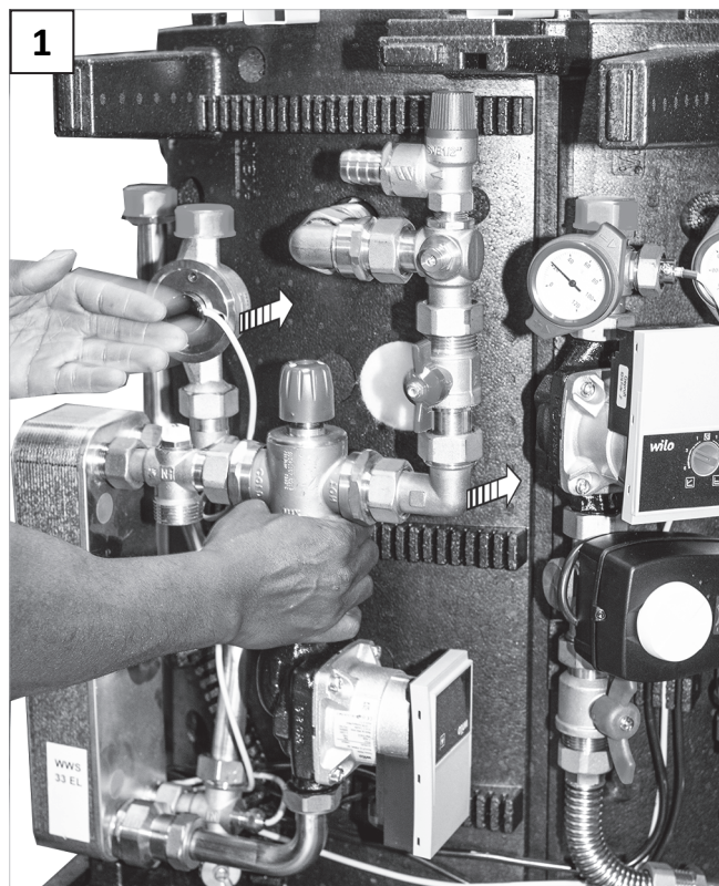
Einsetzen / Insert / Inserto / Insertar / Insérer / Inzetten
