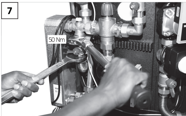
Gegenhalten! / Counter! / Contatore! / ¡Contador! / Contador! / Contre ! / Teller!
