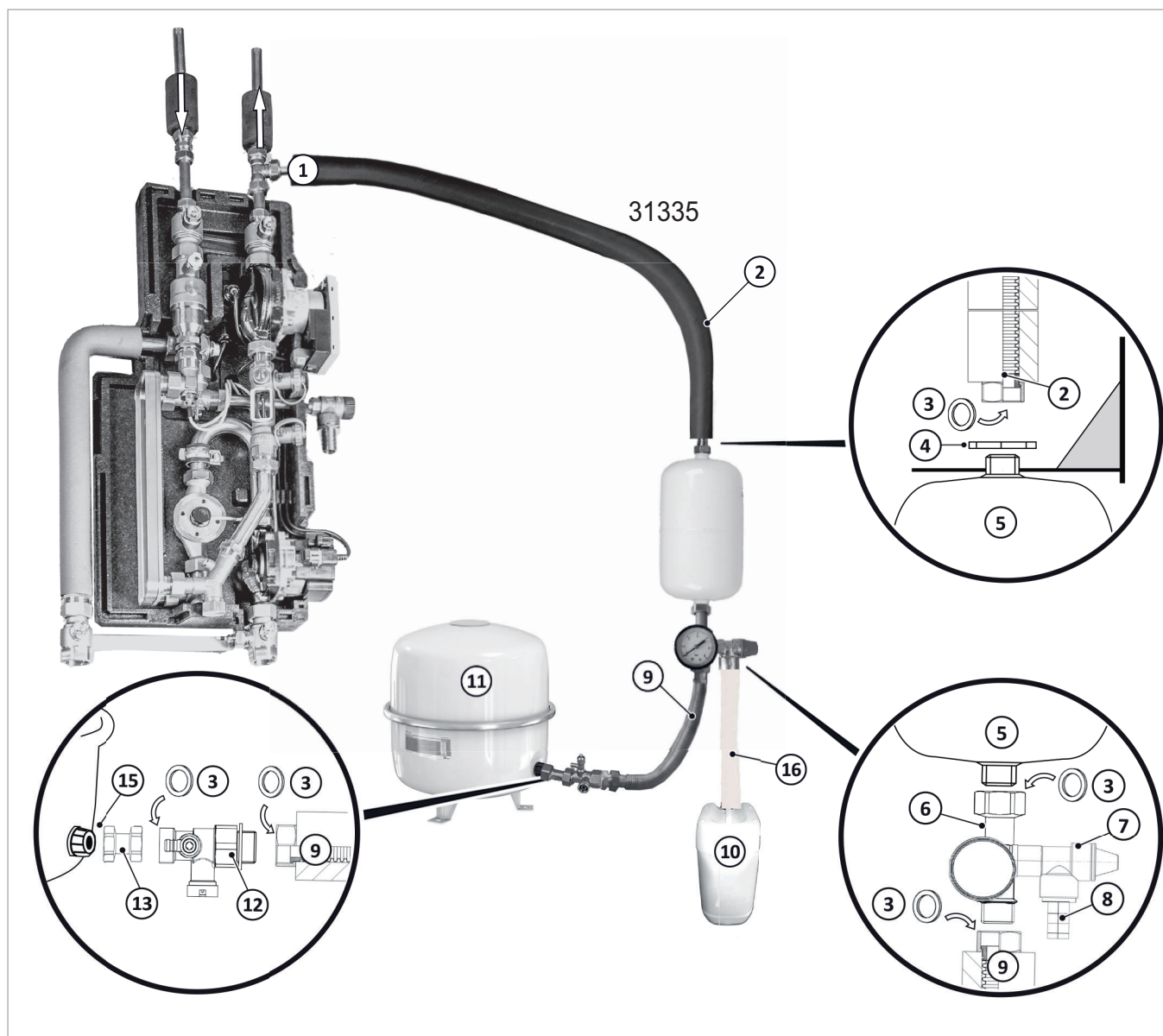
Fig. 2: Collegamento Solar-MAG
