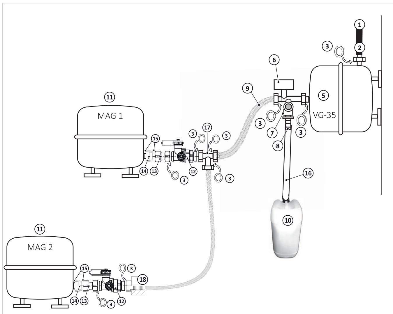
Fig. 8: raccordement du deux vases d'expansion à membrane solaire au moyen d'un kit d'extension d'un vase d'expansion (EW-AG)
