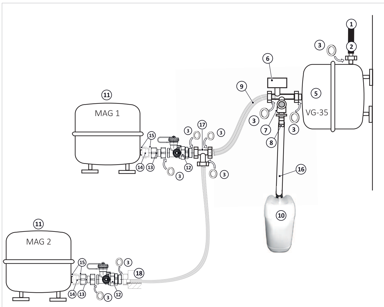
Fig. 4: Collegamento di due Solar-MAG per mezzo del vaso di espansione del set di estensione (EW-AG)
