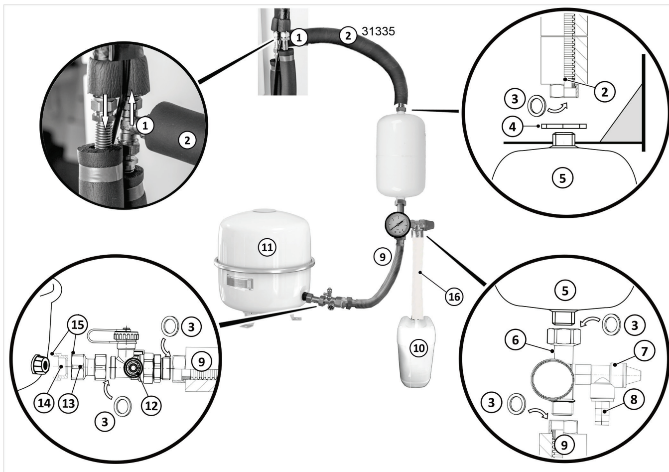
Afb. 9: Koppeling Solar-MAG
