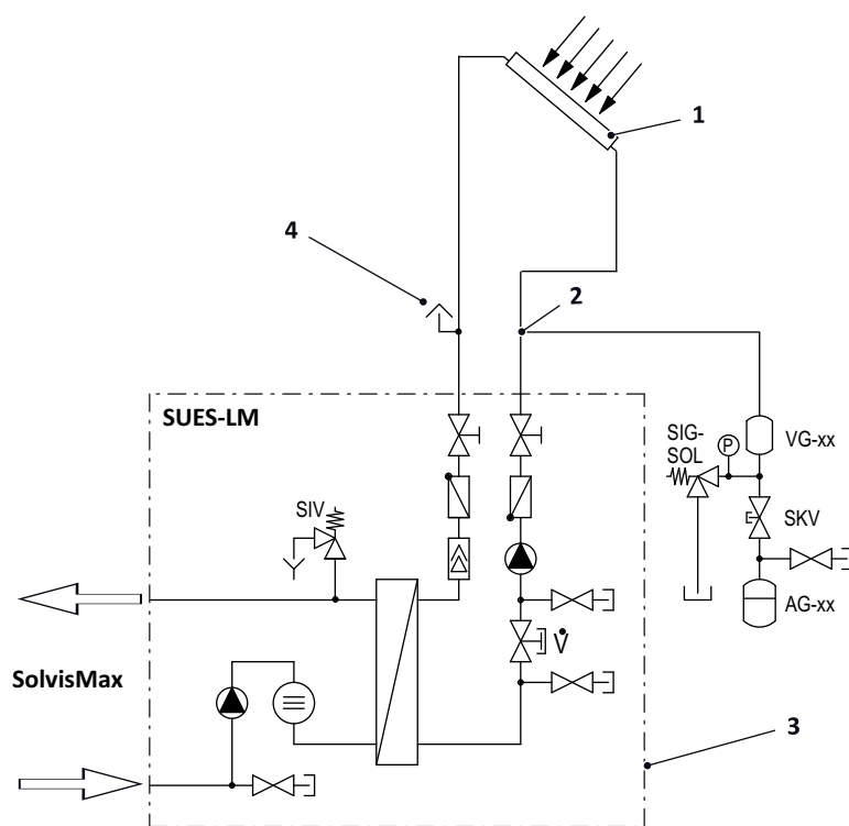
Abb. 1: Hydraulikschema Einbindung Luftabscheider
