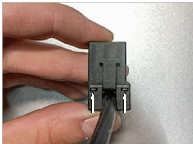
Abb. 4: Entriegeln / Unlocking / Sblocco / Desbloqueo / Déblocage / Ontgrendeling
