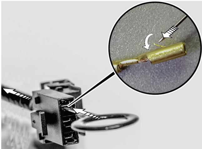
Abb. 6: Entriegeln / Unlocking / Sblocco / Desbloqueo / Déblocage / Ontgrendeling
