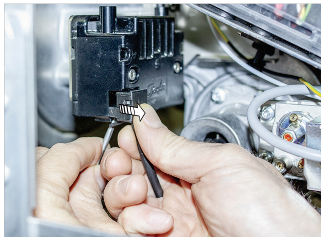
Abb. 3: Entriegeln / Unlocking / Sblocco / Desbloqueo / Déblocage / Ontgrendeling
