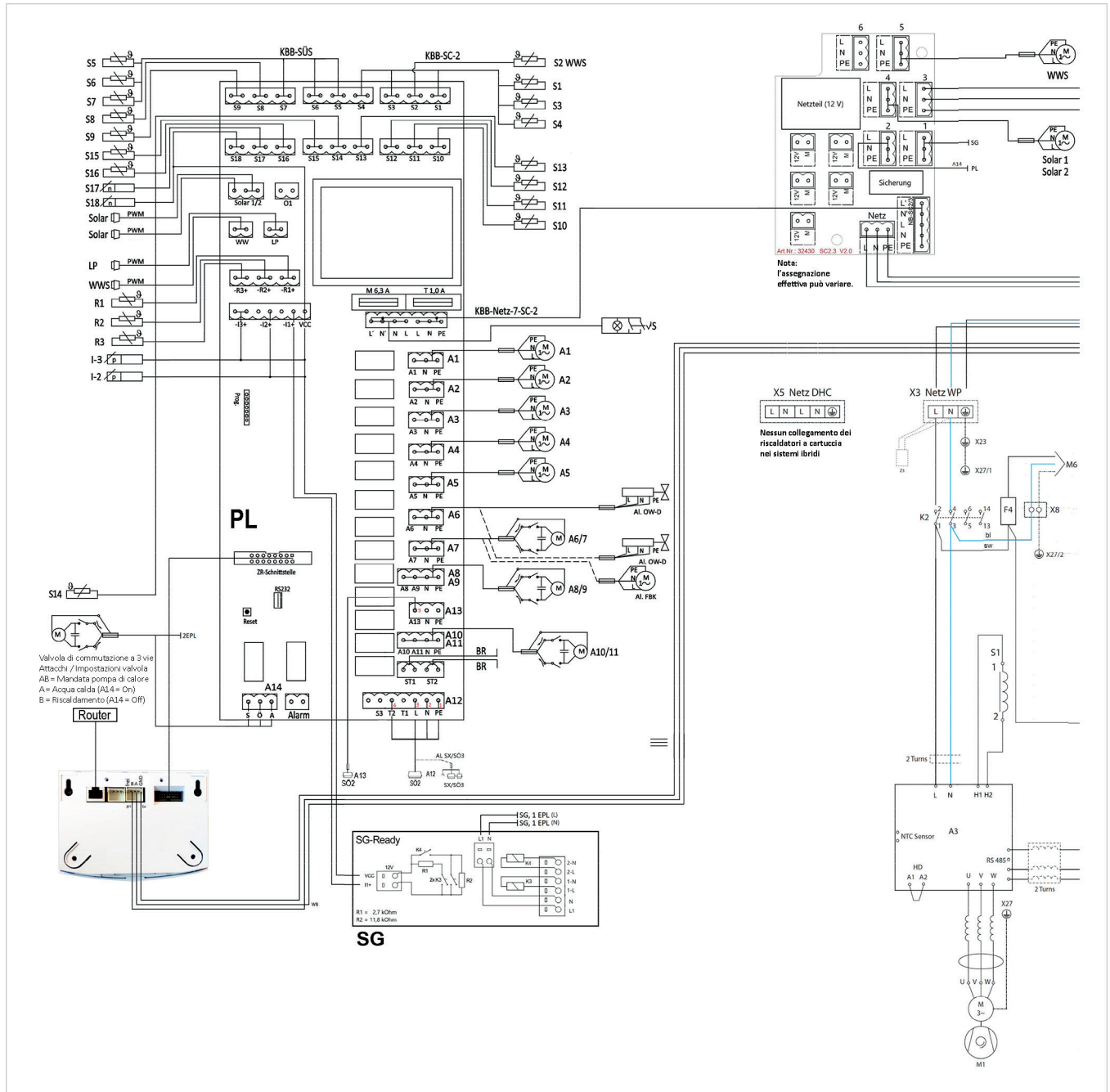
Fig. 45: Schema elettrico SolvisLea 7 kW sistema ibrido - Parte 1
