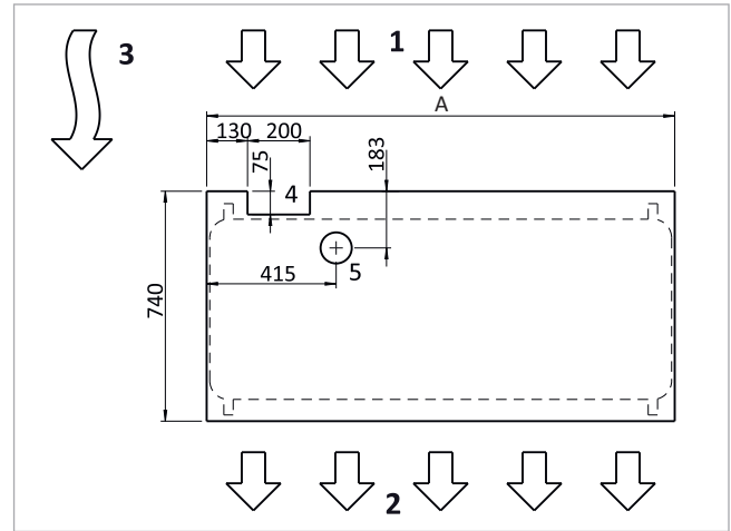
Fig. 6: Fondamenta per SolvisLea (vista dall'alto)
