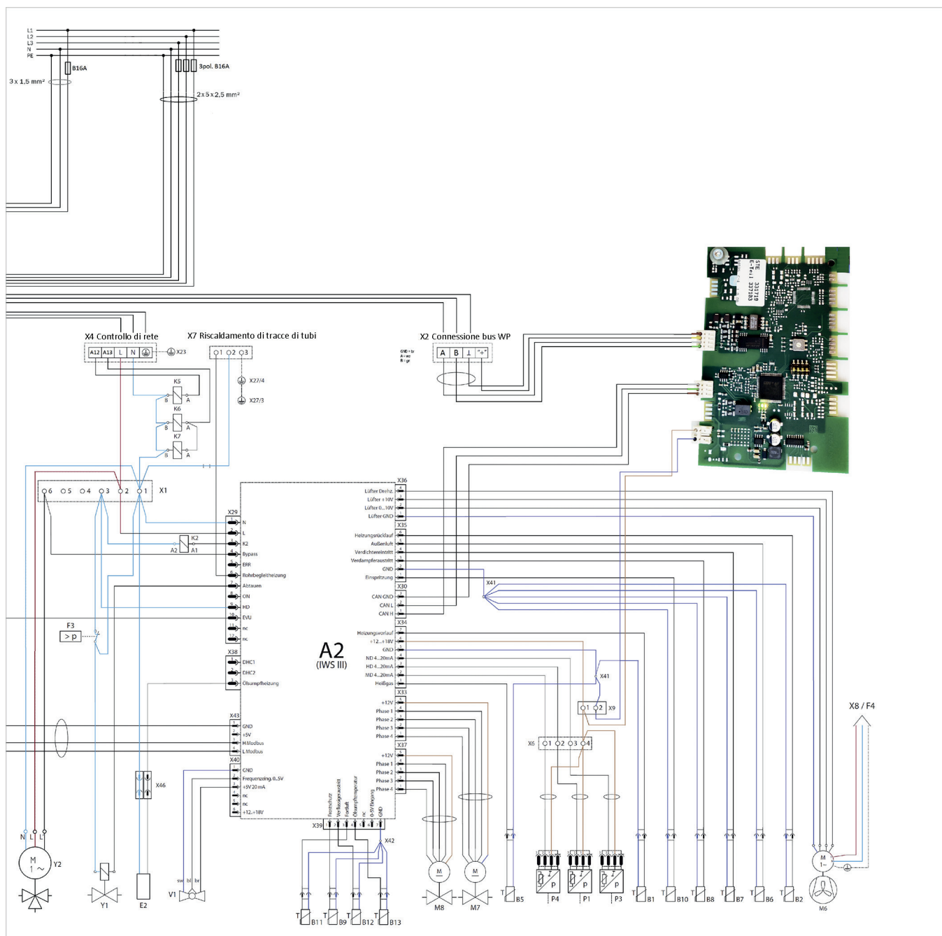
Fig. 50: Schema di flusso di corrente sistema ibrido SolvisLea 11 e 14 KW - Parte 2
