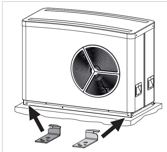
Fig. 10: Ancoraggio alle fondamenta
