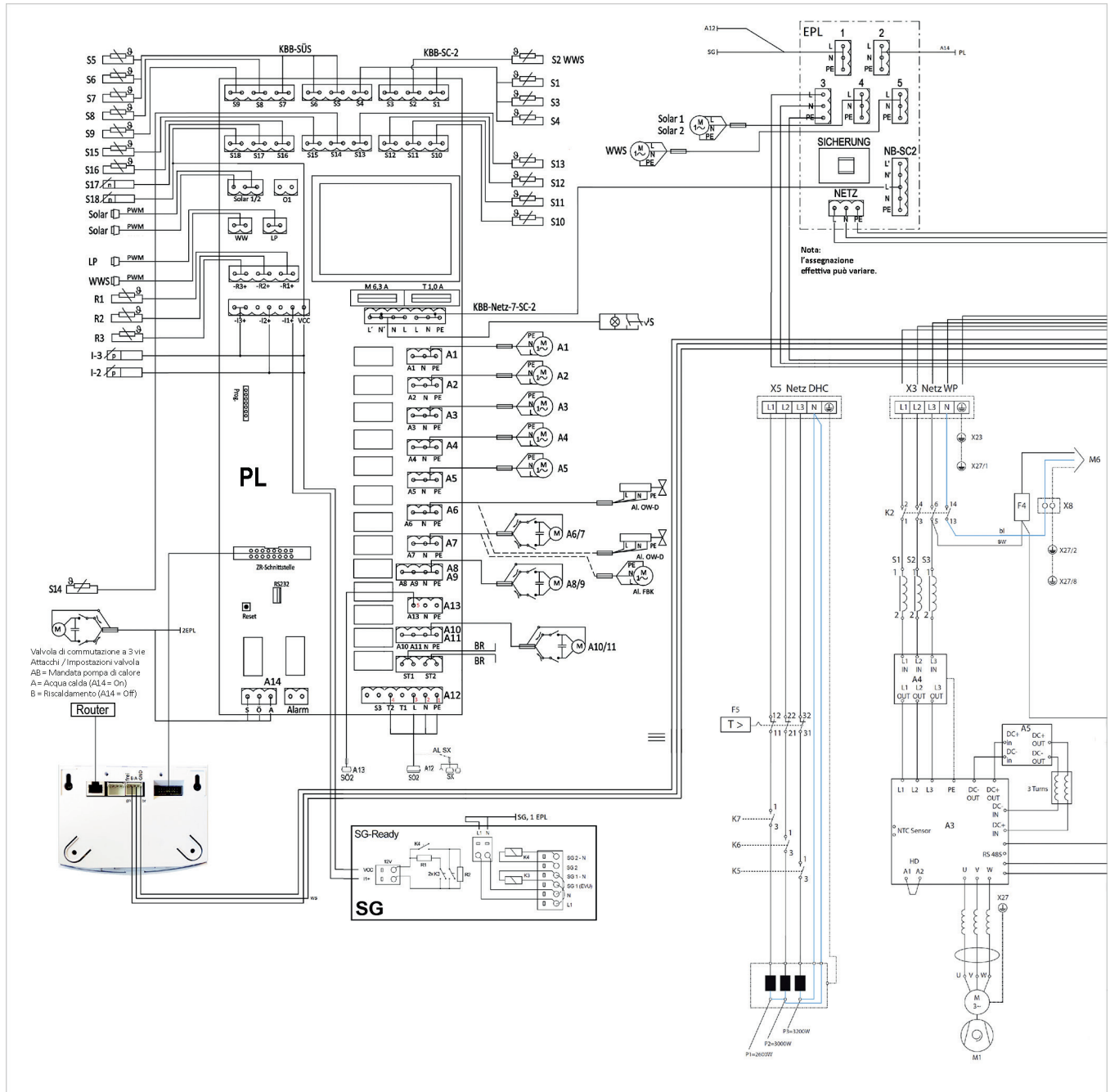
Fig. 49: Schema di flusso di corrente sistema ibrido SolvisLea 11 e 14 KW - Parte 1
