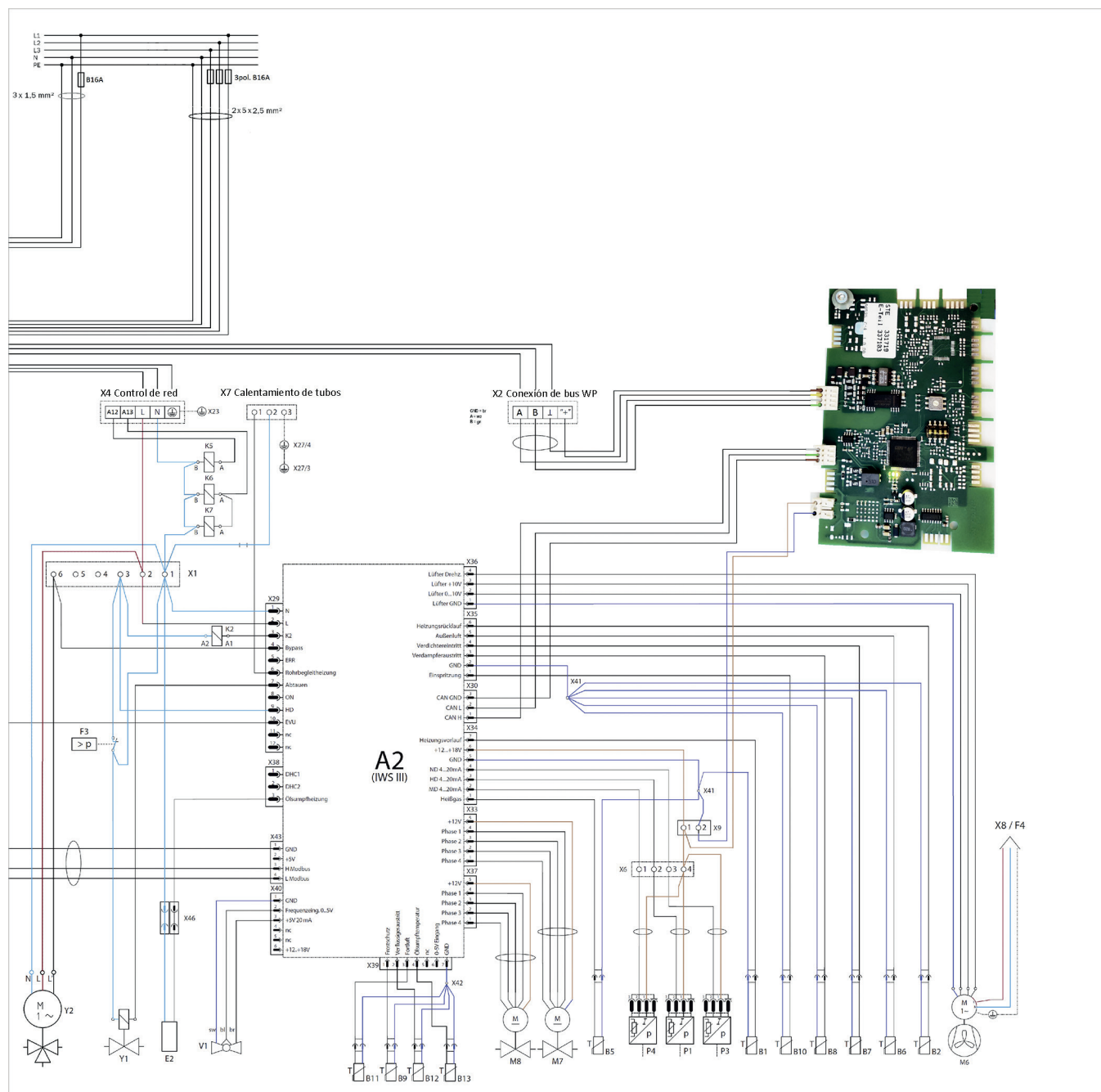
Fig. 50: Esquema de circuitos de SolvisLea 11 y 14 KW sistema híbrido - Parte 2
