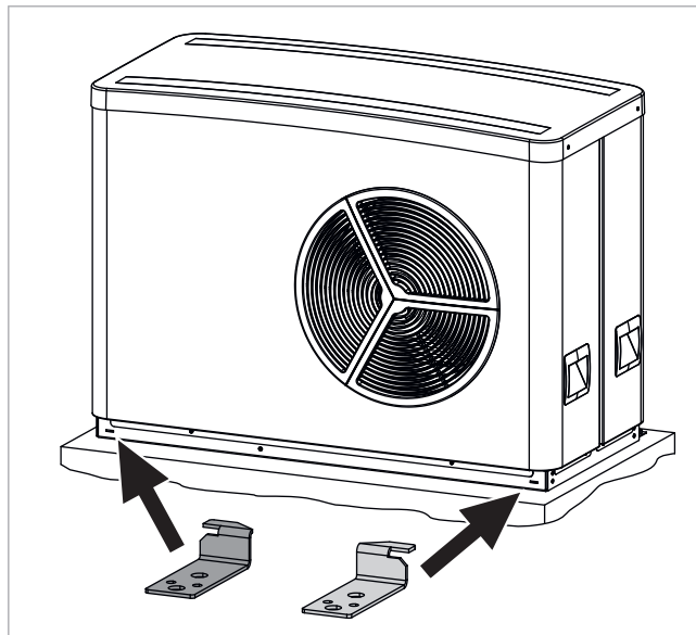
Fig. 10: Atornillado a los cimientos
