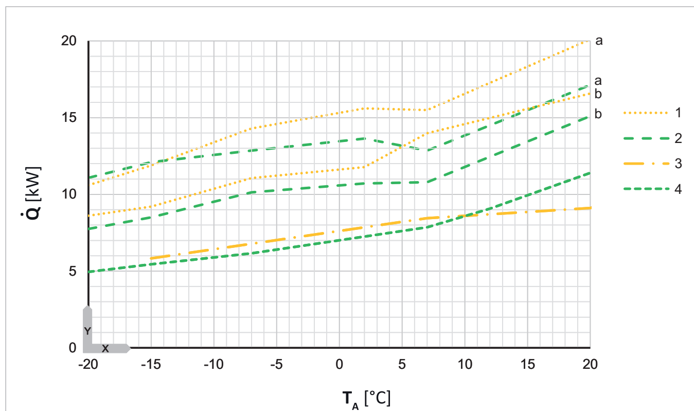
Fig. 41: Diagrama de datos de potencia de SolvisLea 11 y 14 kW
