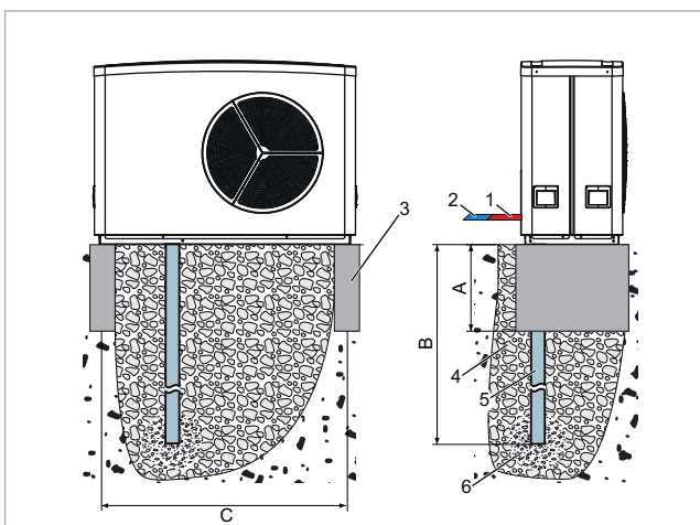
Fig. 13: SolvisLea montada en cimientos corridos
