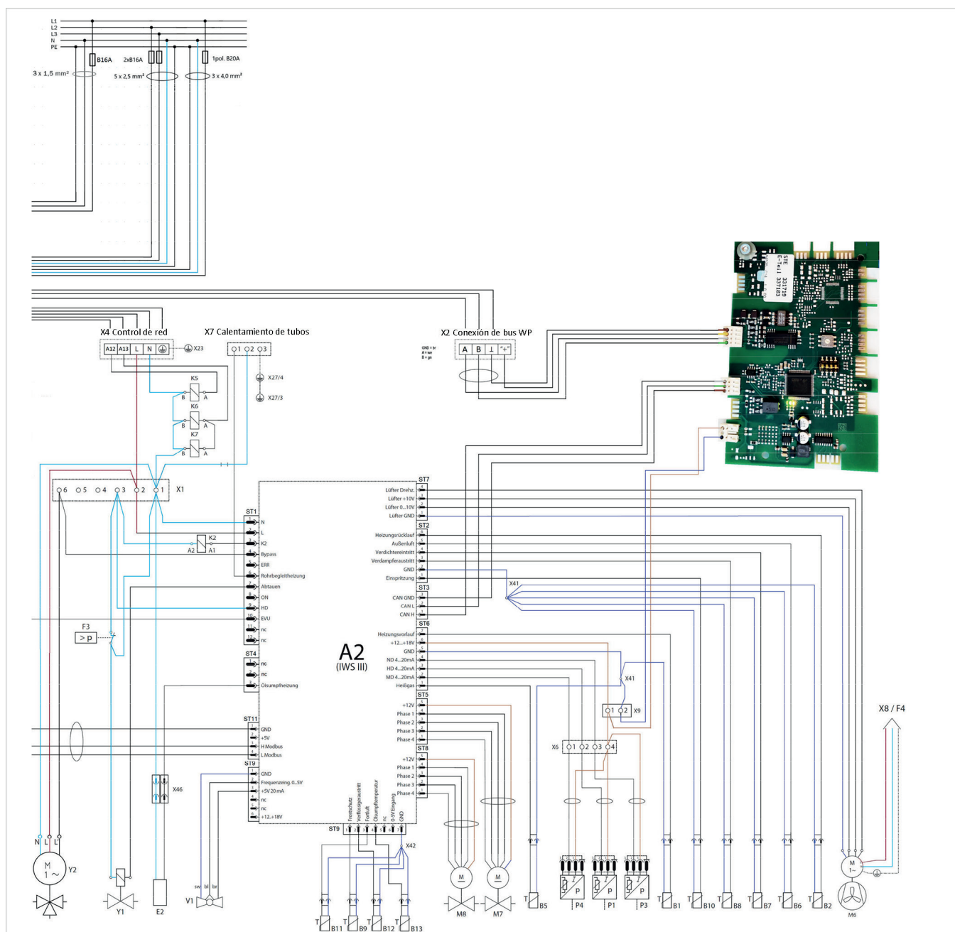
Fig. 44: Esquema de circuitos de SolvisLea 7 kW - Parte 2
