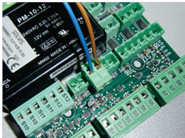
Abb. 2: Anschluss Gasdruckwächter an S14
