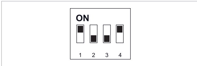
Abb. 35: Schiebeschalter WP-Typ
