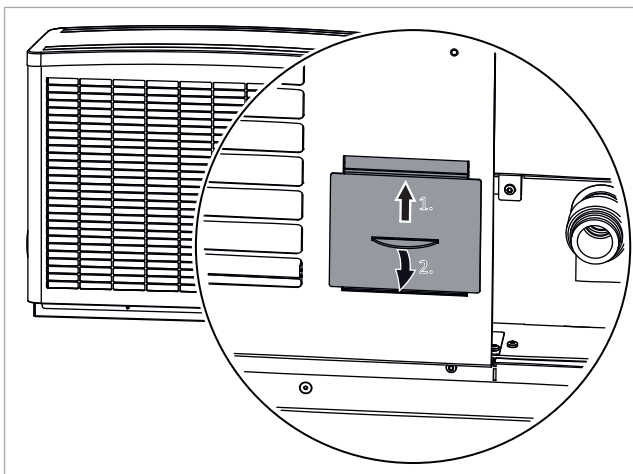
Abb. 34: Revisionsschacht öffnen
