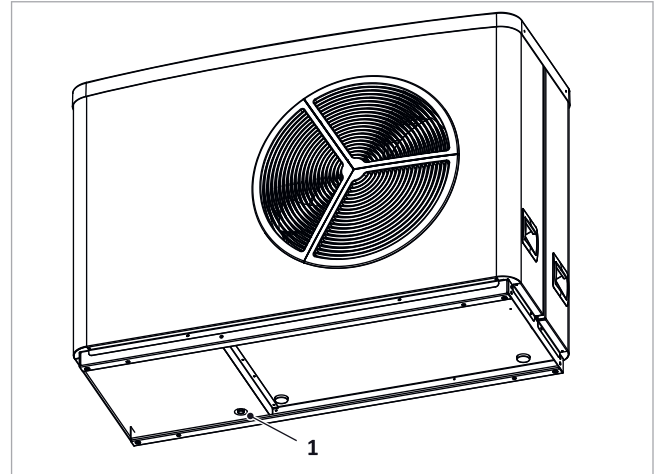
Abb. 19: SolvisLea: Kondensatablauf
