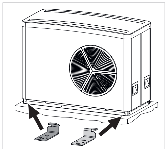
Abb. 10: Verschraubung auf Fundament
