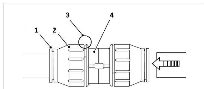
Abb. 15: Steckverbindung entriegelt
