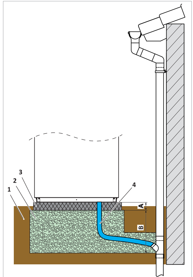
Abb. 9: Kondensatabfluss in Fallrohr oder Abfluss
