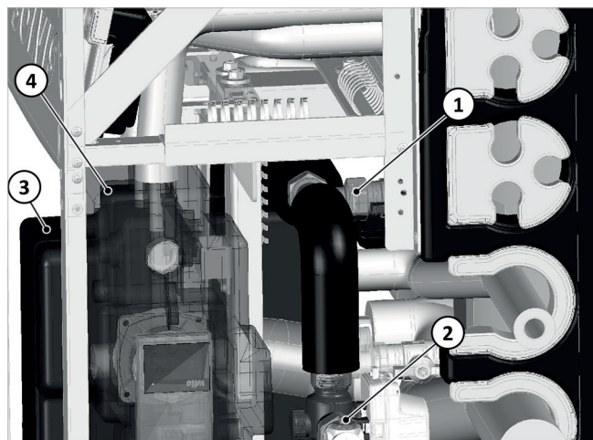
Abb. 4: Umschaltventil montieren (WP-Vorlauf nach rechts)
