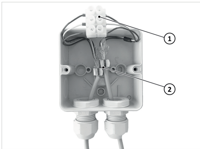
Abb. 16: Modbus-Verbindungsdose befestigen
