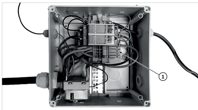
Abb. 18: Anschlussbox
