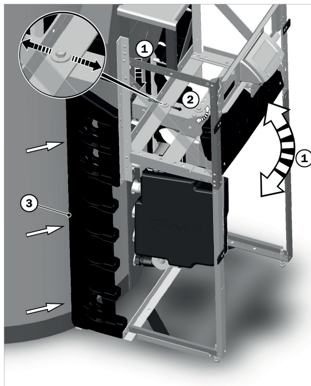
Abb. 11: Lademodul ausrichten
