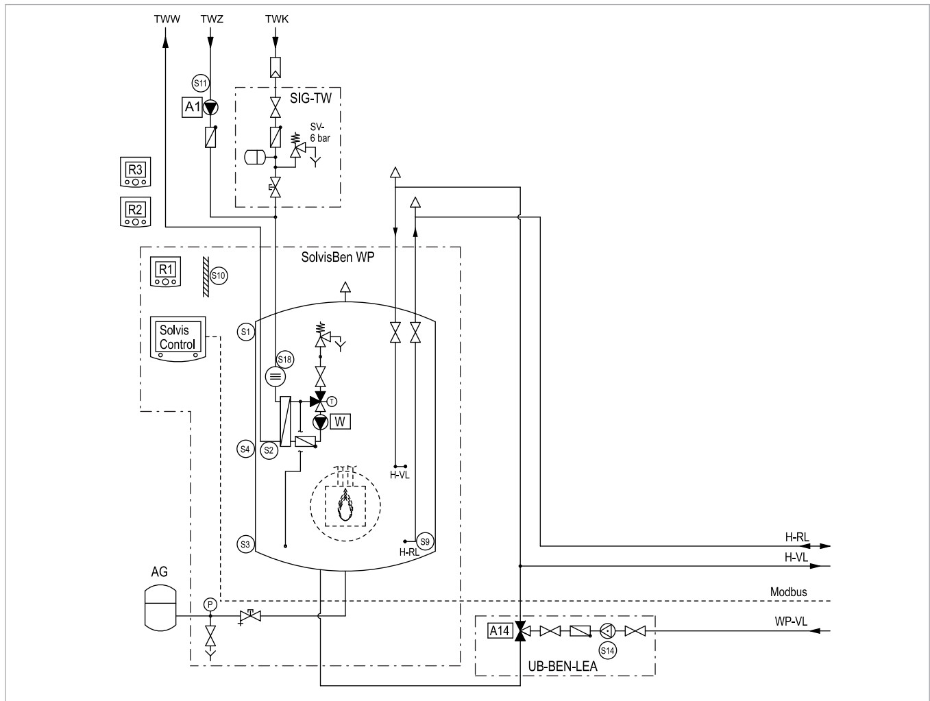
Abb. 19: SolvisBen WP drei gemischten Heizkreisen und Wärmepumpe SolvisLea - Teil 1
