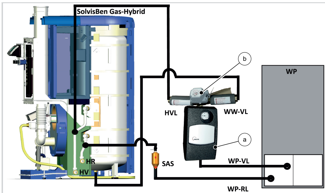
Abb. 8: Übersicht Anschluss SolvisLea an SolvisBen GAS-Hybrid, ohne integrierter Heizkreisstation (HKS)
