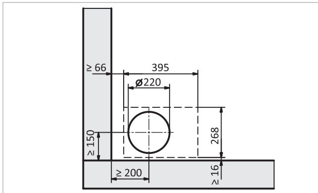
Abb. 16: Mauerdurchführung für Umschalteinheit, Wand links
