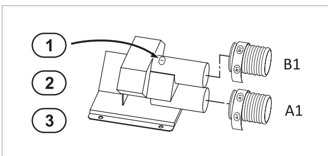
Abb. 15: Saugsonde
