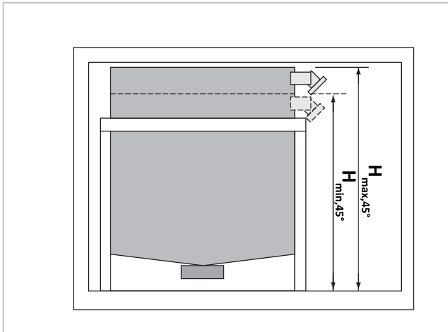
Abb. 93: Raumböhe bei Füllstutzen mit 45°
