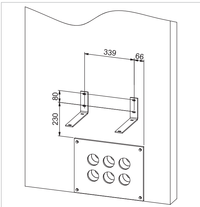
Abb. 33: Haltewinkel montieren
