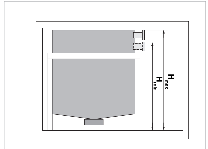
Abb. 94: Raumböhe bei geradem Füllstutzen
