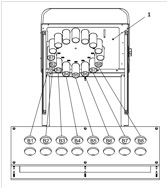
Abb. 85: Rückluftschläuche B1 bis B8 auf Umschalteteinheit montieren
