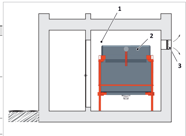
Abb. 3: SolvisvLinotank mit direkter Belüftungsöffnung ins Freie
