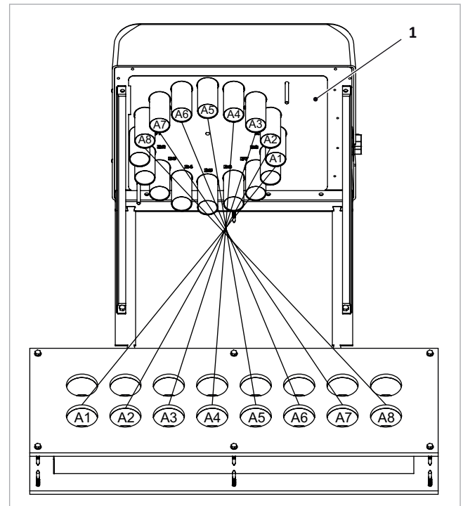
Abb. 86: Förderschläuche A1 bis A8 auf Umschalteteinheit montieren
