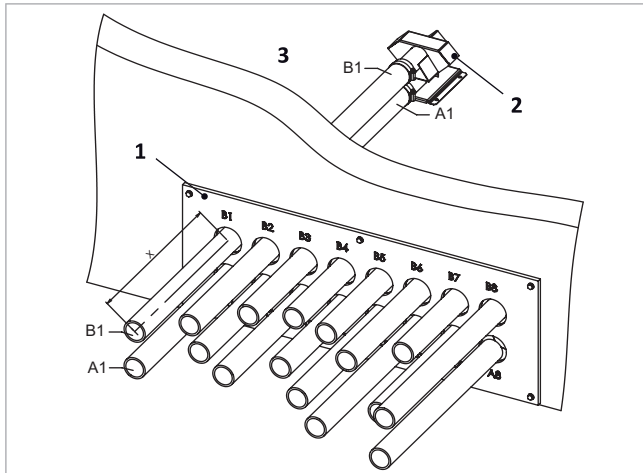
Abb. 78: Schlauch außerhalb des Lagerraumes ablängen
