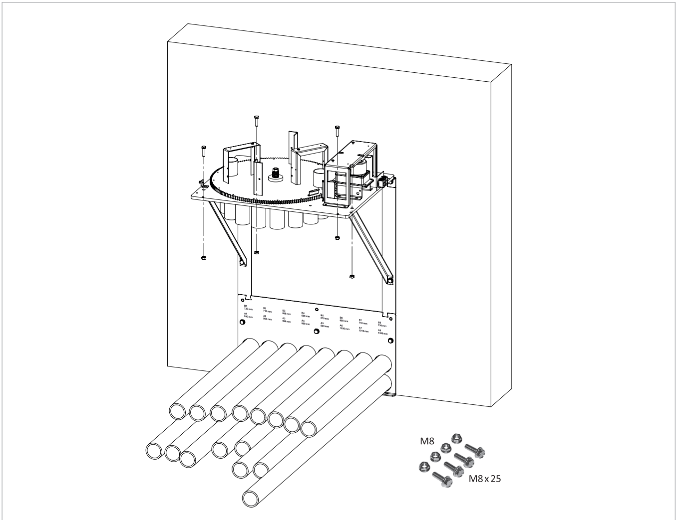
Abb. 63: Umschalteinheit montieren
