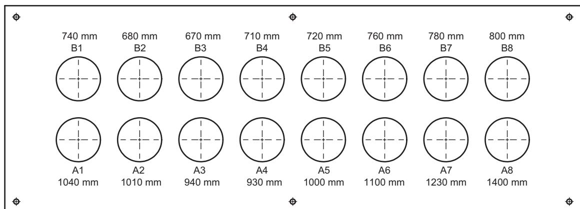
Abb. 77: Brandschott mit Längenangaben für Anschlüsse A1/B1 bis A8/B8
