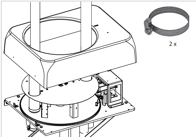
Abb. 90: Förder- und Rückluftschlauch anschließen
