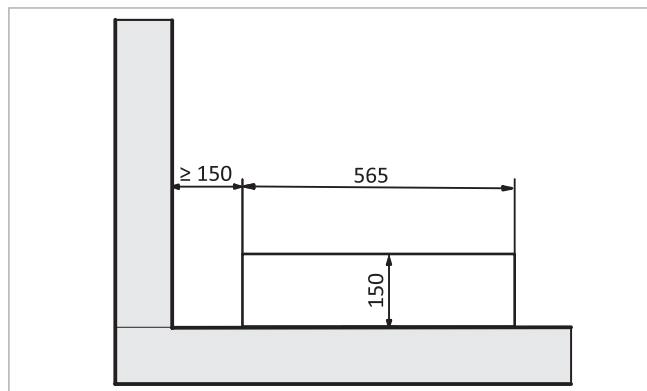
Abb. 54: Mauerdurchführung für Umschalteinheit, Wand links
