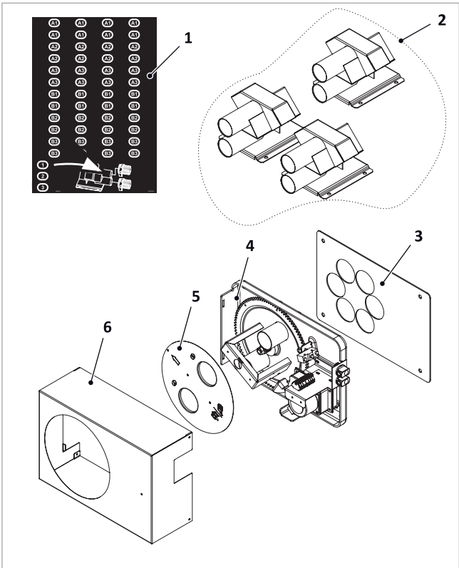
Abb. 11: Lieferumfang 3-Saugsonden-System
