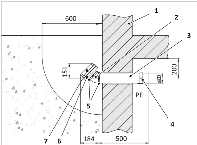
Abb. 119: 45°-Stutzen im Lichtschacht – Seitenansicht
