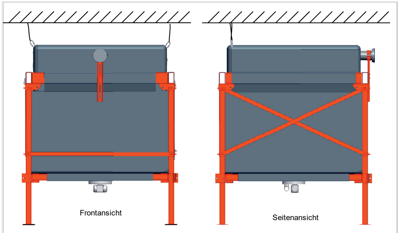
Abb. 111: SolvisLinotank, Gewebesack hinten aufgehängt
