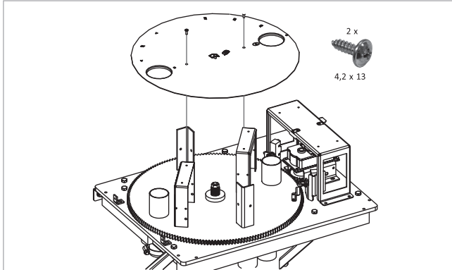
Abb. 87: Abdeckscheibe auf Umschalteinheit montieren
