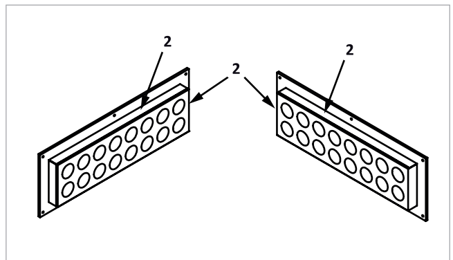
Abb. 74: Brandschott mit Brandschutzband an je 2 Seiten
