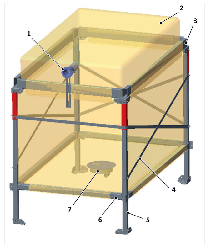
Abb. 10: SolvisLinotank mit Entnahmetopf
