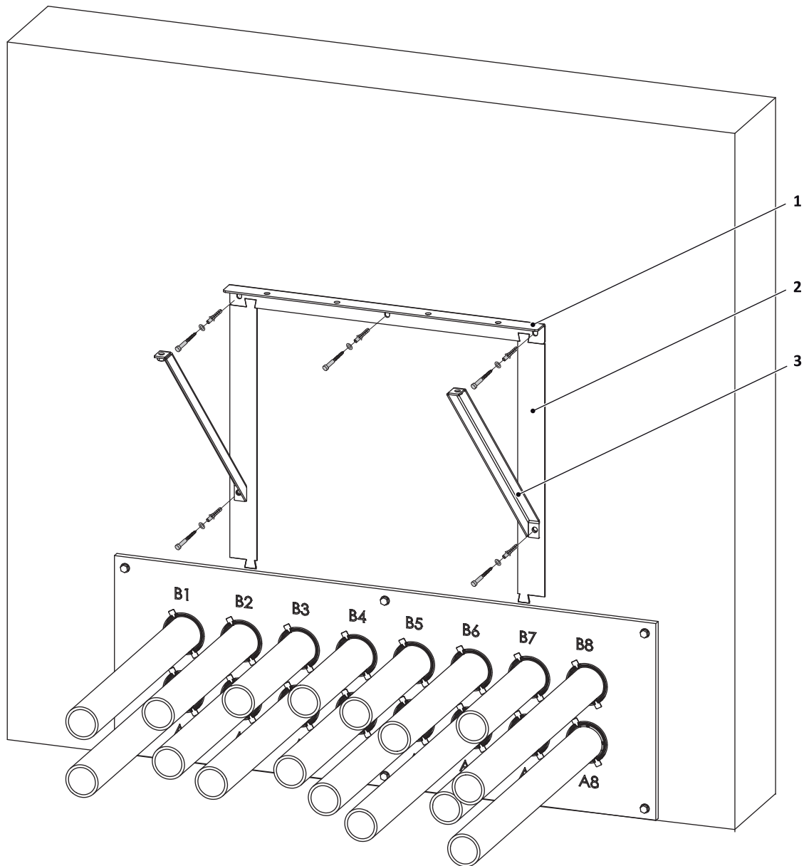
Abb. 82: Montagewinkel (1), Verbinder (2) und Abstützwinkel (3) montieren
