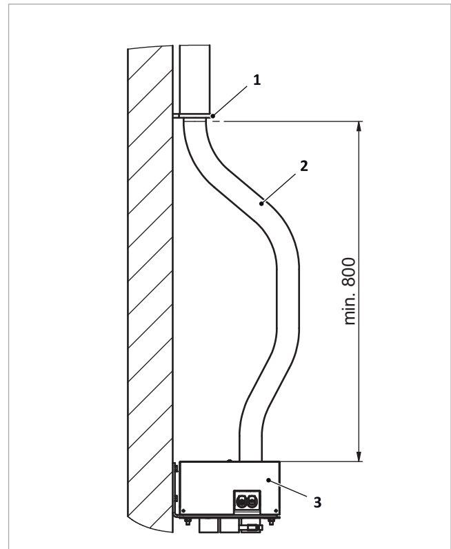
Abb. 88: Schlauchbefestigung Wand mit HT-Rohr
