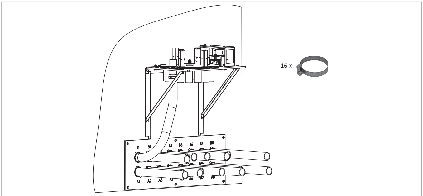
Abb. 84: Schläuche der Reihe nach von B1 bis B8 und danach von A1 bis A8 auf Umschalteteinheit montieren
