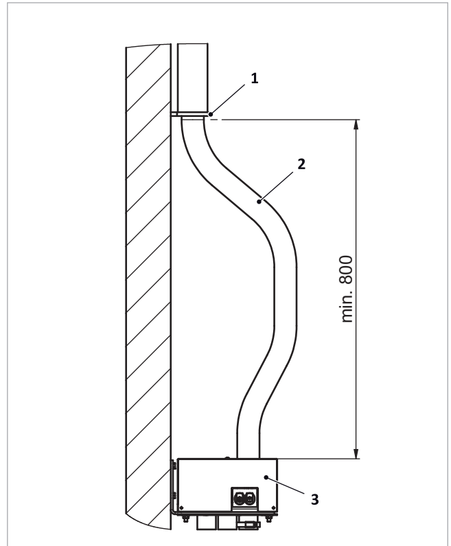
Abb. 68: Schlauchbefestigung Wand mit HT-Rohr
