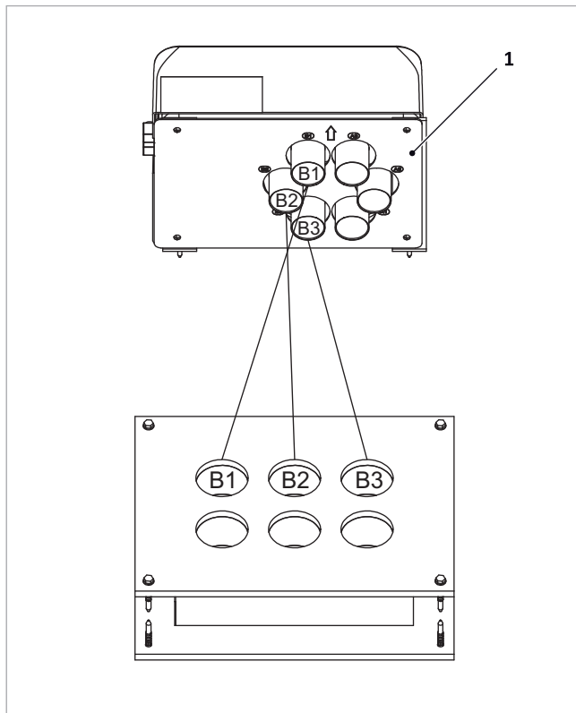
Abb. 41: Rückluftschläuche B1 bis B3 auf Umschalteneinheit montieren
