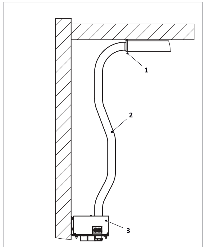
Abb. 69: Schlauchbefestigung Decke mit HT-Rohr
