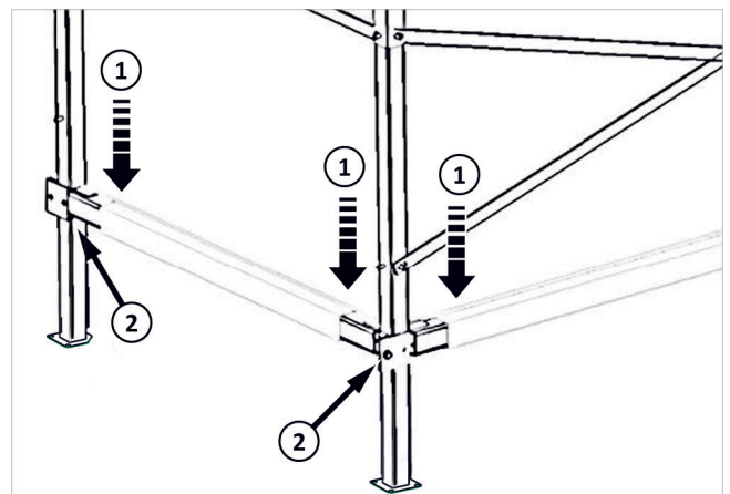
Abb. 103: Gewebe spannen
