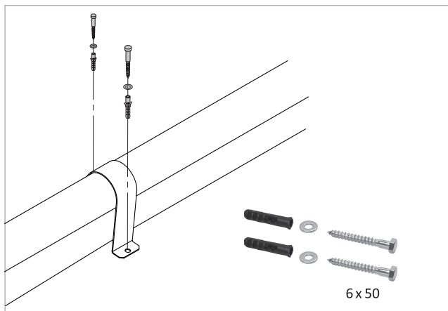
Abb. 38: Schläuche mit Befestigungsschellen am Boden fixieren
