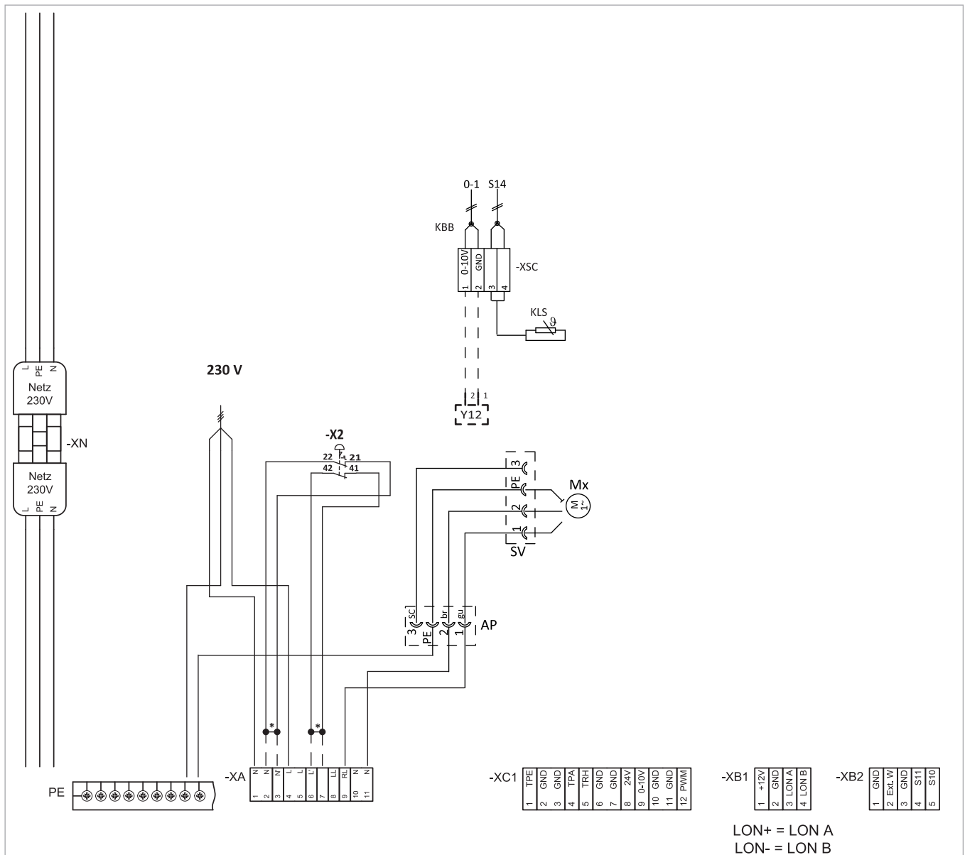
Abb. 134: Anschlussplan Maulwurfentnahme
