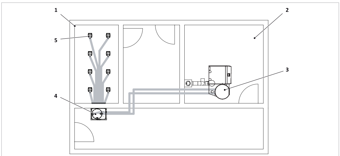
Abb. 50: Ansicht von Lager- und Heizraum von oben
