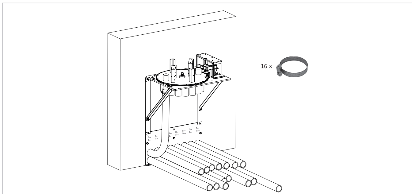
Abb. 64: Schläuche der Reihe nach von B1 bis B8 und danach von A1 bis A8 auf Umschalteteinheit montieren
