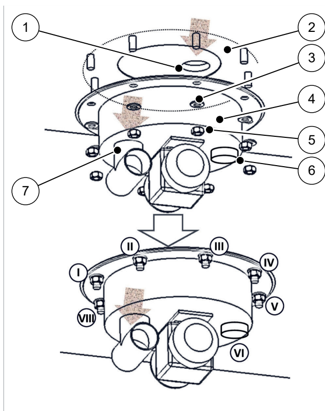
Abb. 128: Muttern entfernen (außer I und V)
