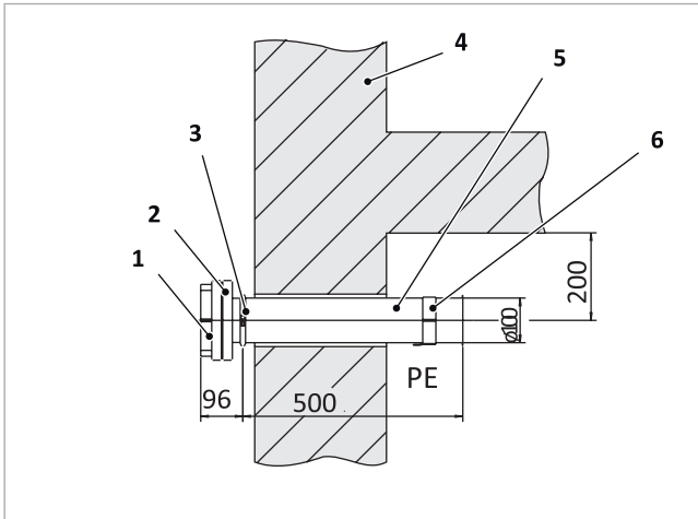
Abb. 118: Gerader Stutzen eingemauert – Seitenansicht
