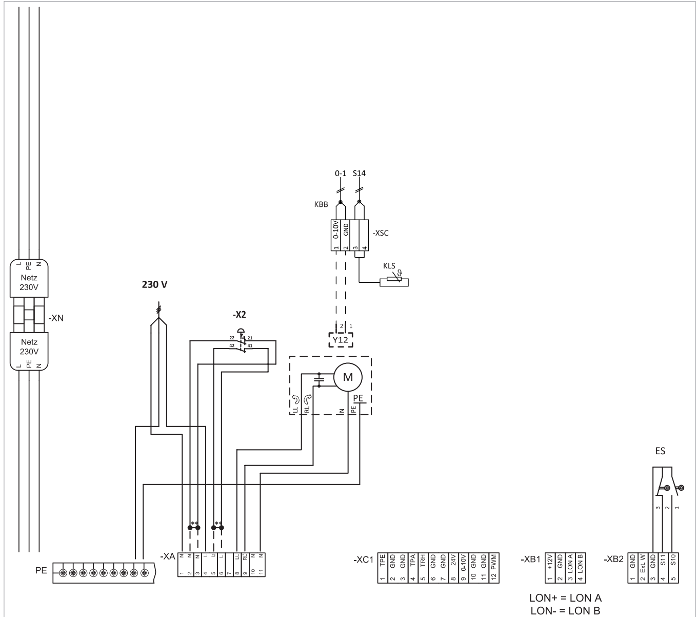
Abb. 133: Anschlussplan Umschalteinheit
