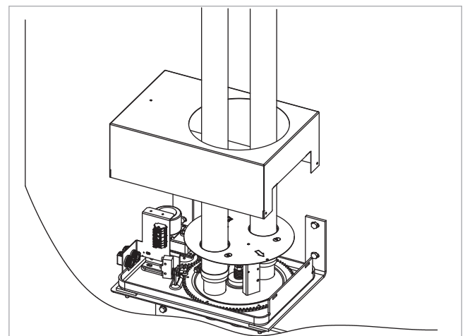
Abb. 45: Förder- und Rückluftschauch anschließen
