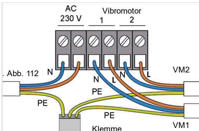
Abb. 125: VMU-Steuerungsbox
