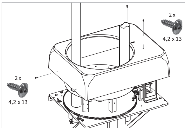
Abb. 71: Abdeckhaube montieren
