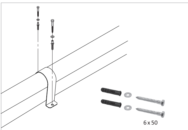
Abb. 21: Schläuche mit Befestigungsschellen am Boden fixieren
