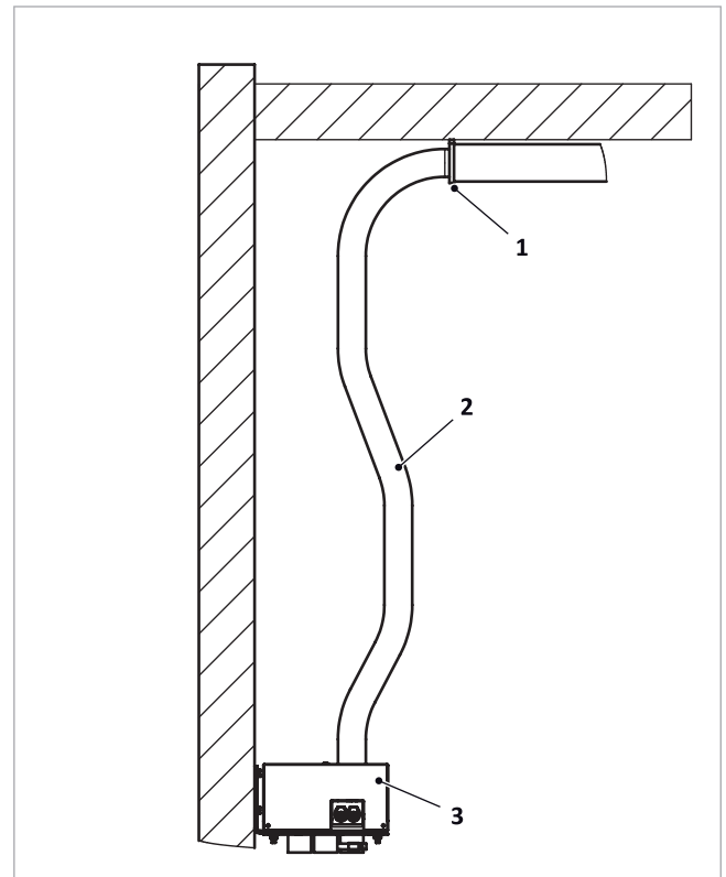
Abb. 44: Schlauchbefestigung Decke mit HT-Rohr
