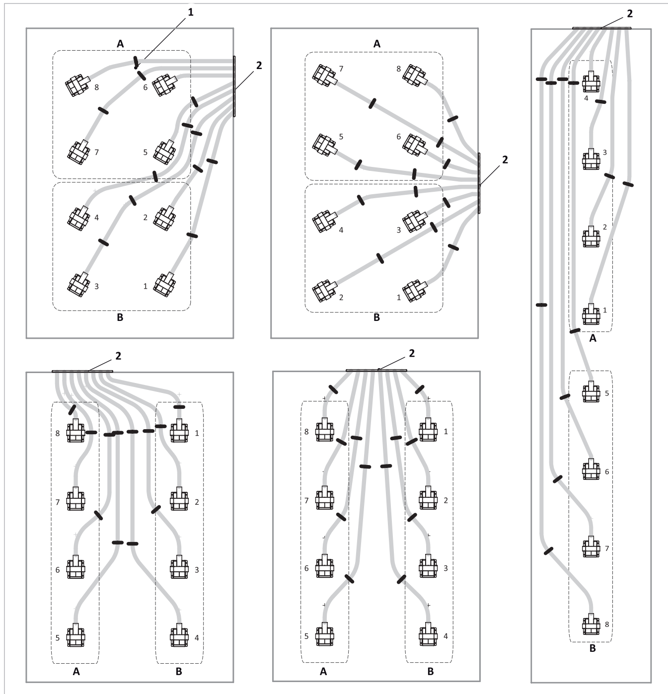
Abb. 51: Varianten Saugsondenanordnung
