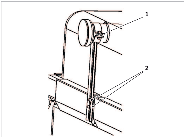
Abb. 108: Füllrohrhalter handfest anschrauben
