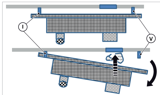
Abb. 129: Öffnung im Silokörper verschließen
