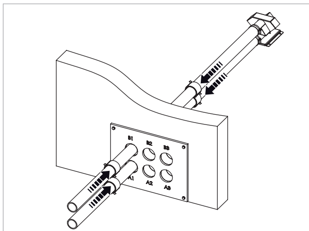
Abb. 37: Brandschutzmanschetten einsetzen
