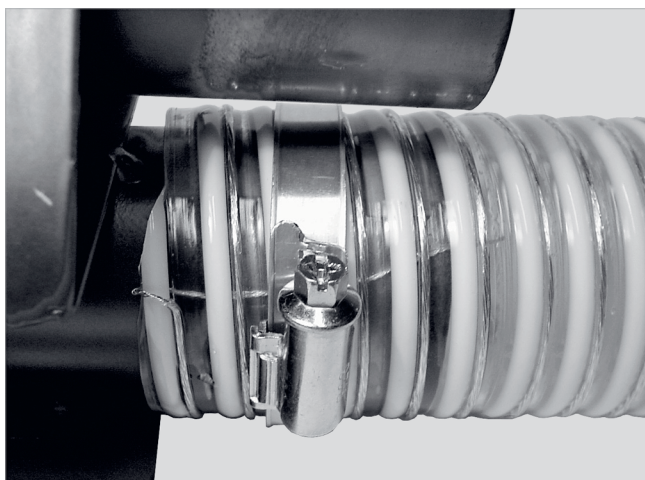
Abb. 2: Schlauchschelle montieren
