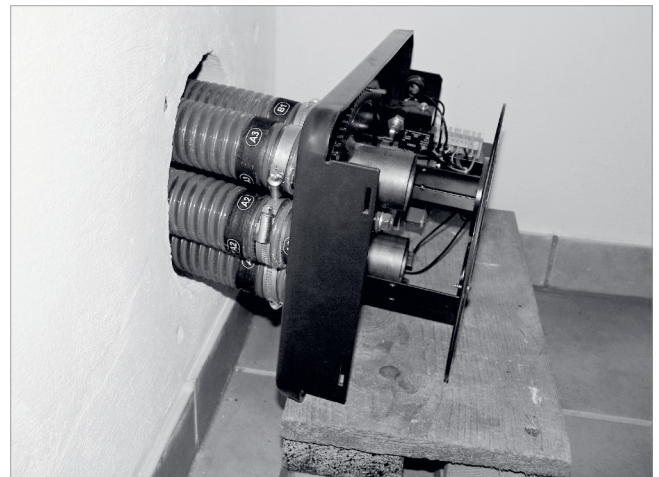
Abb. 23: Umschalteinheit Schläuche montiert
