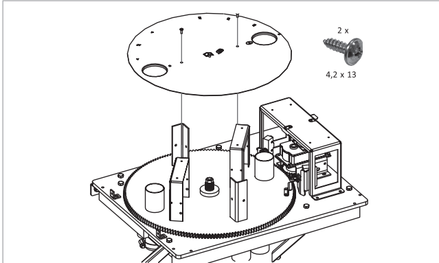
Abb. 67: Abdeckscheibe auf Umschalteinheit montieren
