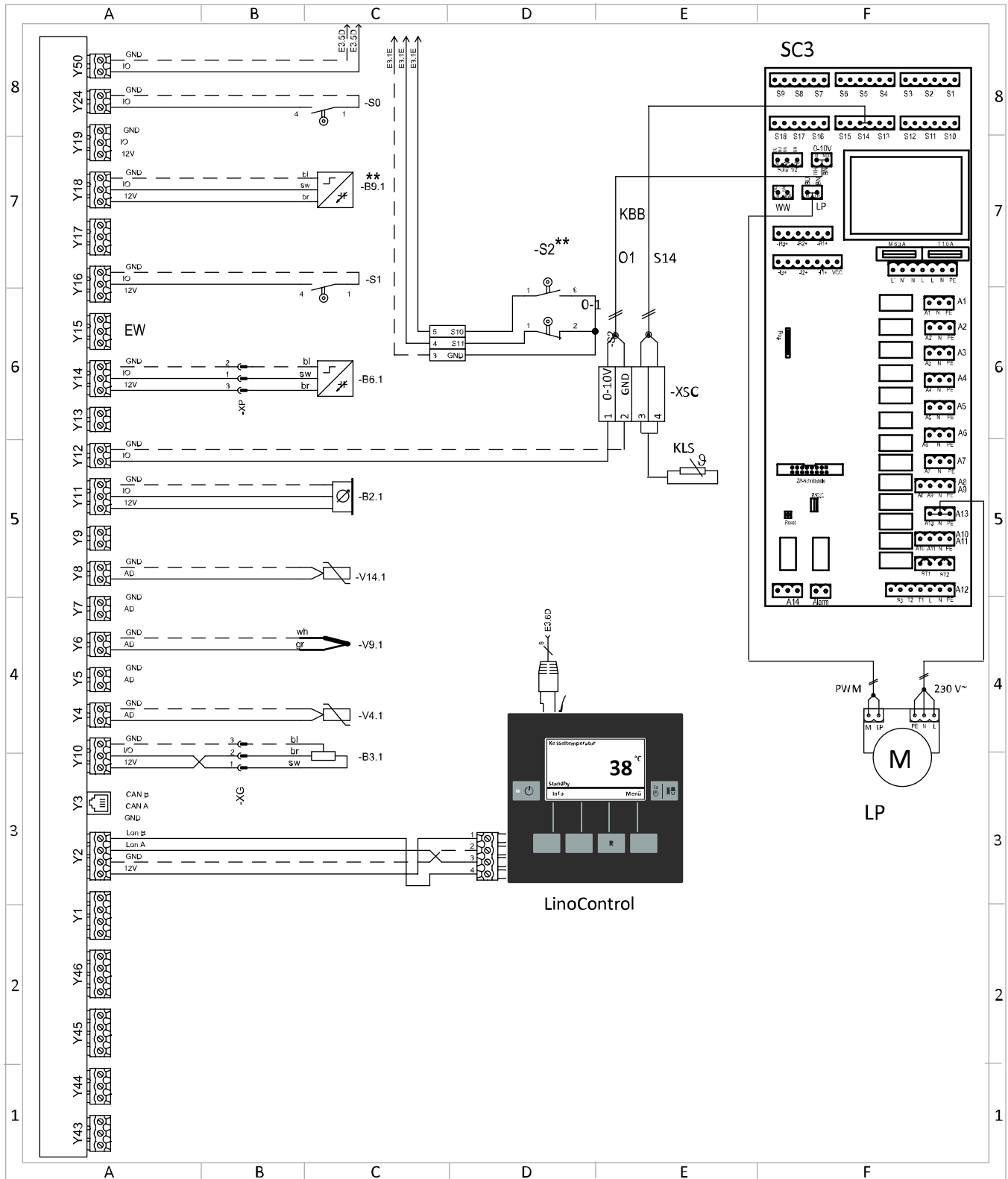
Abb. 131: Grundschaltbild SolvisLino 4 / SolvisLino 5 (Plan E2)
