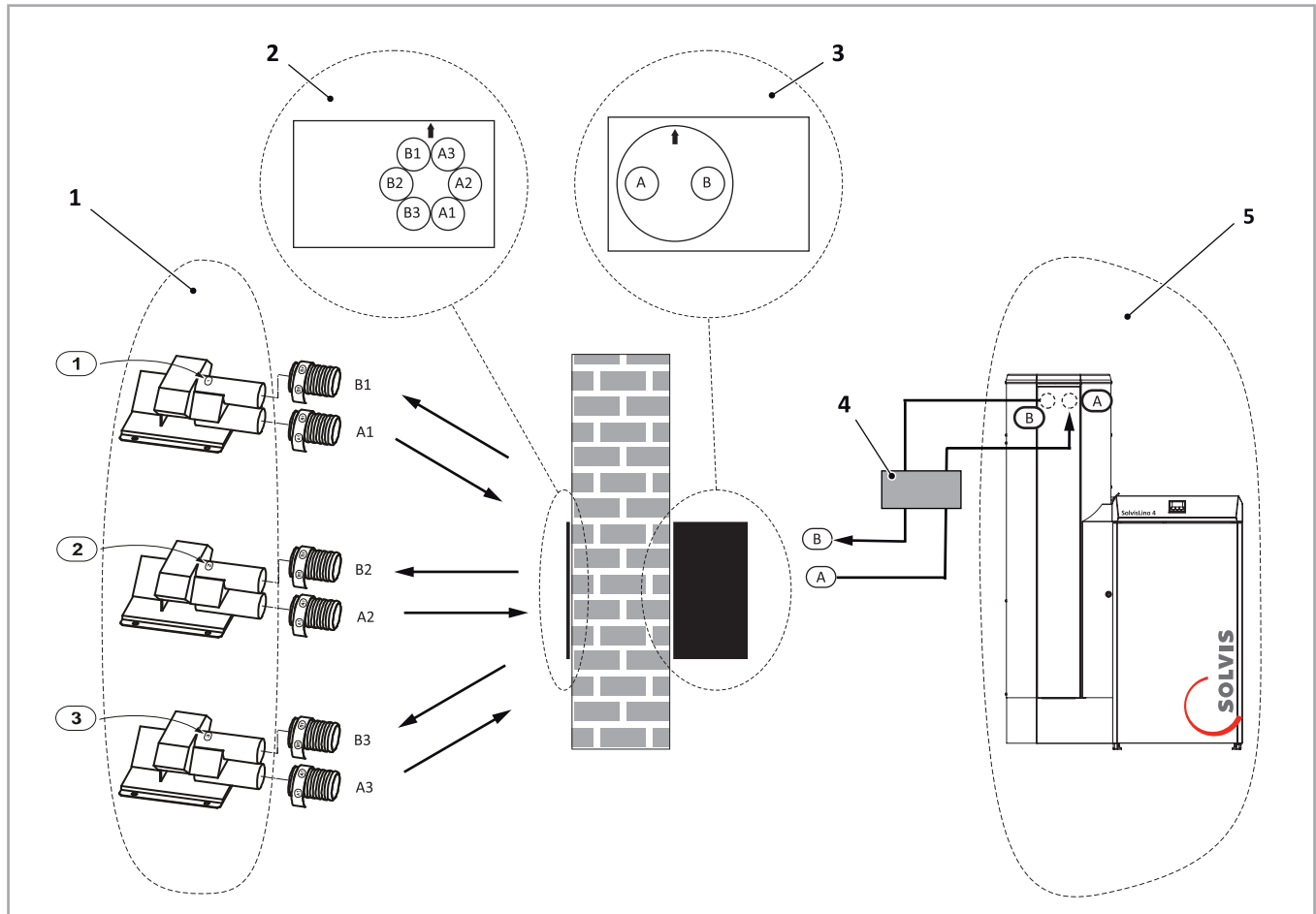
Abb. 13: Anschluss-Übersichtsskizze
