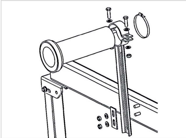
Abb. 107: Zusammenbau der Füllrohrhalterung
