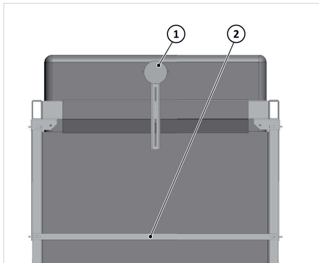
Abb. 96: SolvisLinotank zusammengebaut (Füllseite)
