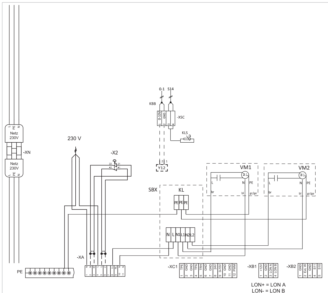
Abb. 136: Anschlussplan Vibrationseinheiten der beiden Entnahmetöpfe am SolvisLinotank ab B = 3,25 m
