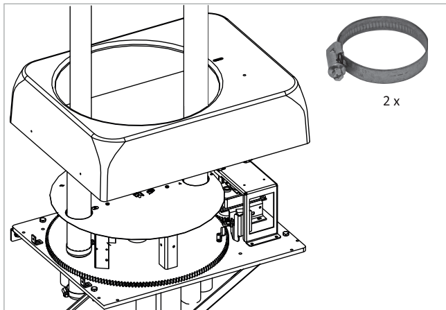
Abb. 70: Förder- und Rückluftschlauch anschließen
