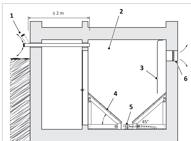
Abb. 6: Pelletlager mit Lüftungsdistanz größer 2 m
