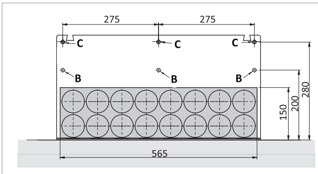
Abb. 57: Befestigungslöcher bohren, Abdeckplatte innen montieren
