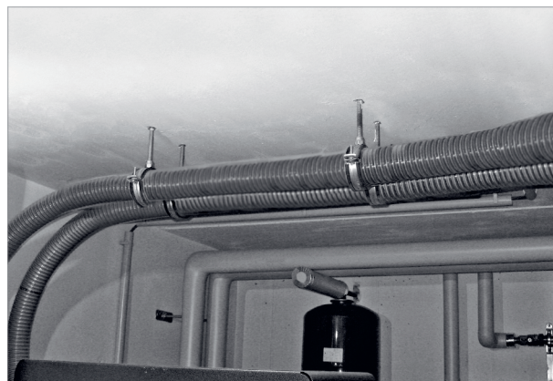
Abb. 26: Förderschläuche befestigen
