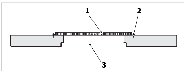
Abb. 122: Pelletlagerraumtür – Ansicht von oben
