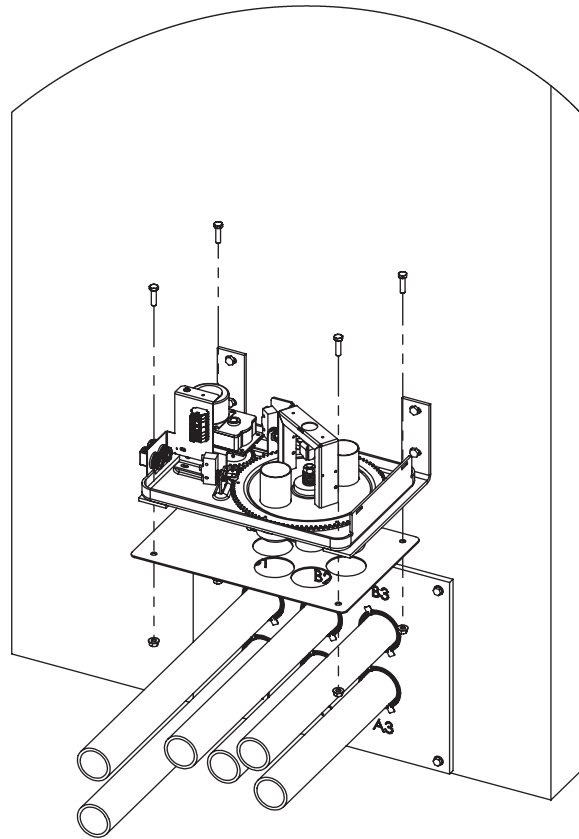
Abb. 39: Umschalteinheit und Abdeckplatte montieren
