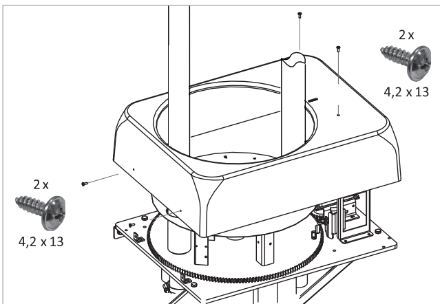
Abb. 91: Abdeckhaube montieren
