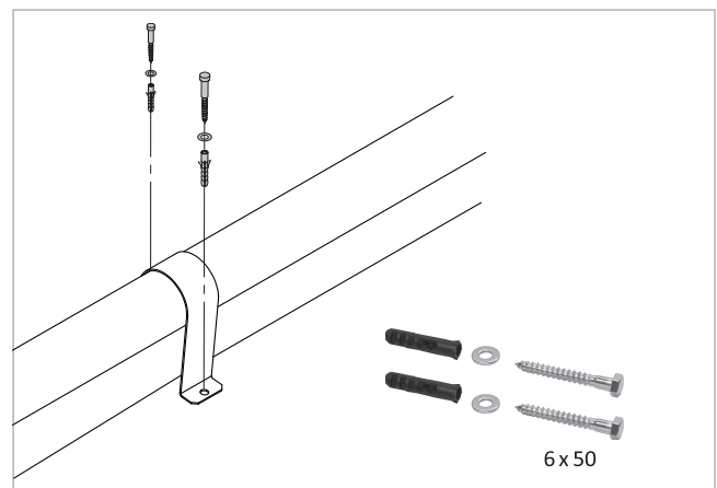
Abb. 81: Schläuche mit Befestigungsschellen am Boden fixieren
