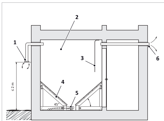
Abb. 5: Pelletlager mit Befüllanschluss nach unten verlegt
