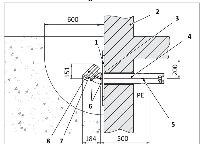
Abb. 114: 45°-Stutzen im Lichtschacht – Seitenansicht
