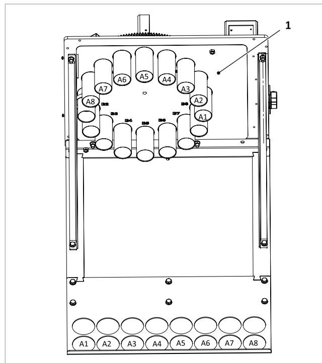
Abb. 66: Förderschläuche A1 bis A8 auf Umschalteteinheit montieren
