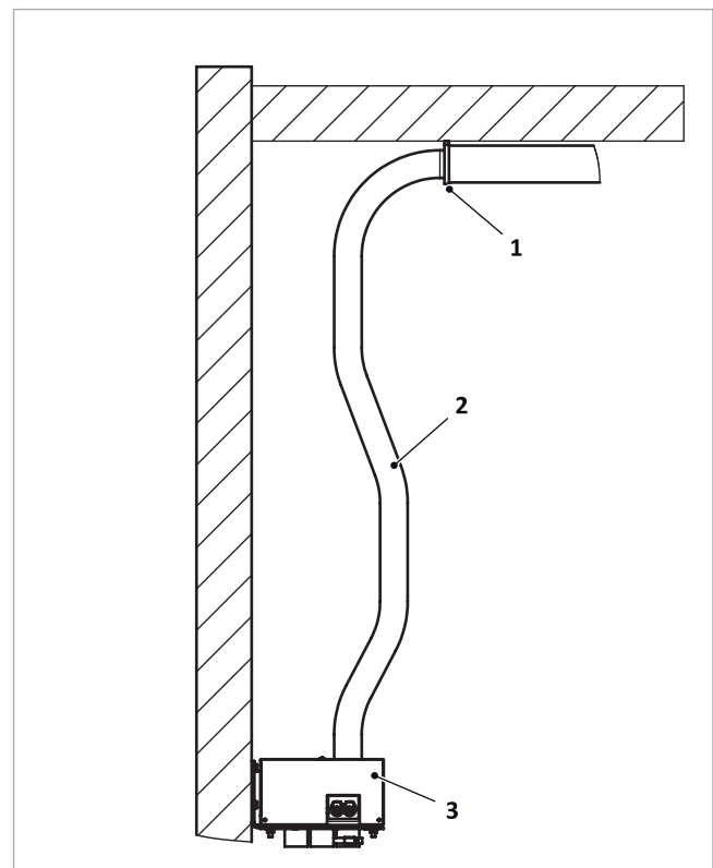
Abb. 89: Schlauchbefestigung Decke mit HT-Rohr
