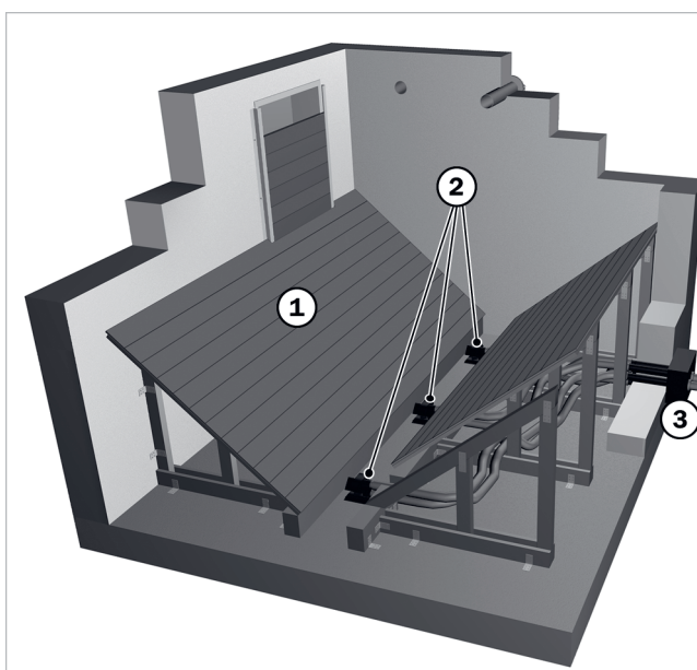
Abb. 7: Pelletlagerraum mit 3-Saugsonden-System
