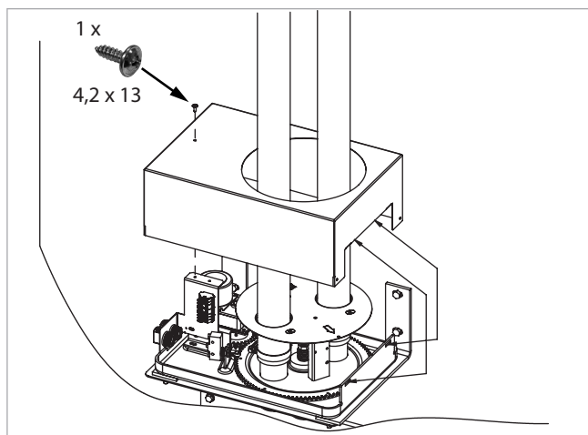
Abb. 46: Abdeckhaube montieren
