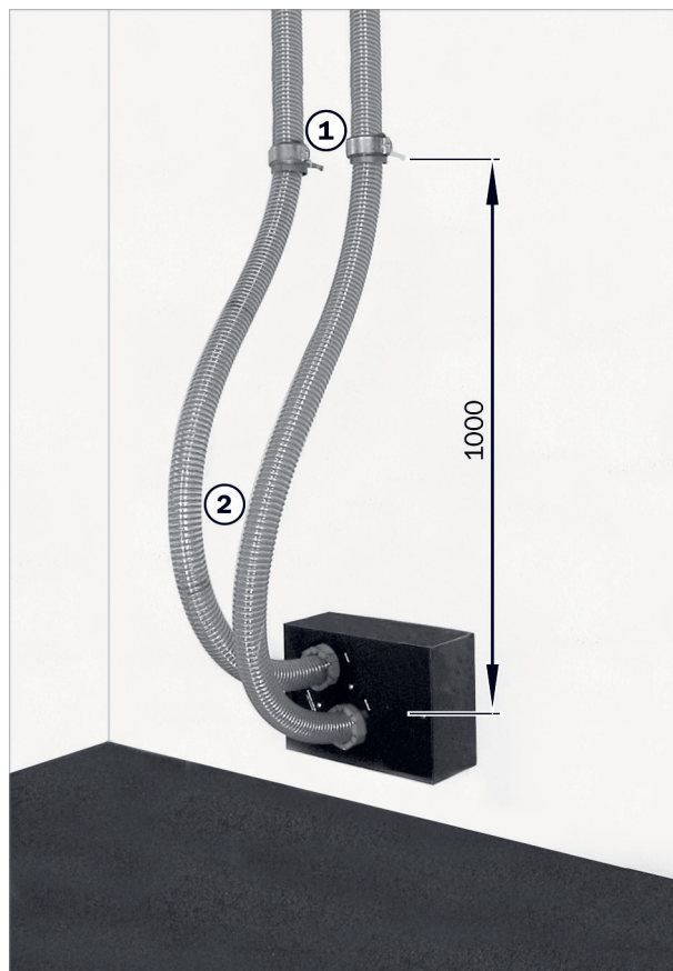
Abb. 27: Anschluss-Umschalteinheit
