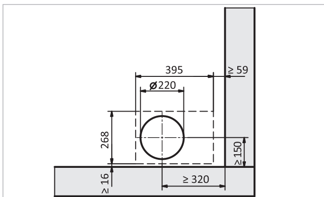
Abb. 17: Mauerdurchführung für Umschalteinheit, Wand rechts
