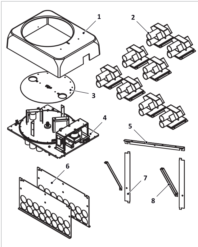
Abb. 47: Lieferumfang 8-Saugsonden-System
