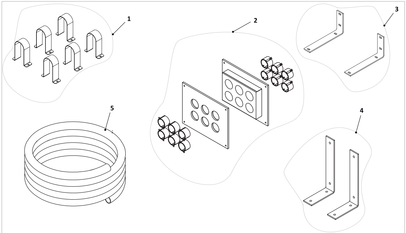
Abb. 12: Zubehör (bitte separat bestellen) für Saugsonden-System mit vollautomatischer Pelletzuführung
