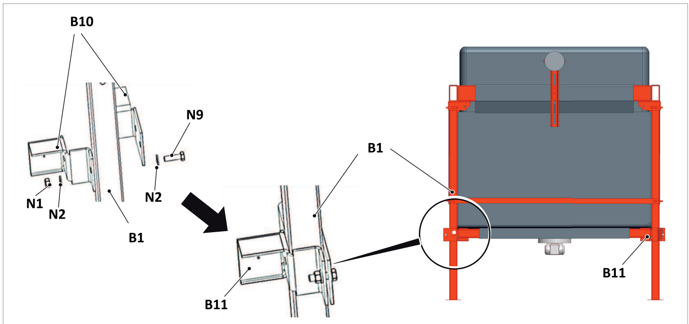
Abb. 101: Spreizriegelhalter anbringen
