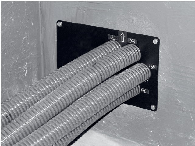
Abb. 20: Abdeckplatte mit Schlauchenden eingesteckt
