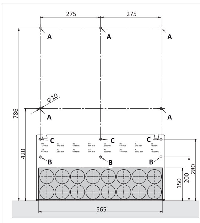
Abb. 56: Befestigungslöcher bohren, Abdeckplatte außen montieren
