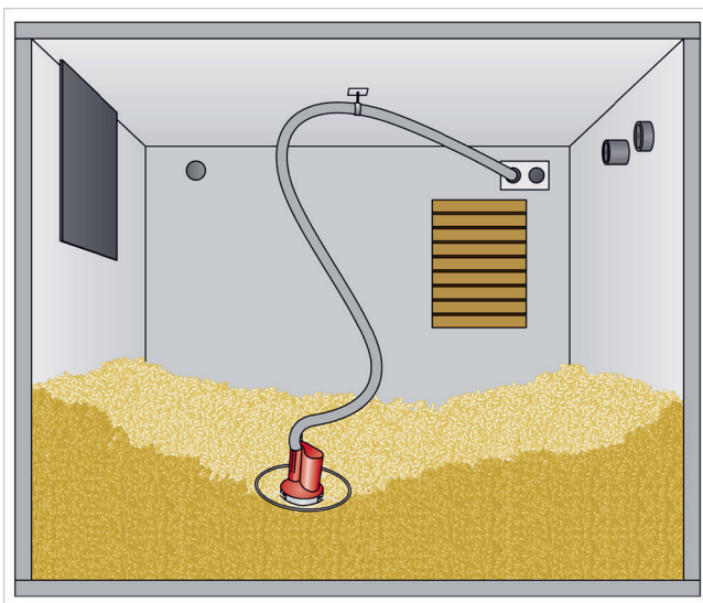
Abb. 9: Pelletlagerraum mit Maulwurfentnahme
