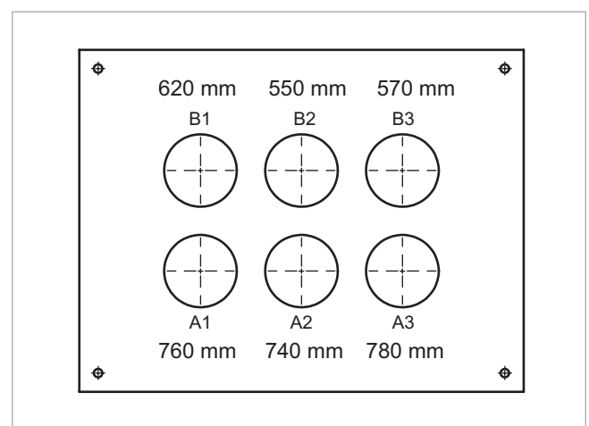
Abb. 34: Abdeckplatte mit Längenangaben für Anschluss A1/B1 bis A3/B3
