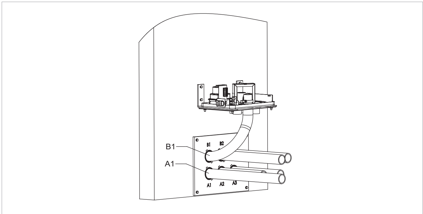
Abb. 40: Schläuche der Reihe nach von B1 bis B3 und danach von A1 bis A3 auf Umschalteneinheit montieren
