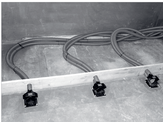
Abb. 25: Sonden anschließen
