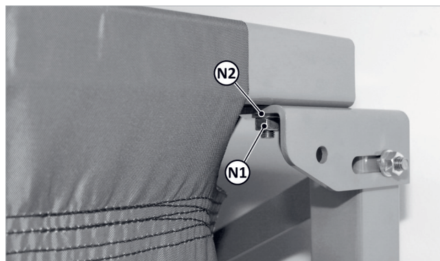
Abb. 98: Tragschiene festschrauben
