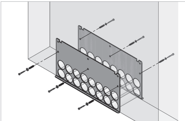
Abb. 58: Abdeckplatten ausrichten und festschrauben
