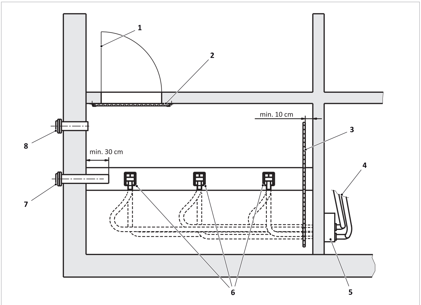
Abb. 14: Pellet-Lagerraum – Ansicht von oben
