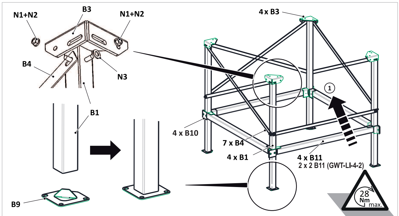
Abb. 95: Zusammenbau des Stahlgestelles, Bauhöhe SolvisLinotank 1,65 m (alle Schrauben mit max. 28 Nm anziehen)
