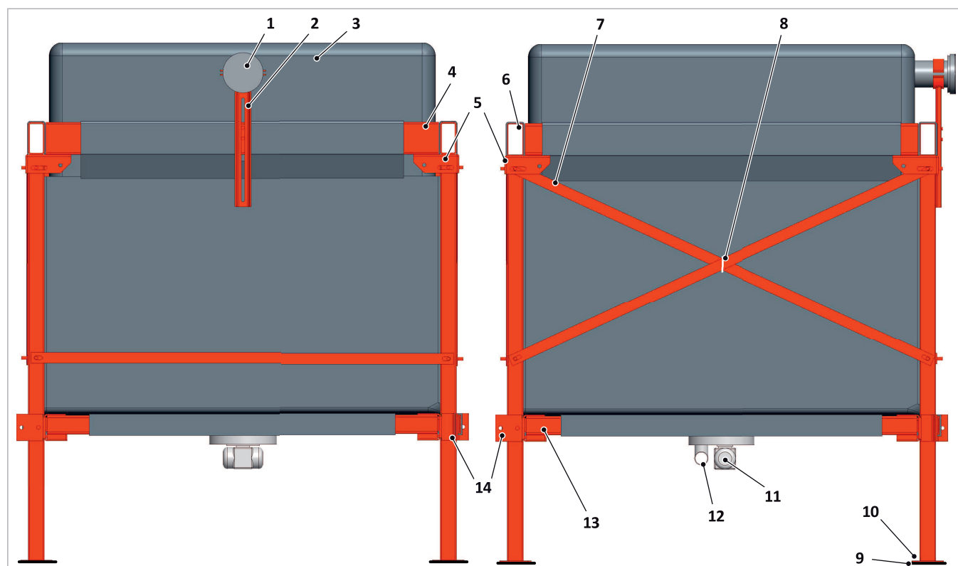
Abb. 92: Bauteile des SolvisLinotanks (ab Baugröße 2,54 m Ausführung mit zwei nebeneinanderliegenden Füllrohren, Pos. 1)
