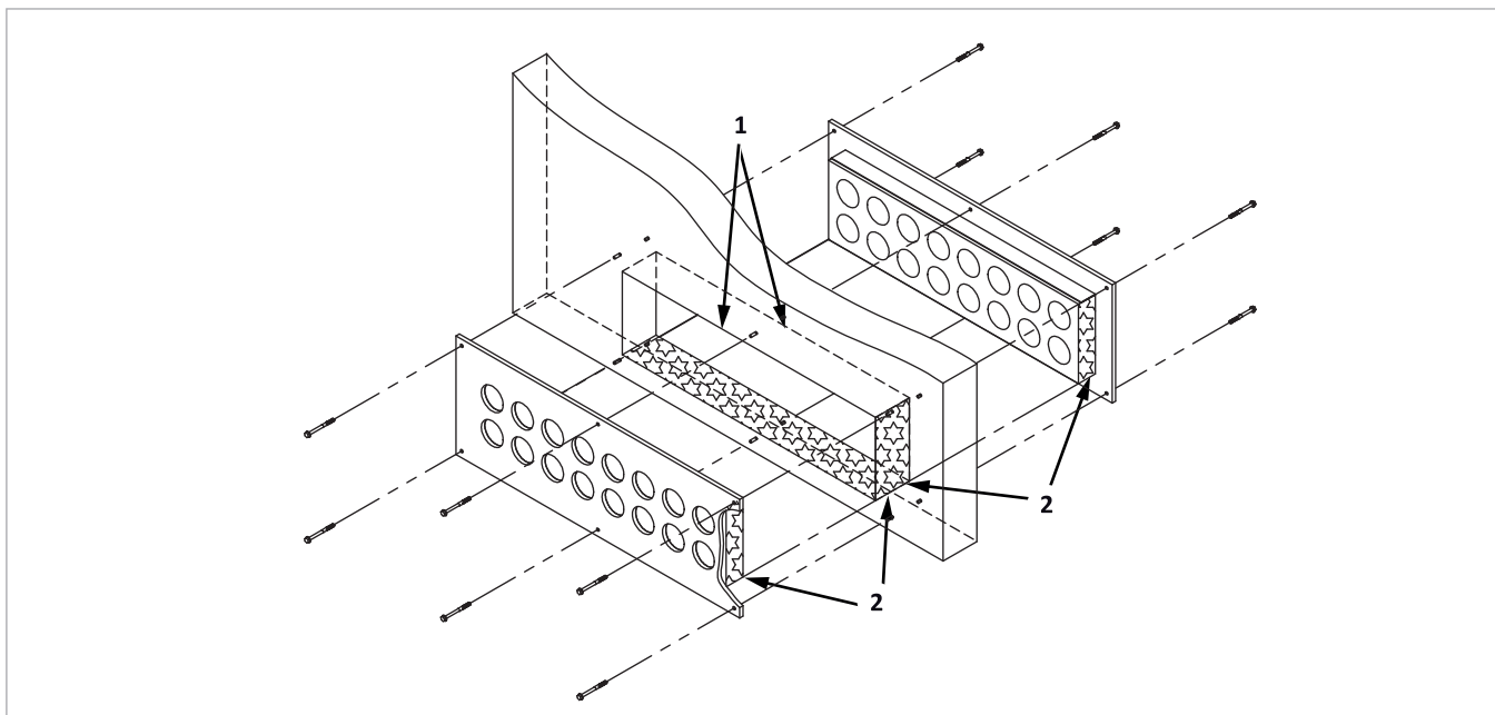
Abb. 75: Brandschott in Mauerdurchführung einbauen
