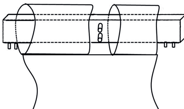
Abb. 99: Tragriegel mit Bolzen eingeschlaucht
