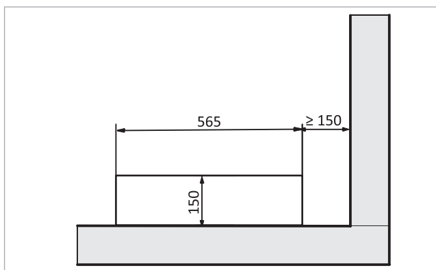
Abb. 55: Mauerdurchführung für Umschalteinheit, Wand rechts
