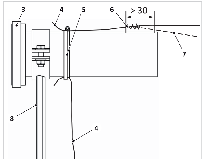
Abb. 109: Gewebesack überstülpen und befestigen
