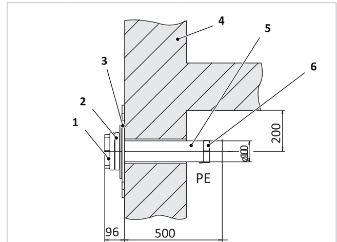
Abb. 113: Gerader Stutzen – Seitenansicht
