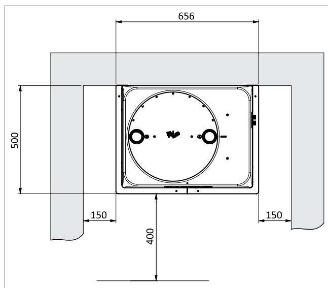
Abb. 53: Umschalteinheit. Ansicht von oben (alle Maße in mm)
