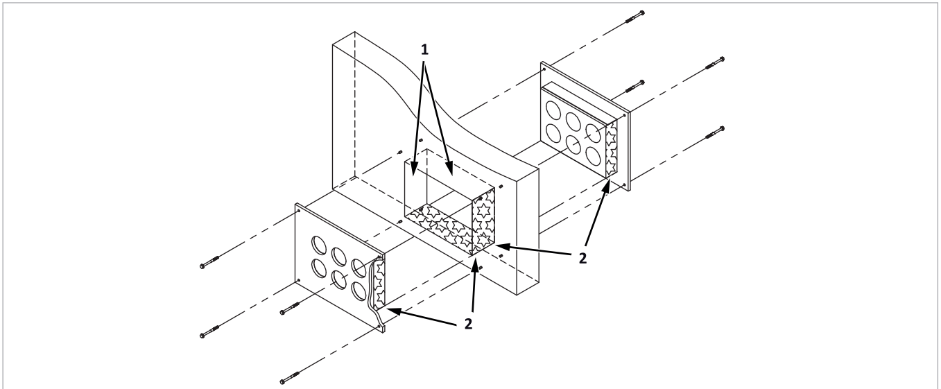
Abb. 32: Brandschott in Mauerdurchführung
