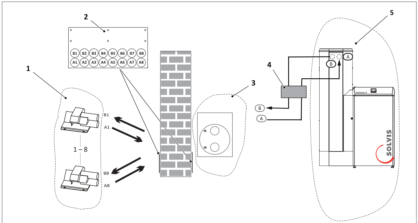
Abb. 49: Anschluss-Übersichtsskizze
