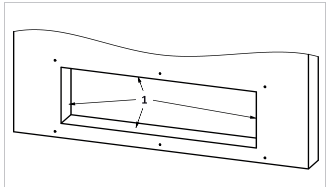
Abb. 73: Laibungen mit Glattstrich (1)
