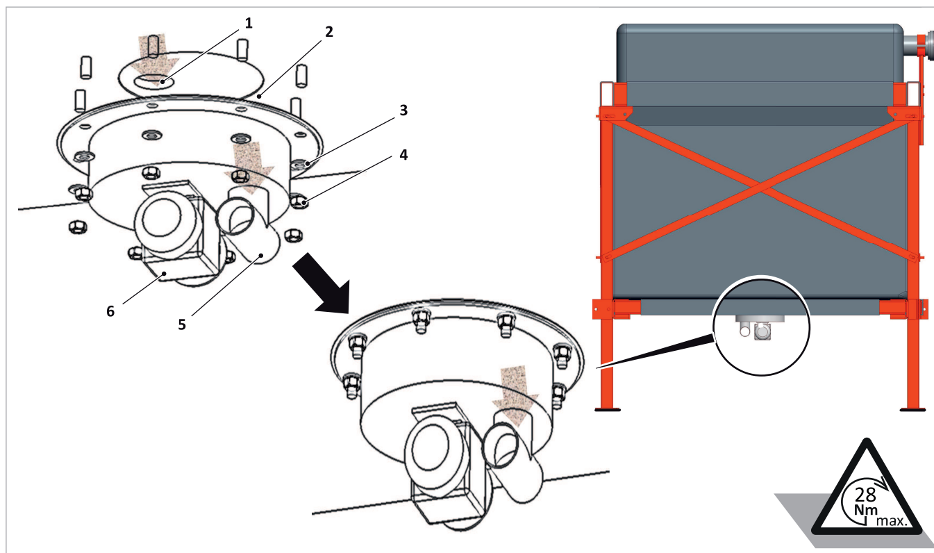
Abb. 105: Montage des Entnahmetopfes mit Vibrationseinheit (maximales Anzugsdrehmoment der Muttern 28 Nm)
