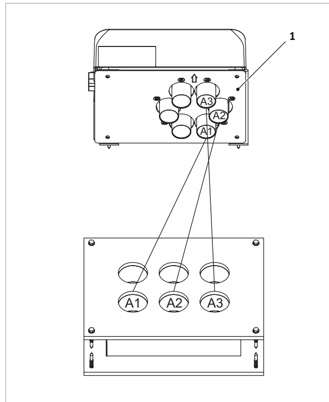
Abb. 42: Förderschläuche A1 bis A3 auf Umschalteneinheit montieren
