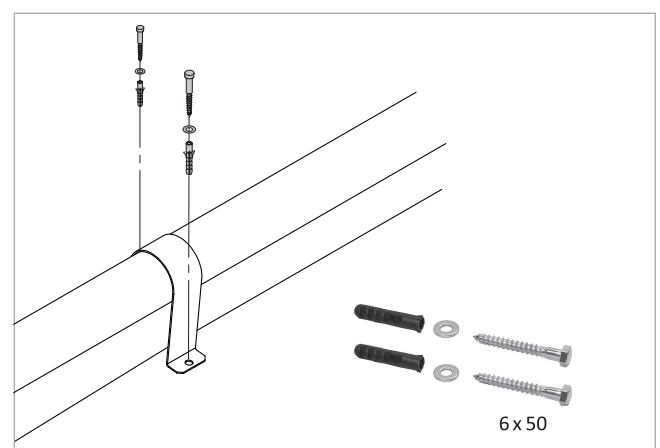
Abb. 61: Schläuche mit Befestigungsschellen am Boden fixieren
