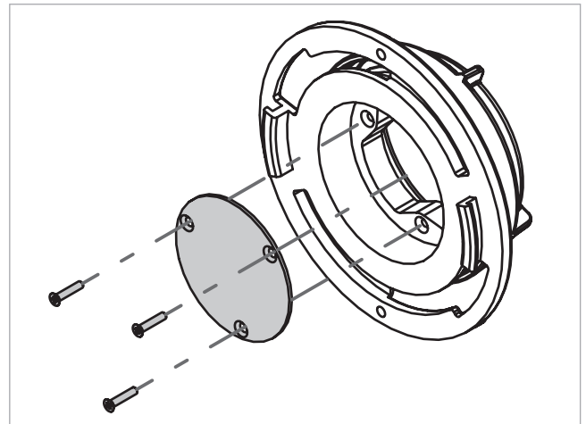
Abb. 120: Kupplungsdeckel mit Dichtscheibe
