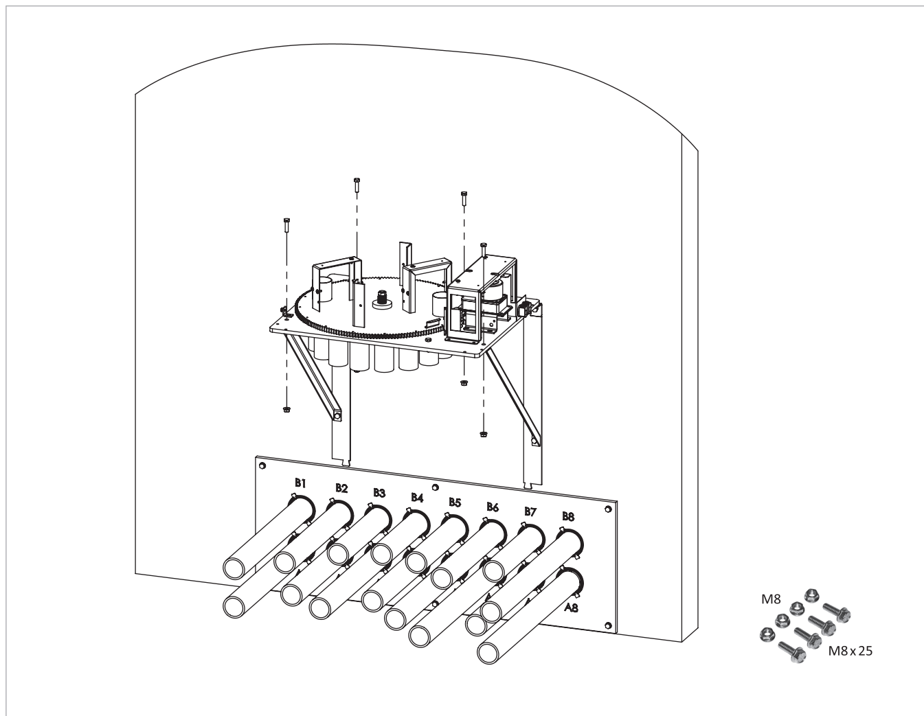
Abb. 83: Umschaltseinheit montieren
