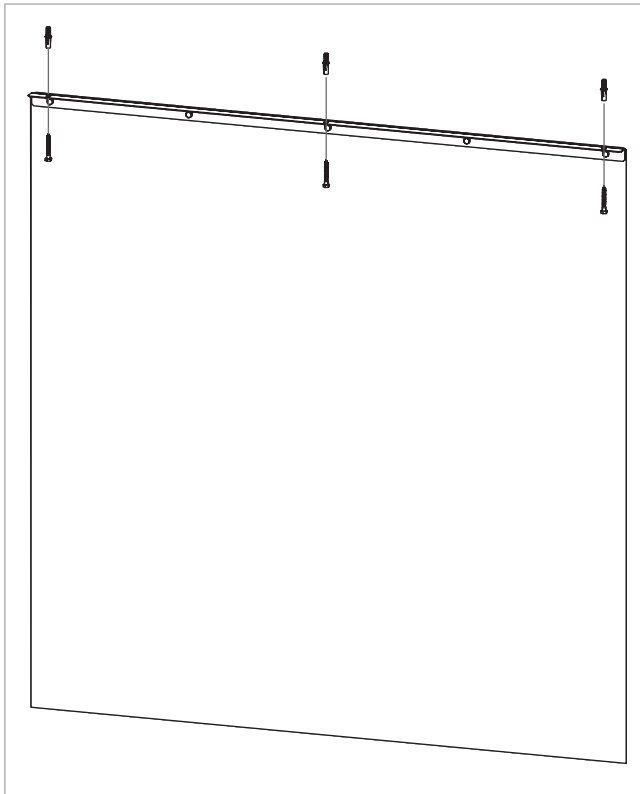
Abb. 121: Prallschutzmatte
