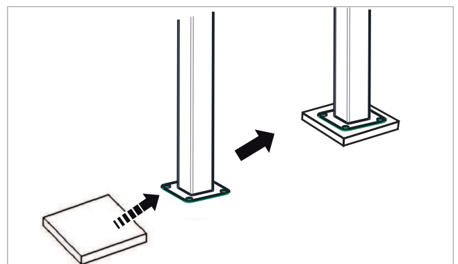
Abb. 104: Dämmplatte unterlegen
