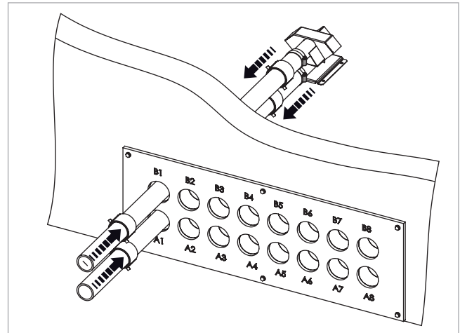
Abb. 80: Brandschutzmanschetten einschieben
