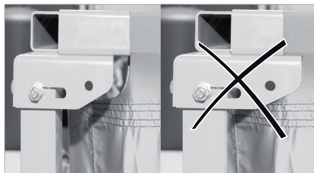
Abb. 100: Auf korrekten Sitz des Gewebes achten
