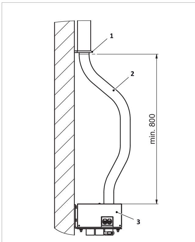
Abb. 43: Schlauchbefestigung Wand mit HT-Rohr
