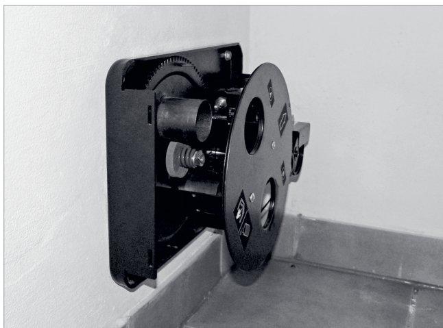
Abb. 24: Umschalteinheit montiert
