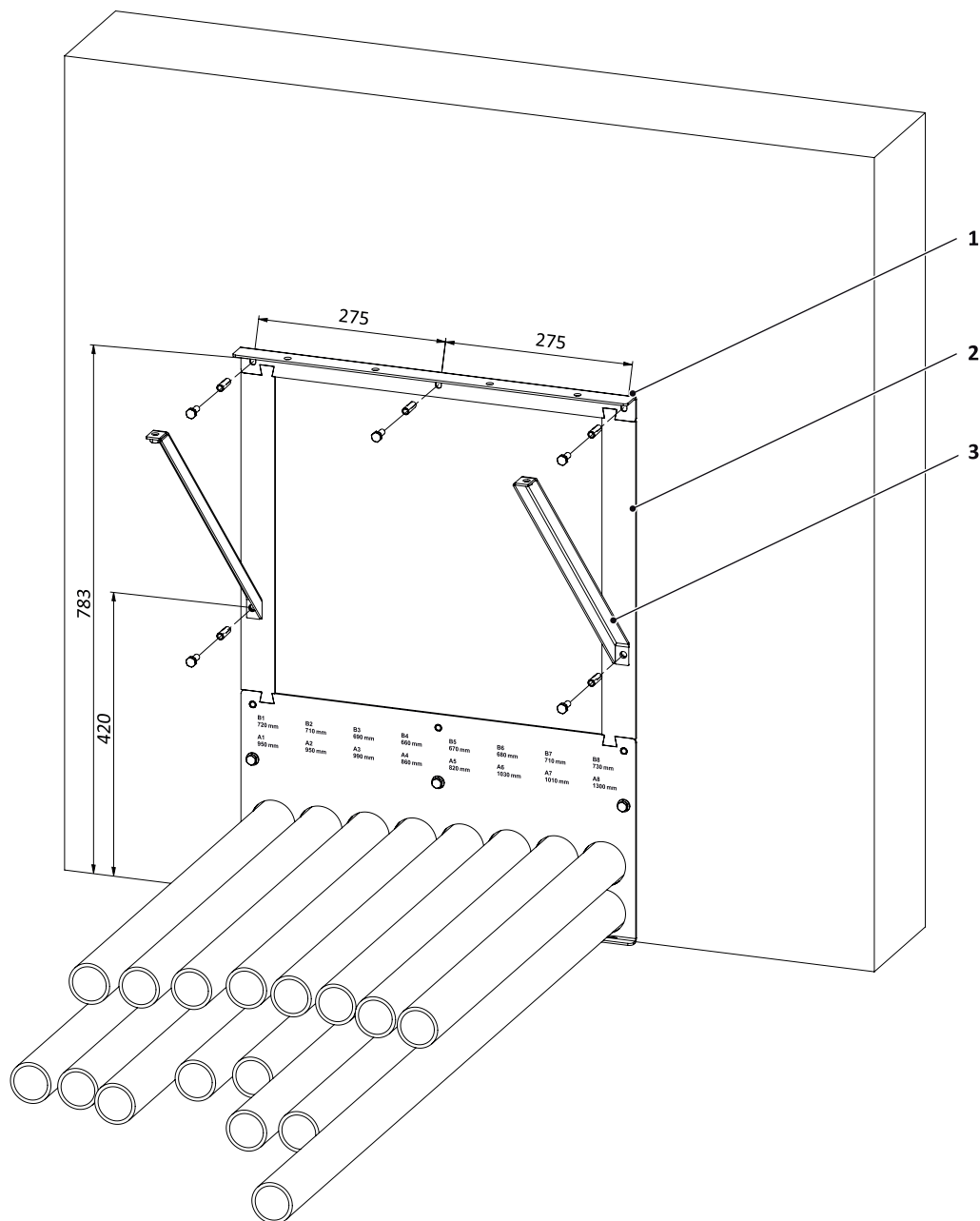
Abb. 62: Montagewinkel (1), Verbinder (2) und Abstützwinkel (3) montieren
