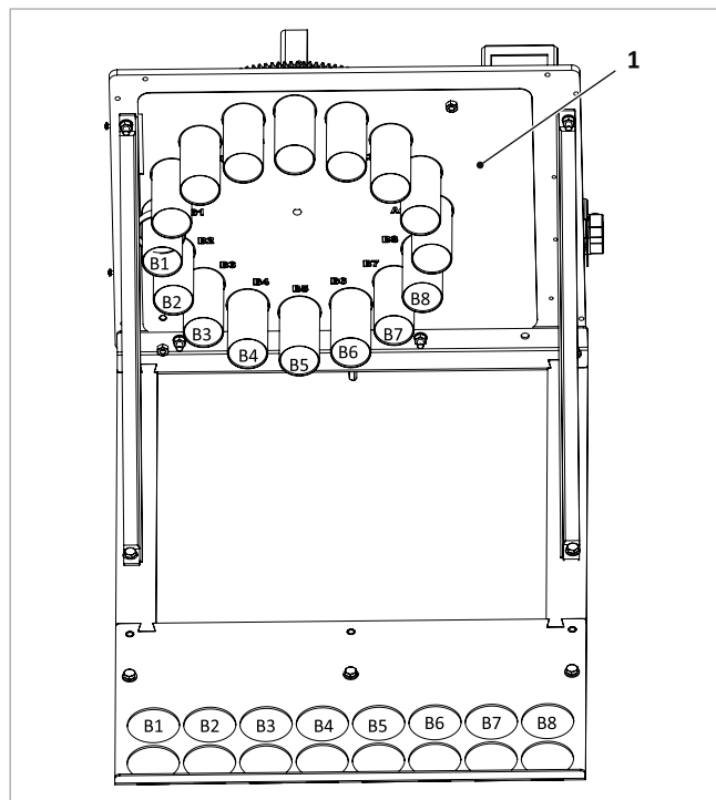
Abb. 65: Rückluftschläuche B1 bis B8 auf Umschalteteinheit montieren
