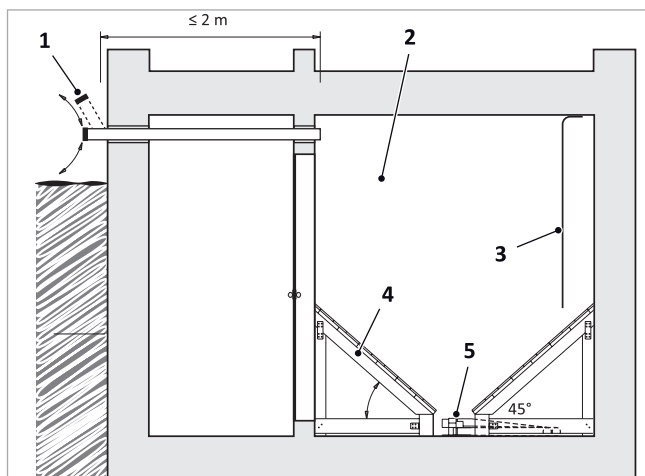
Abb. 4: Pelletlager bis zu 2 m Lüftungsdistanz
