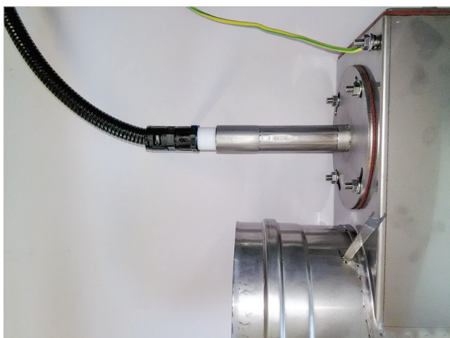
Abb. 5: Hochspannungskabel am Isolator montiert
