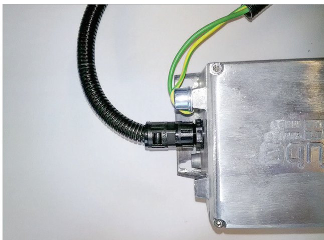
Abb. 7: Hochspannungskabel an Steuerungsbox montiert
