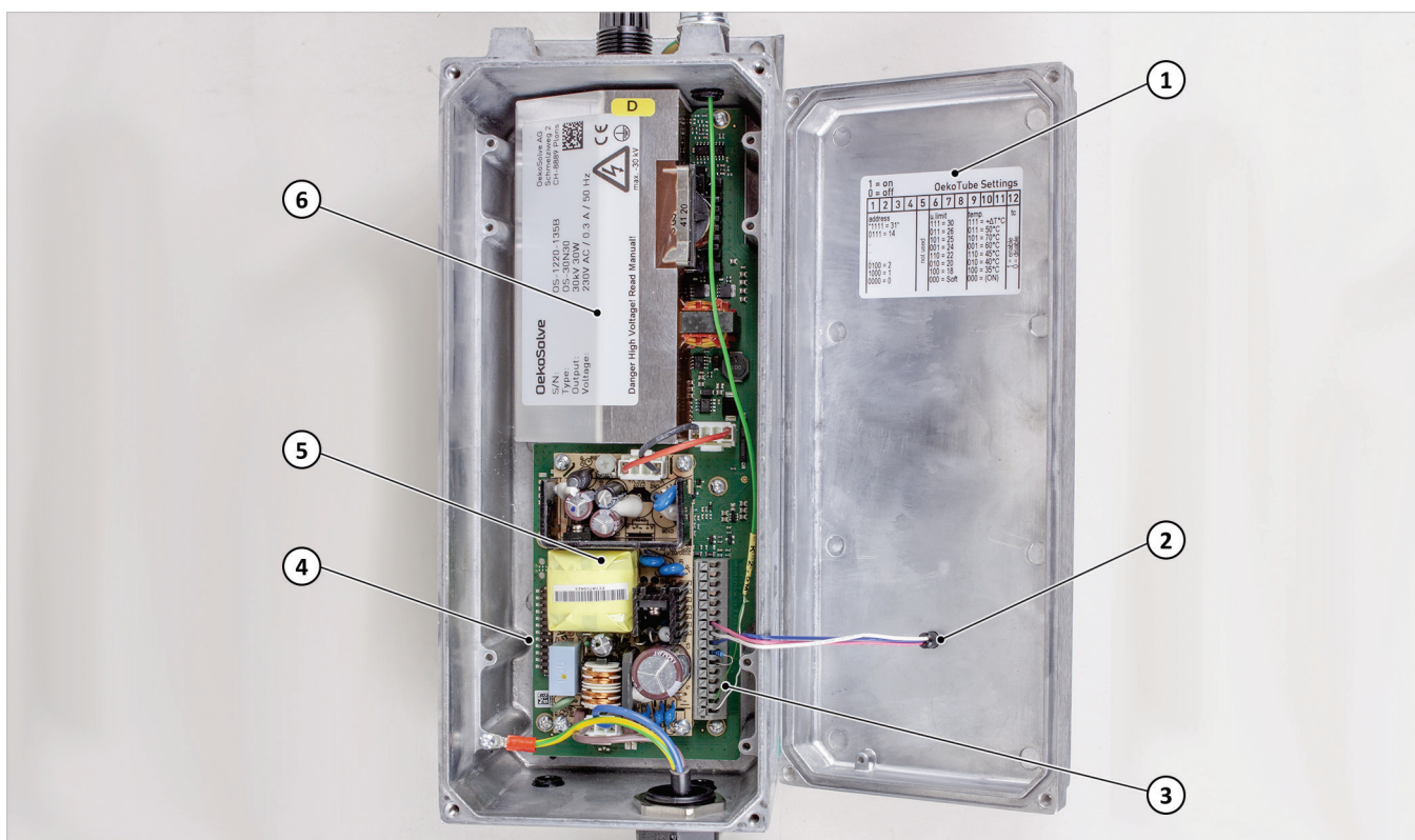
Abb. 19: Steuerungsplatine Feinstaubfilter
