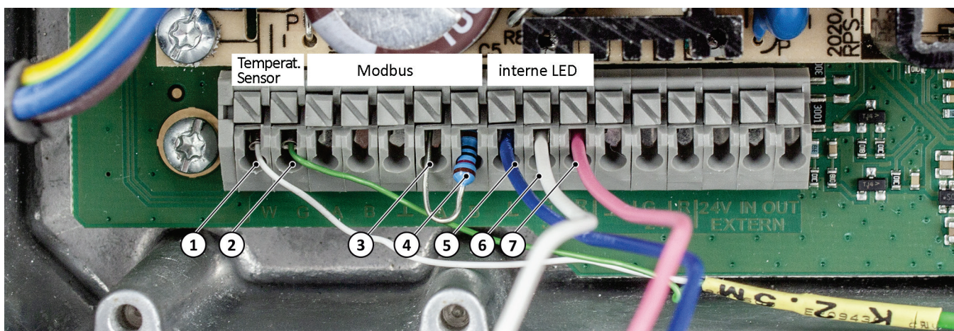
Abb. 20: Klemmenblock Feinstaubfilter
