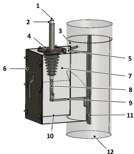
Abb. 3: Komponentenübersicht des Abscheiders des Feinstaubfilters
